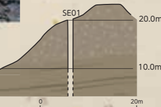
井戸の断面図
