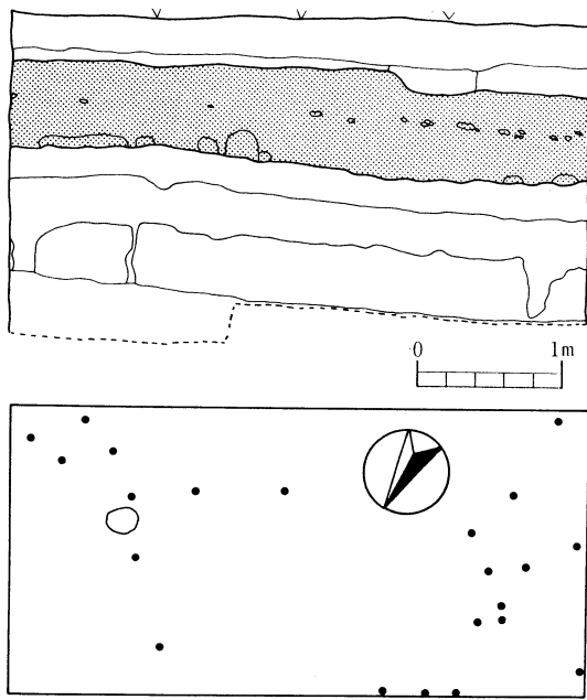
第9図 第3地点8 Tの層位断面図
