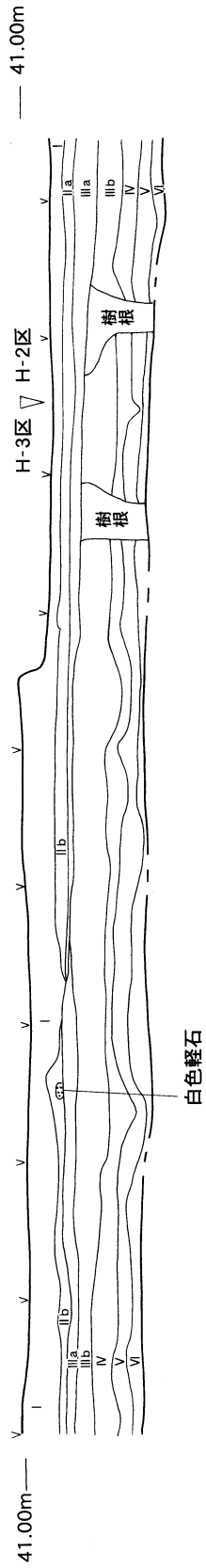
H-2~4区 東側土層断面図 ③
