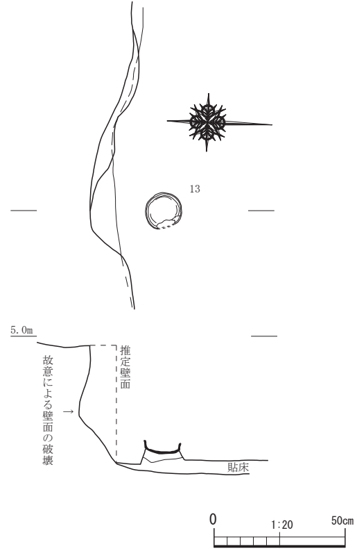
第11図 竪穴建物11南壁遺物出土状況図
