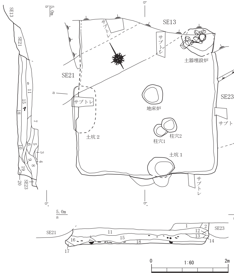
第16図 堅穴建物22地床炉実測図
