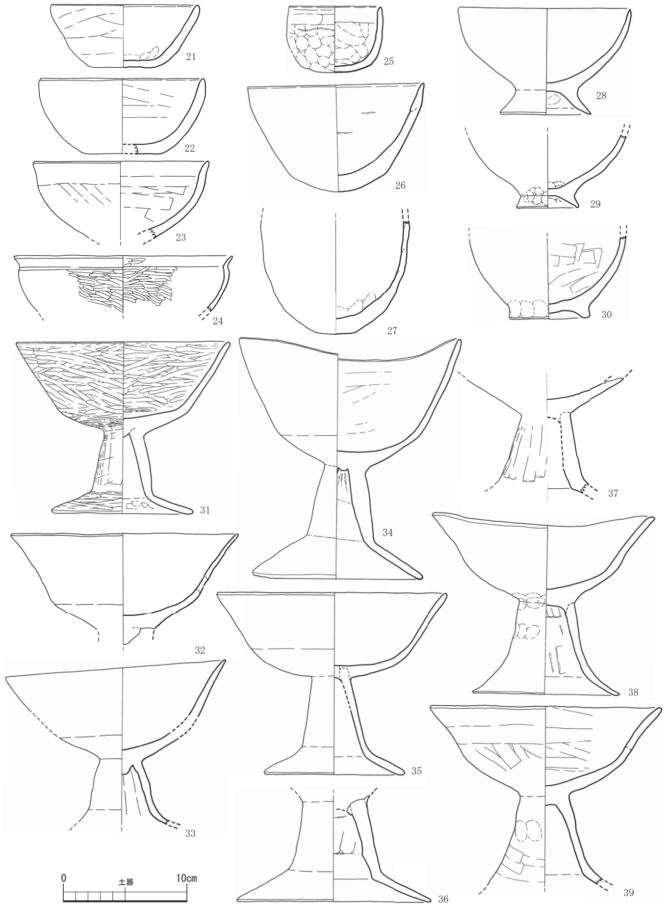
第19図 堅穴建物22出土遺物実測図①
