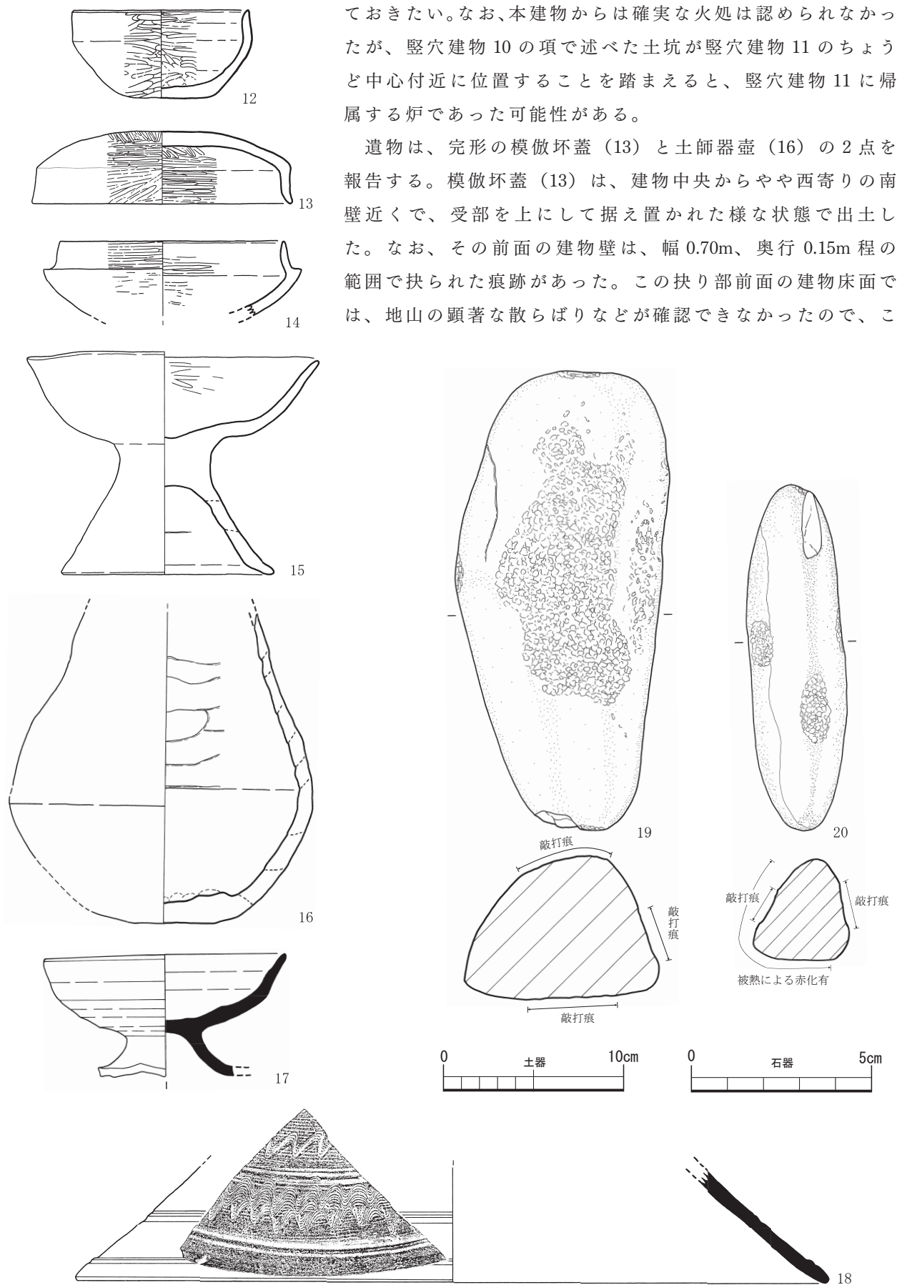
第 14 図 竪穴建物 10、11 出土遺物実測図
