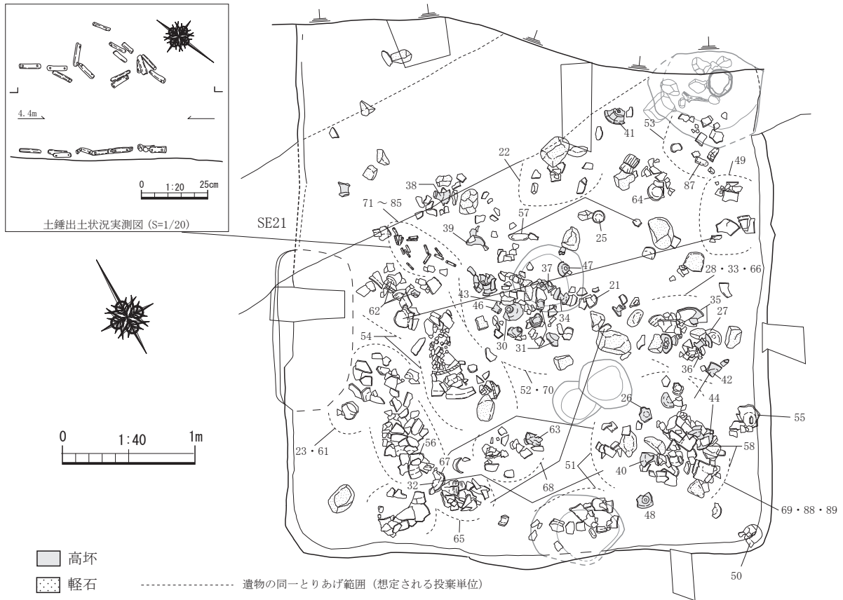
第 18 図 竪穴建物 22 遺物出土状況図 (S=1/40)
