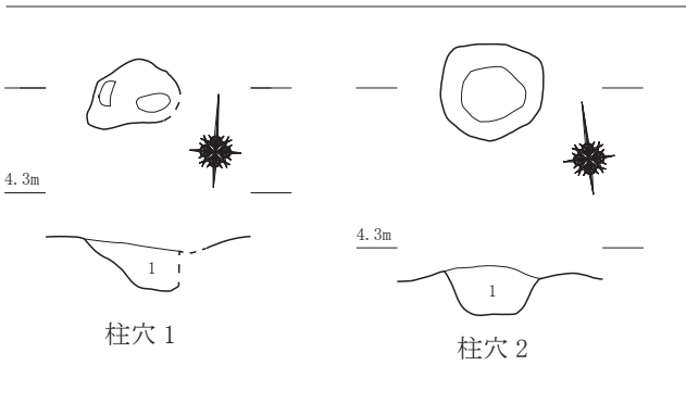
第7図 堅穴建物 10、11 実測図②(S=1/60)
