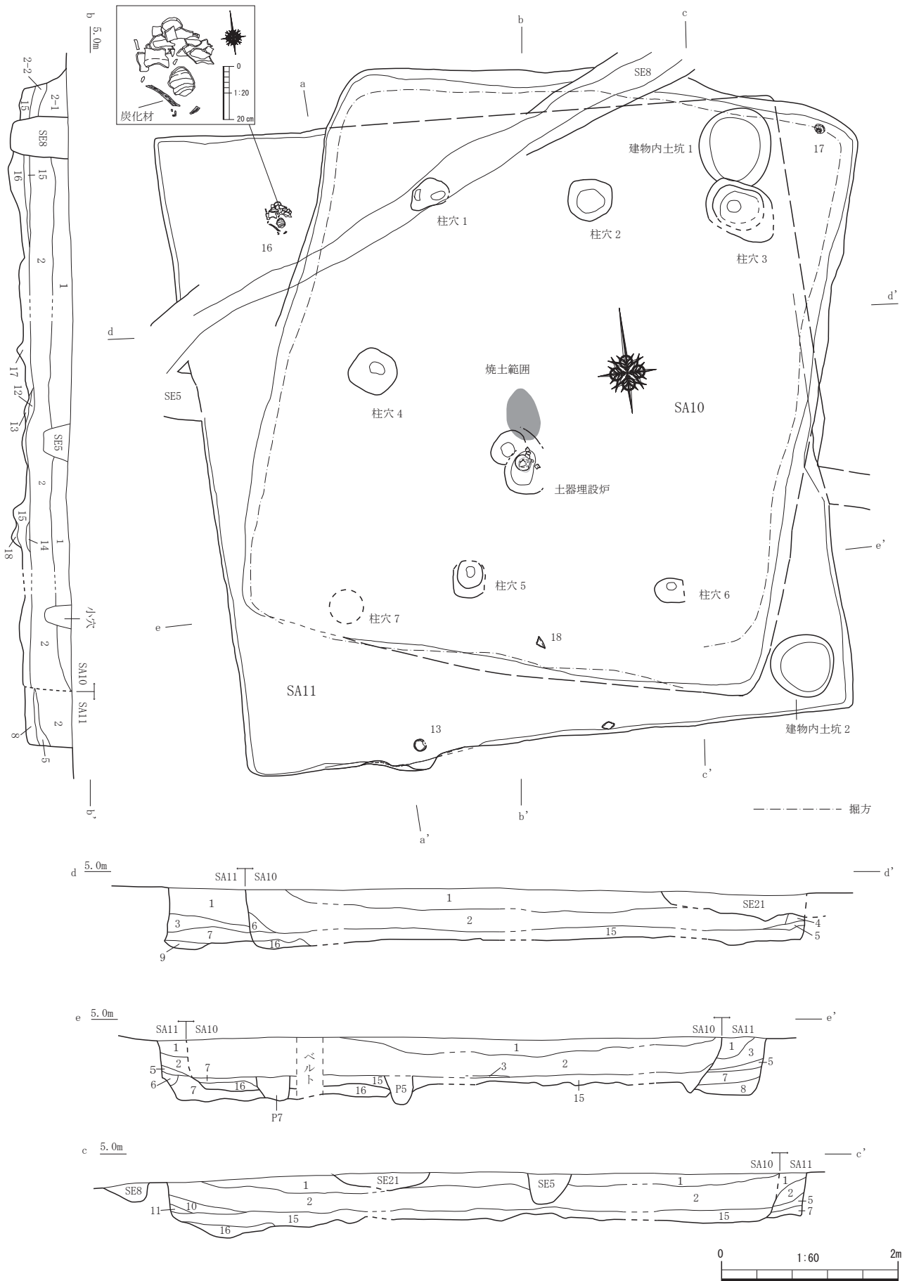
第 6 図 竪穴建物 10、11 実測図①(S=1/60)
