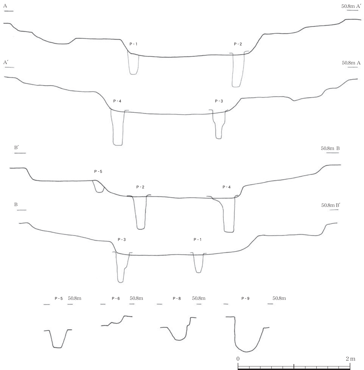
第105図 2号竖穴住居跡断面図
