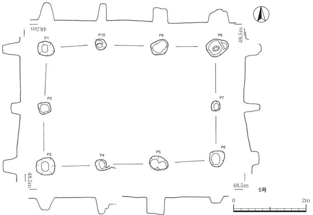
第138图 掘立柱建物跡4・5号
