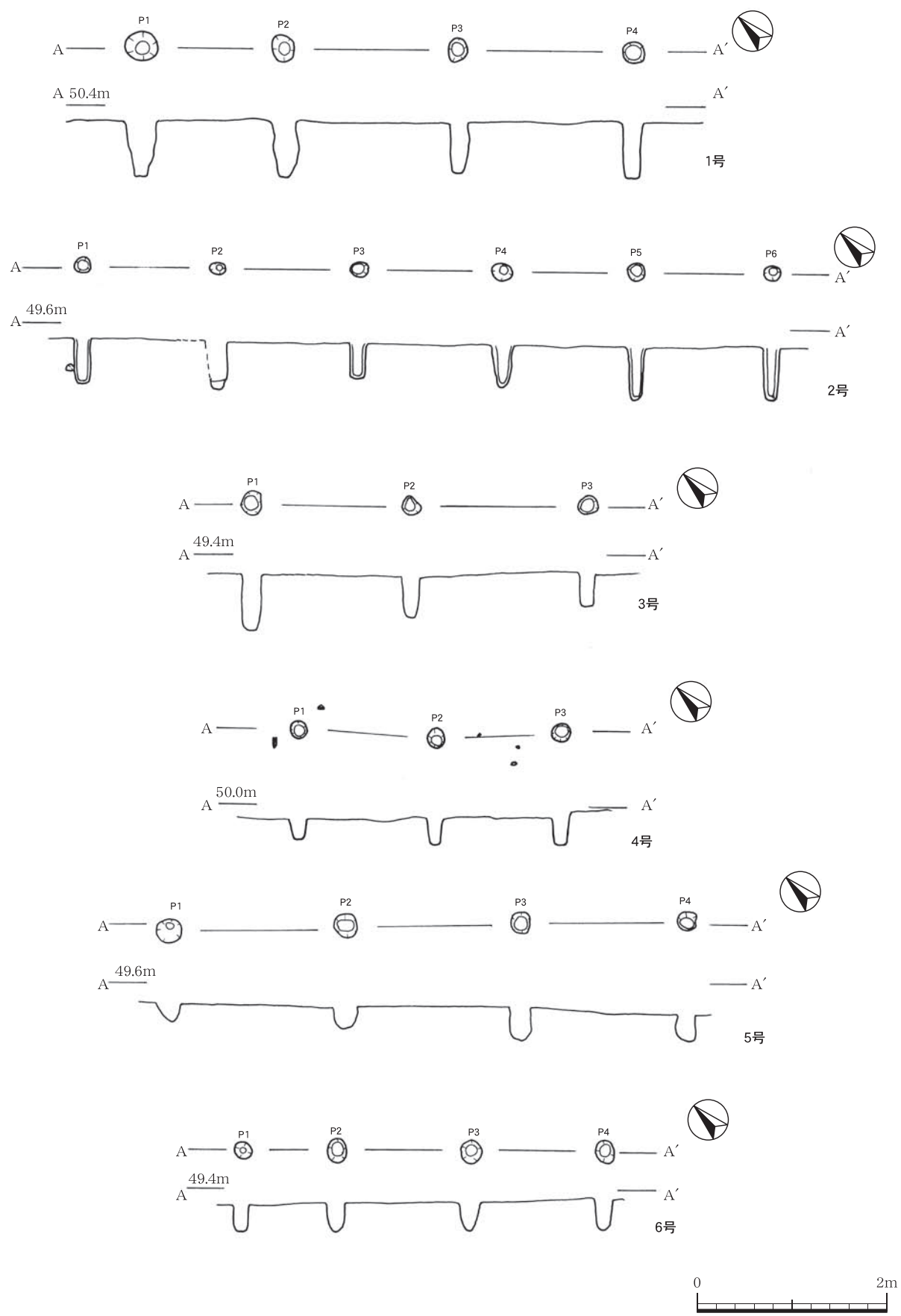
第94图 柱穴列 1~6号
