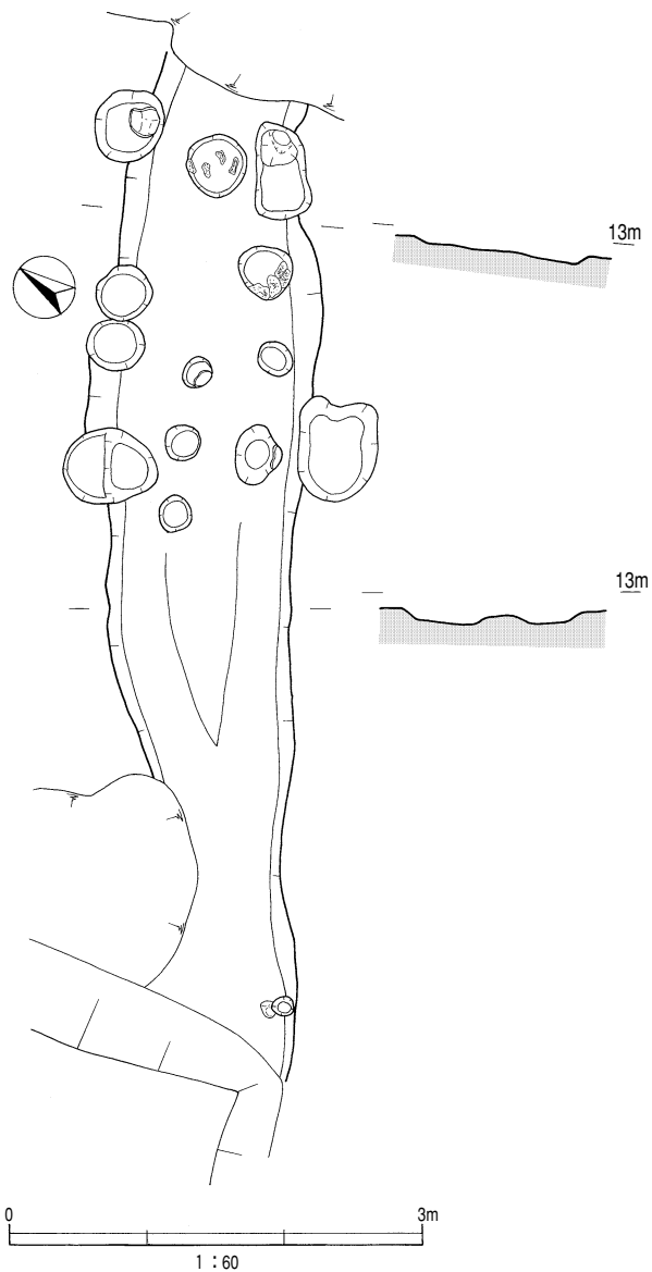
第21図 溝状遺構
