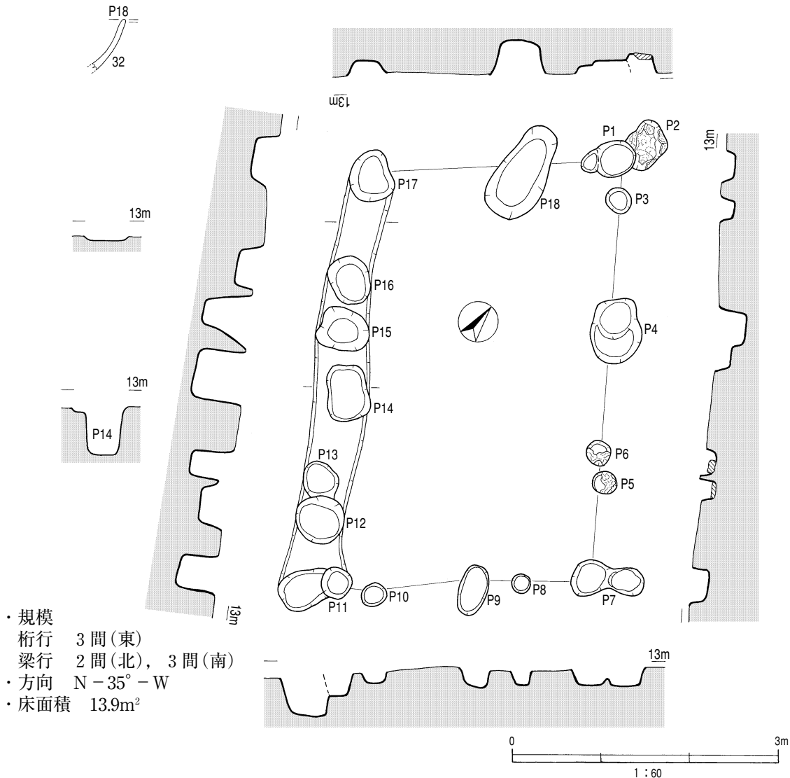
第12図 掘立柱建物跡1号
