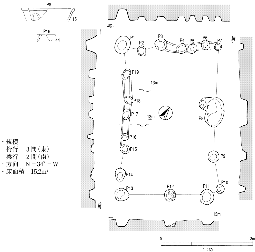
第13図 掘立柱建物跡2号
