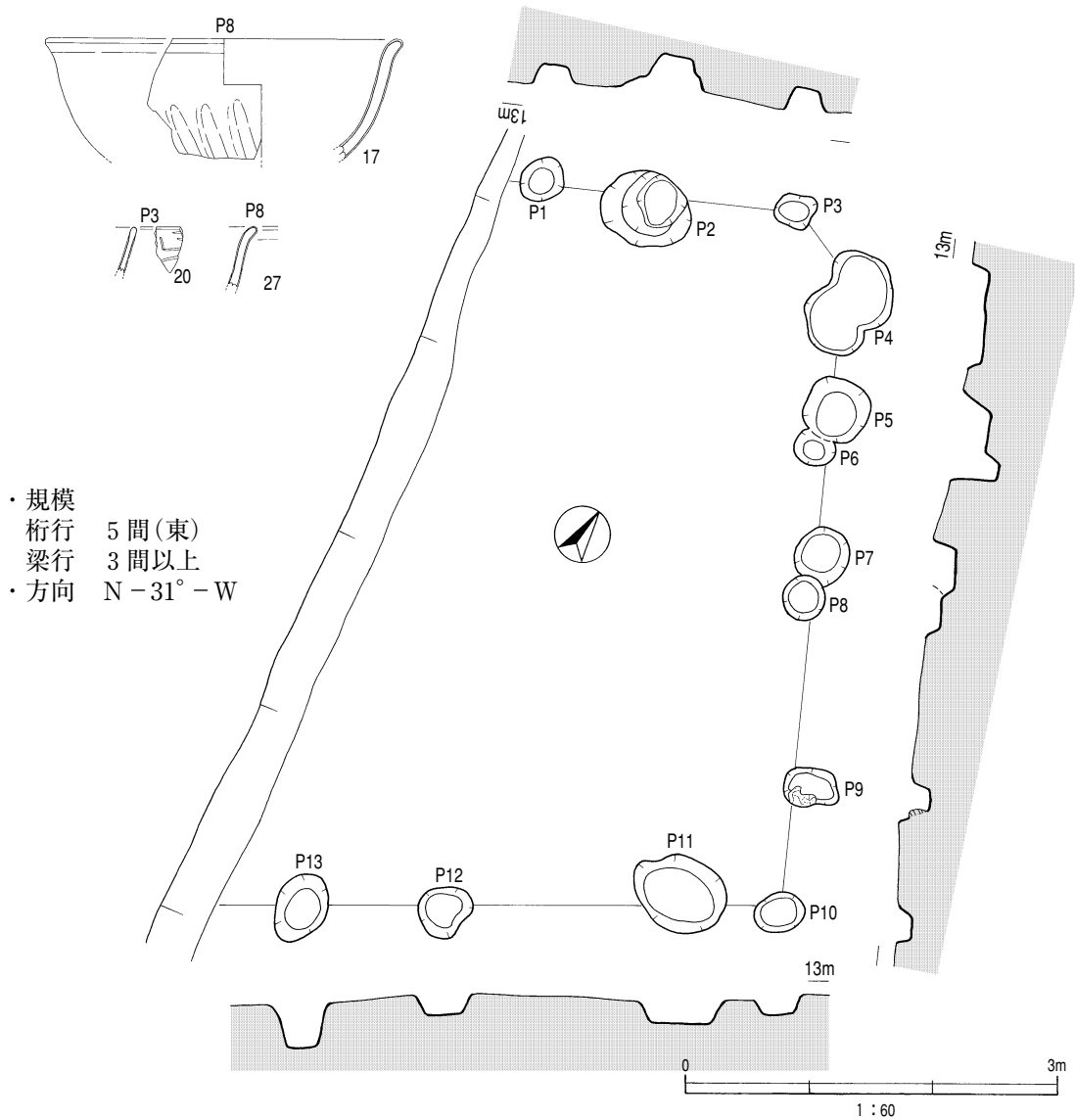
第17図 掘立柱建物跡5号
