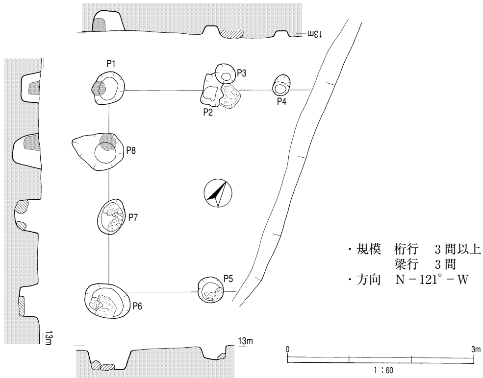
第16図 掘立柱建物跡4号
