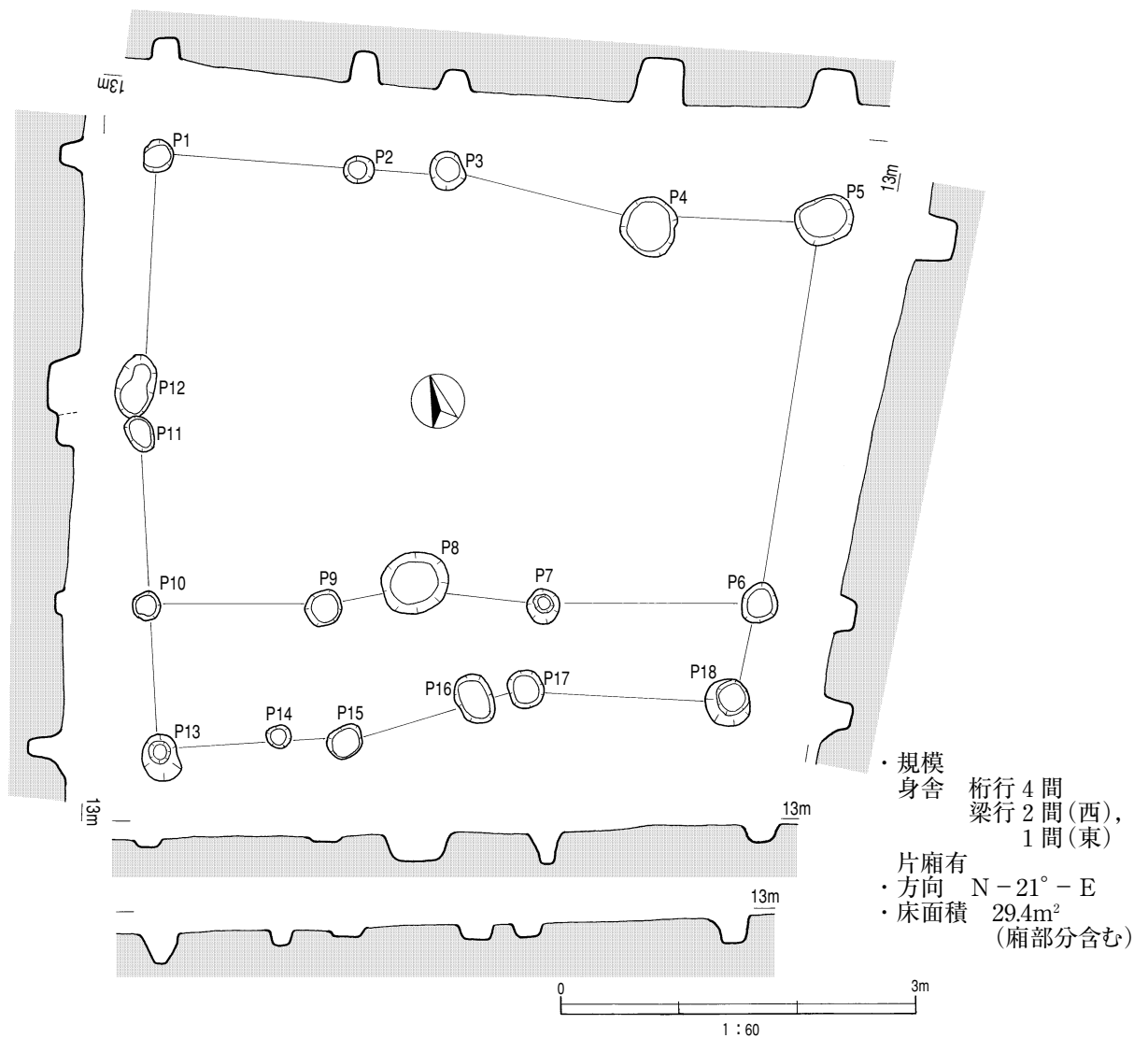
第20図 掘立柱建物跡 9号
