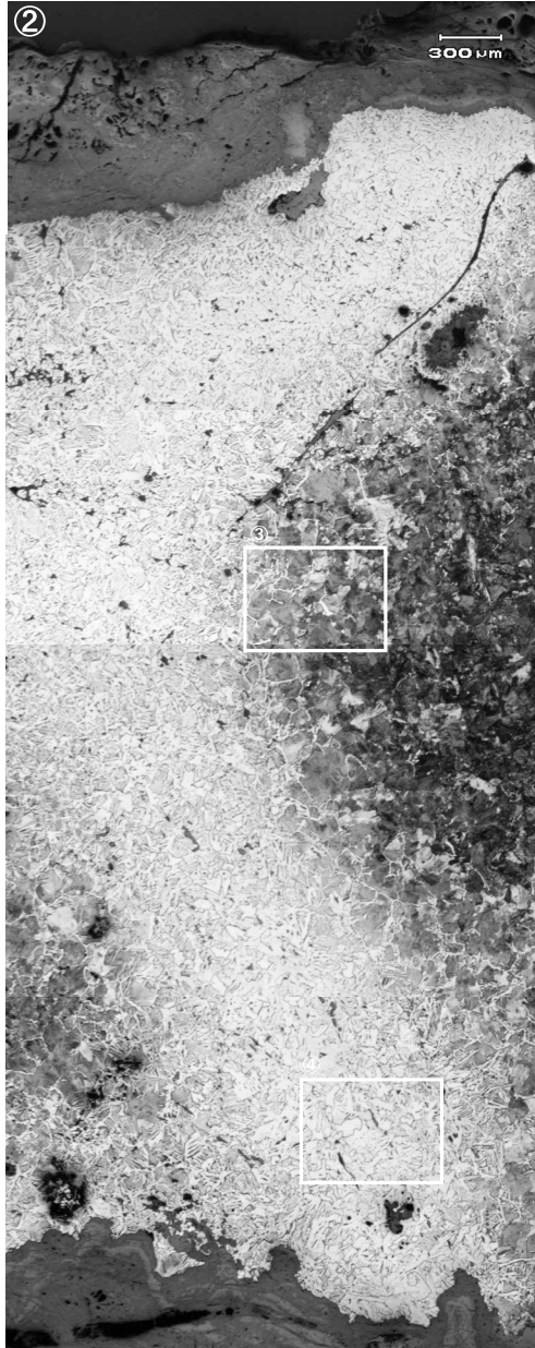
Photo.2 鉄釘の顕微鏡組織
