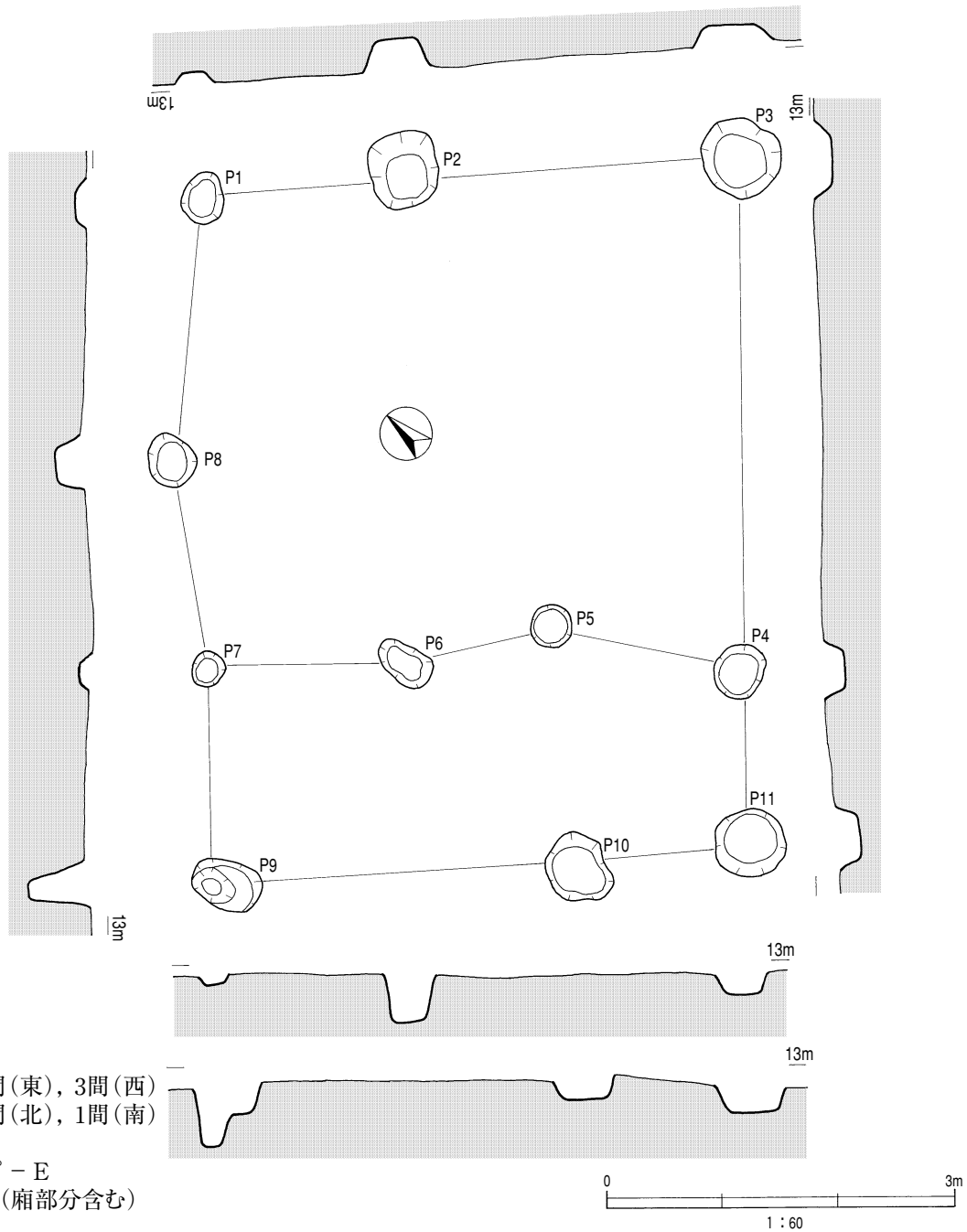
第19図 掘立柱建物跡 8号
