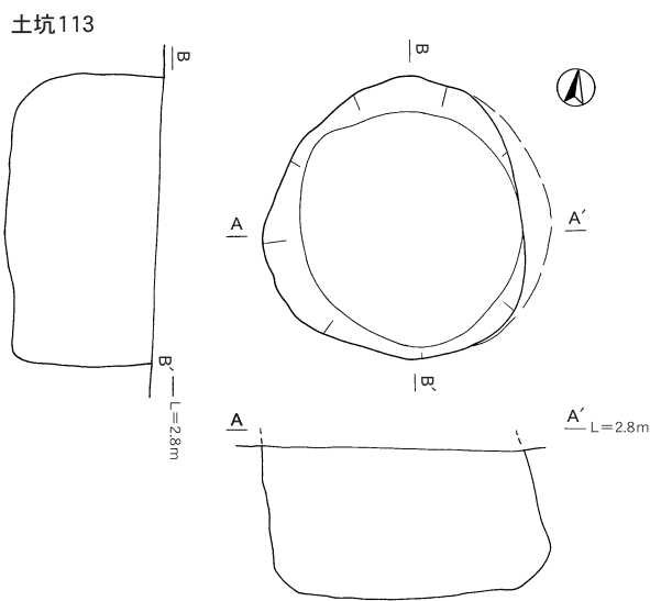
第144図 土坑⑥
