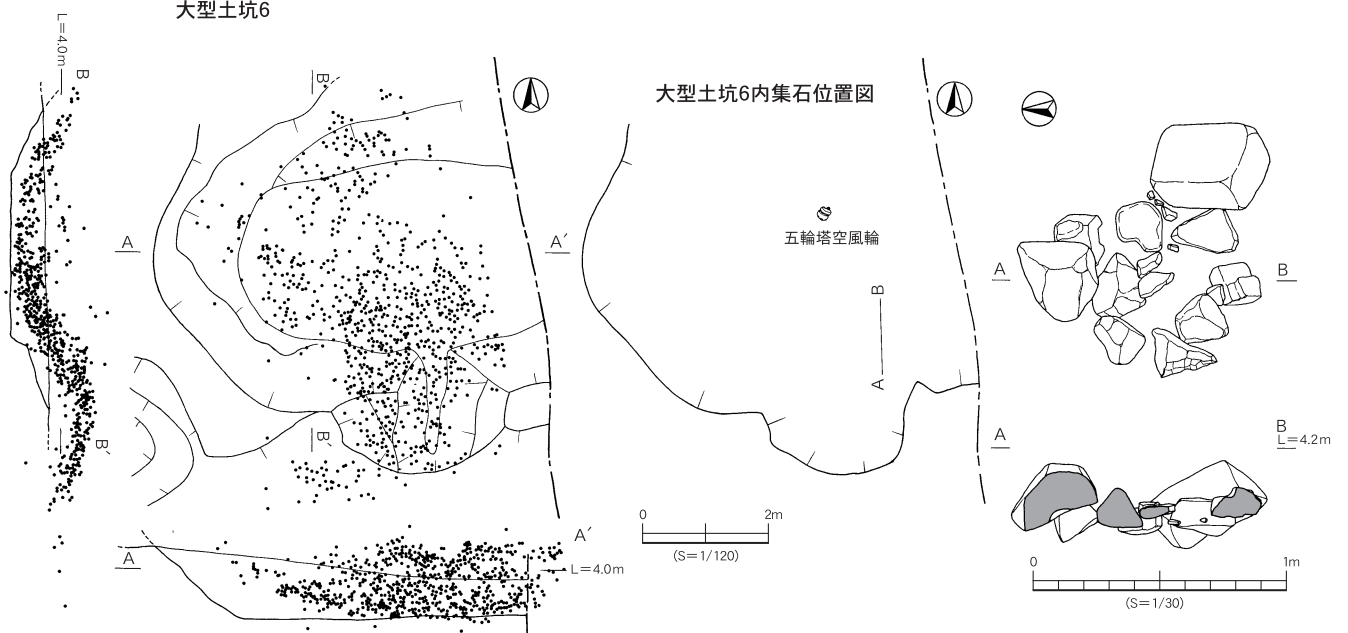
第134図 大型土坑④
