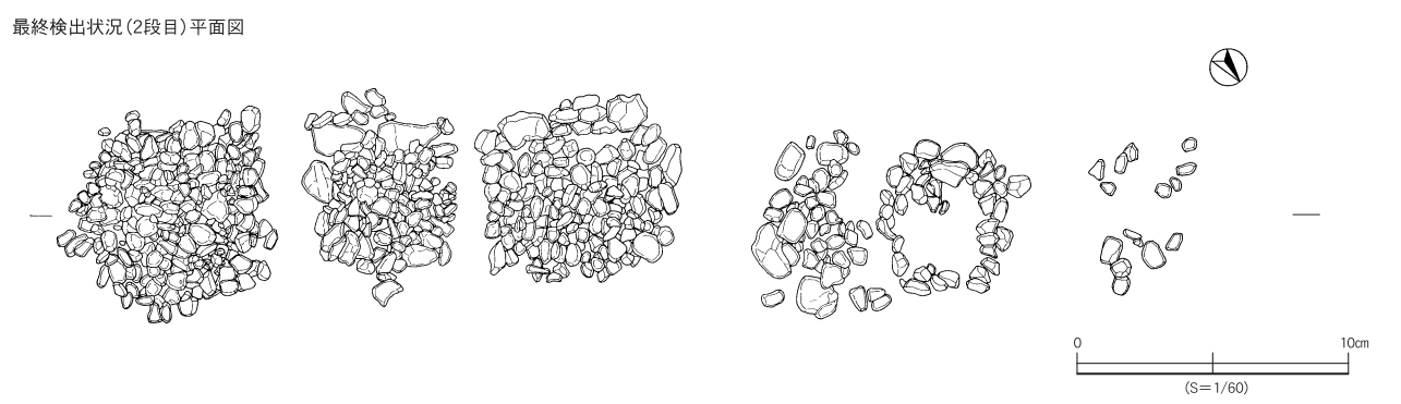
第189図 礫積遺構
