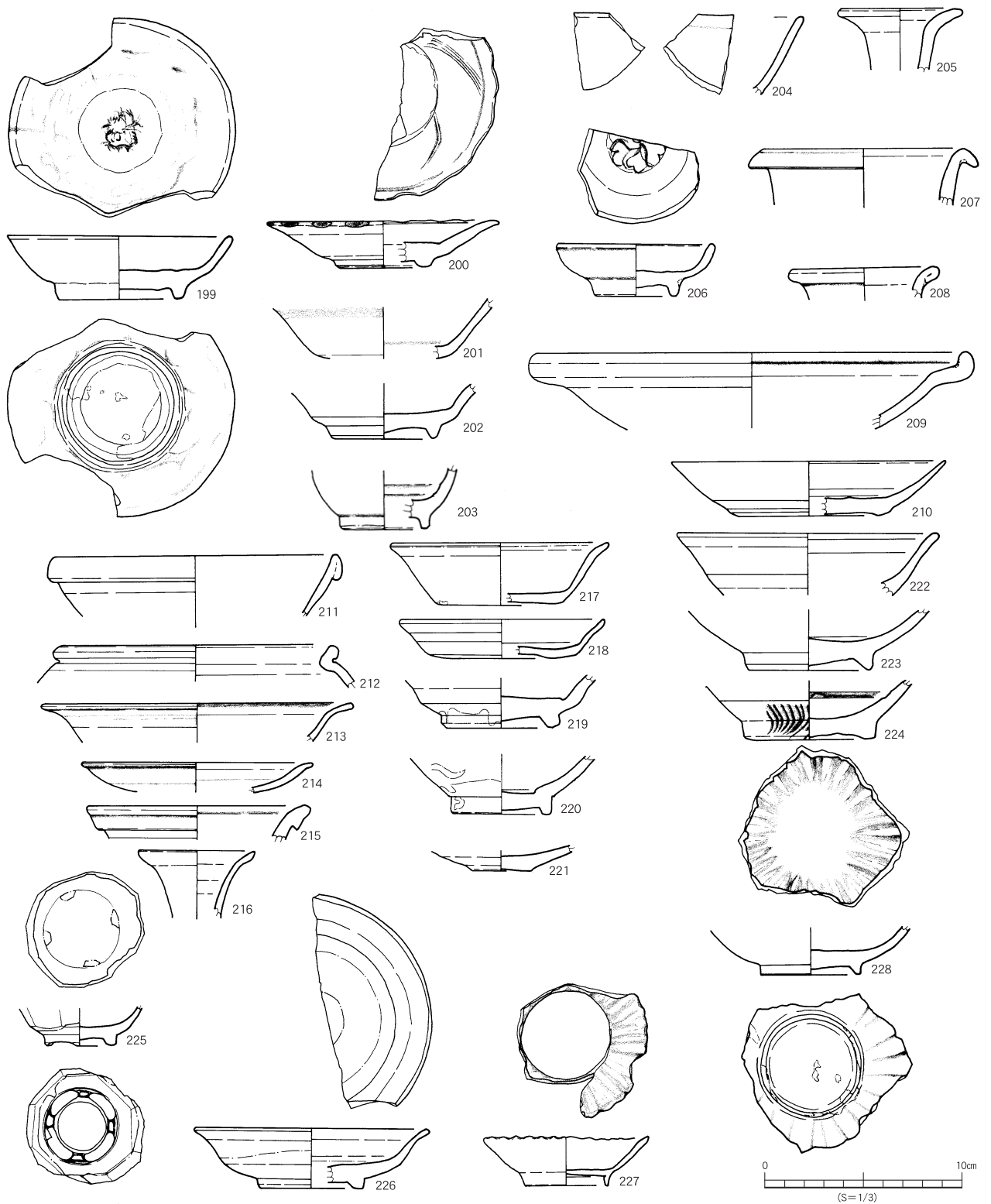
第168図 大溝出土遺物実測図⑯
