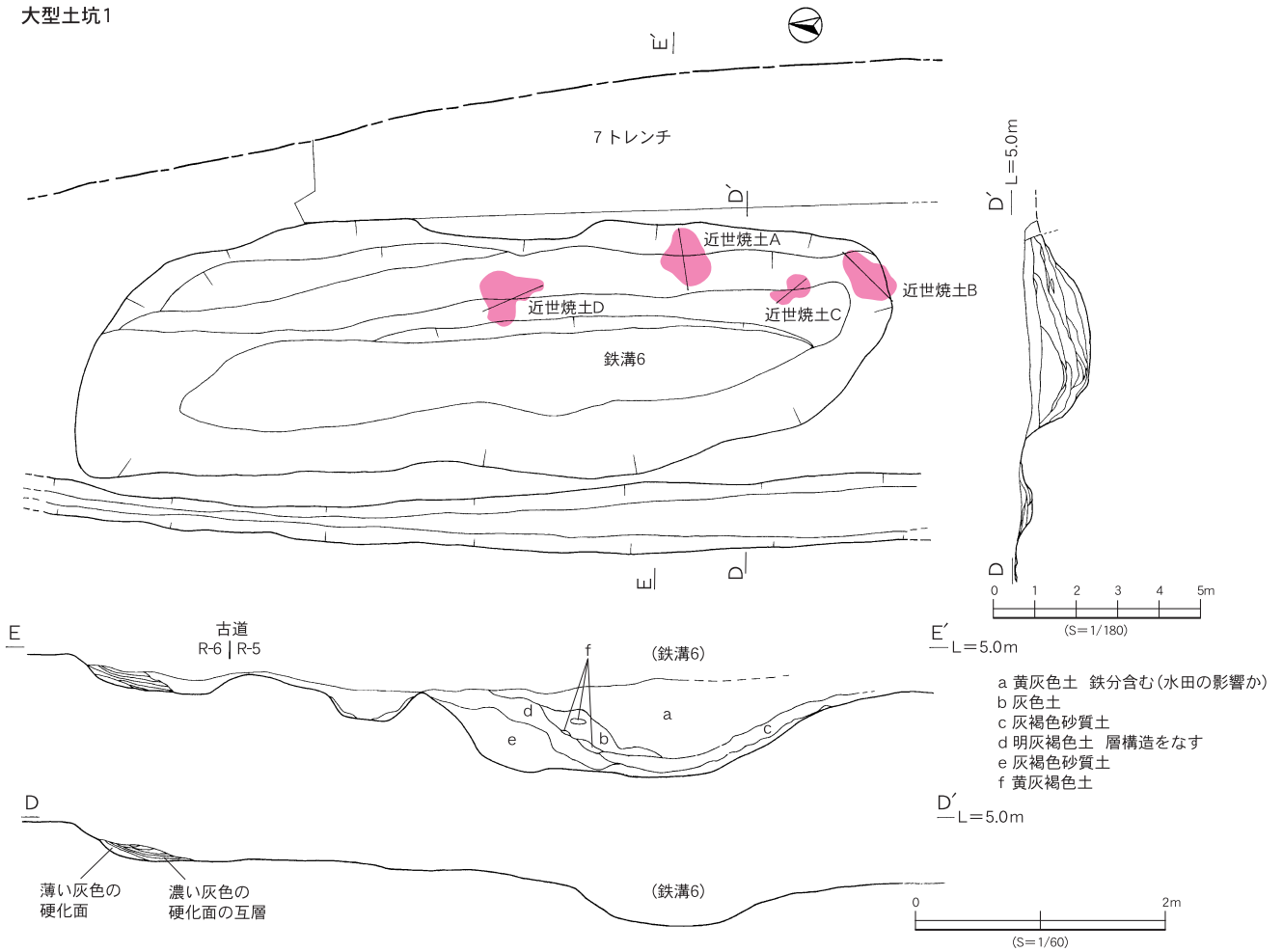
第124図 大型土坑①
