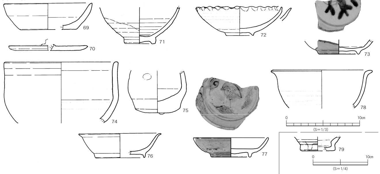
第128図 大型土坑出土遺物実測図③
