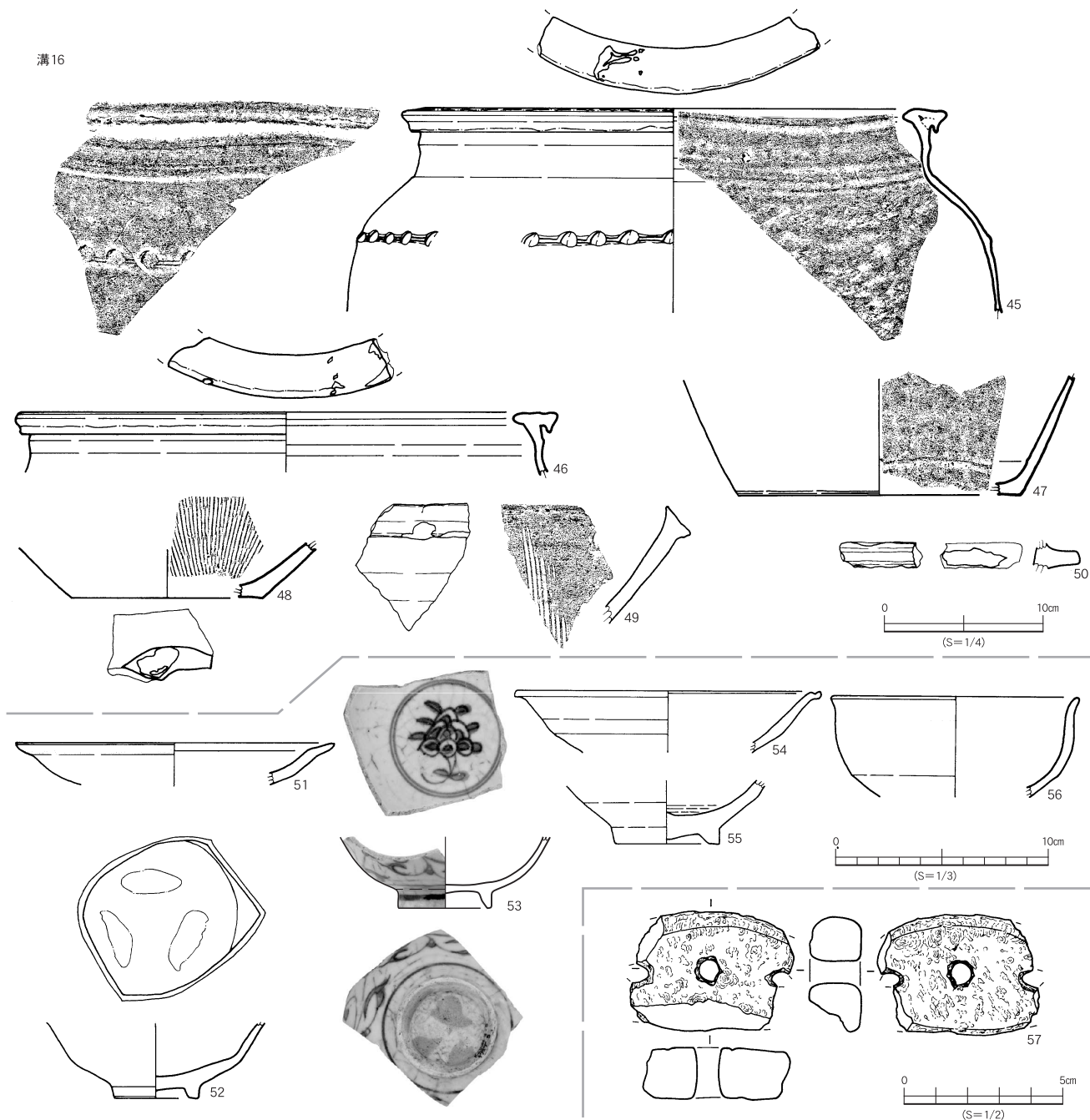
第180図 溝内出土遺物実測図④
