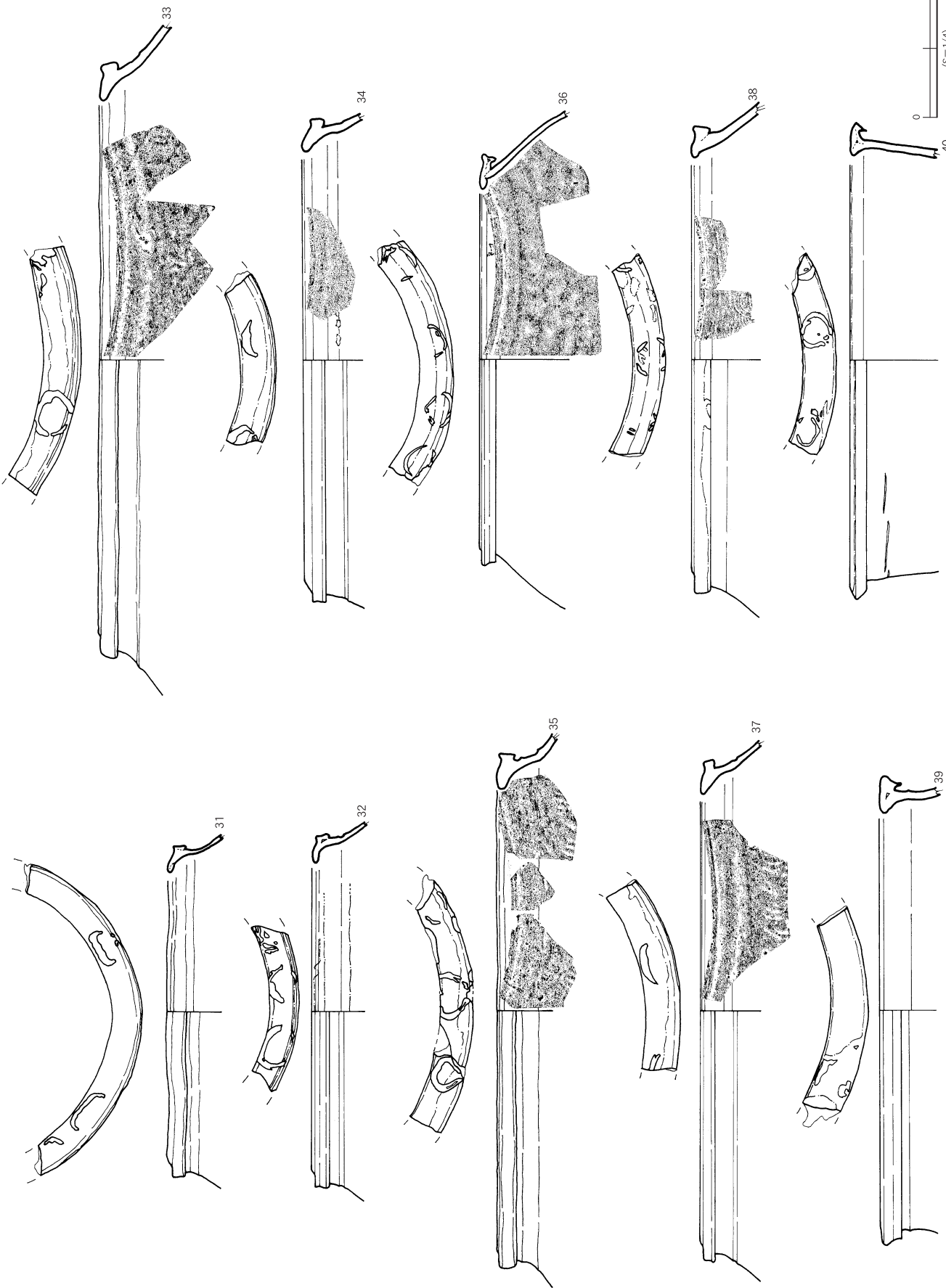
第155図 大溝出土遺物実測図③
