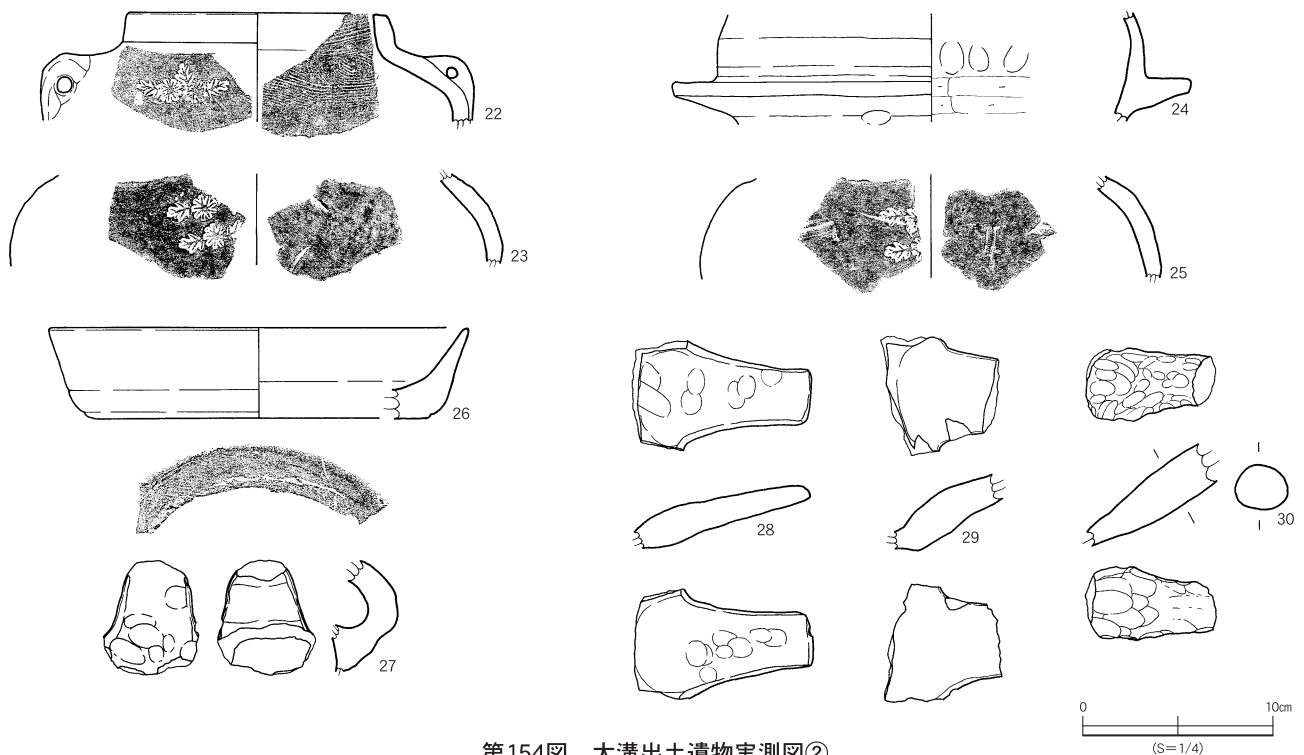
第154図 大溝出土遺物実測図②
