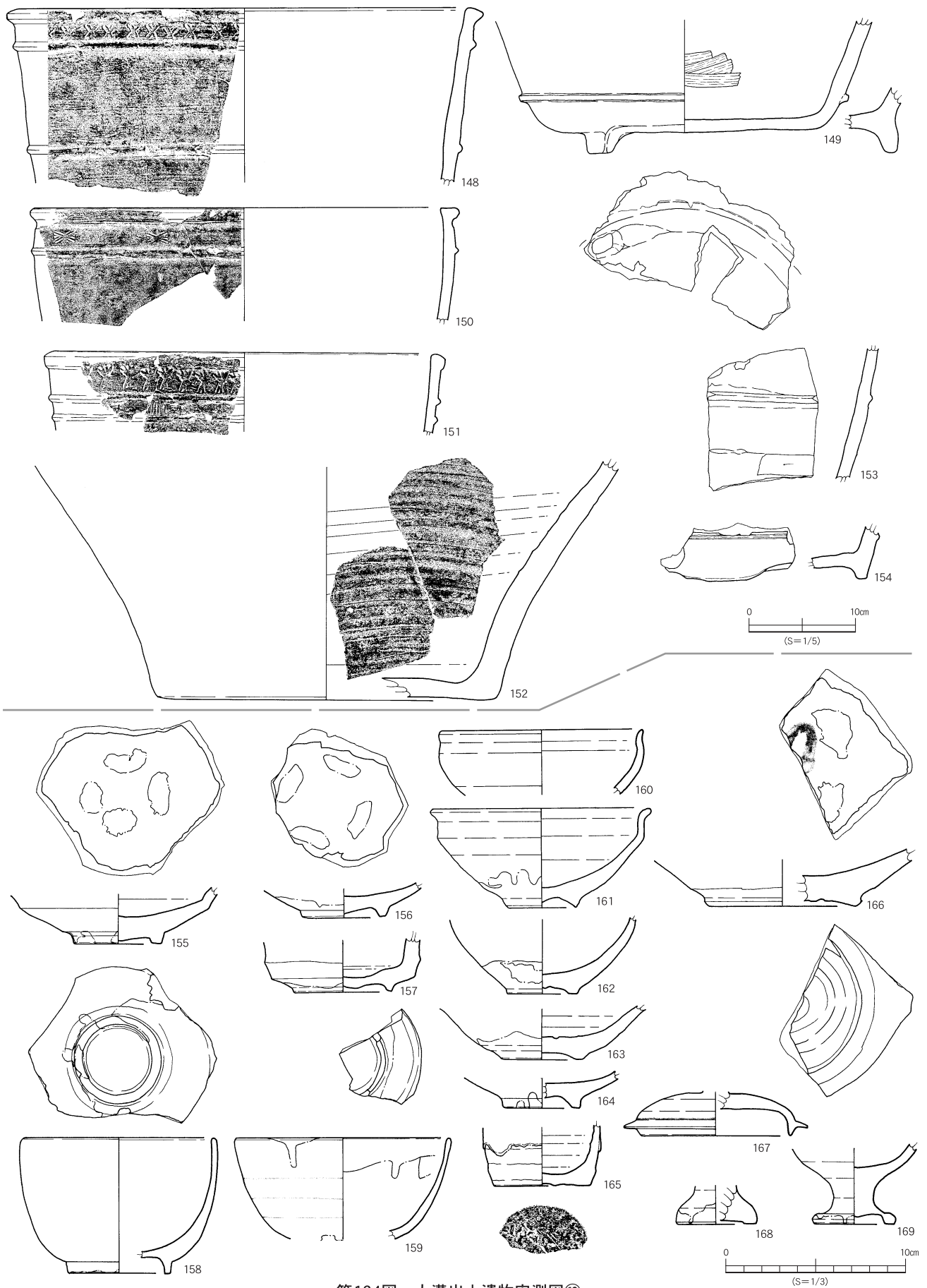
第164図 大溝出土遺物実測図⑫
