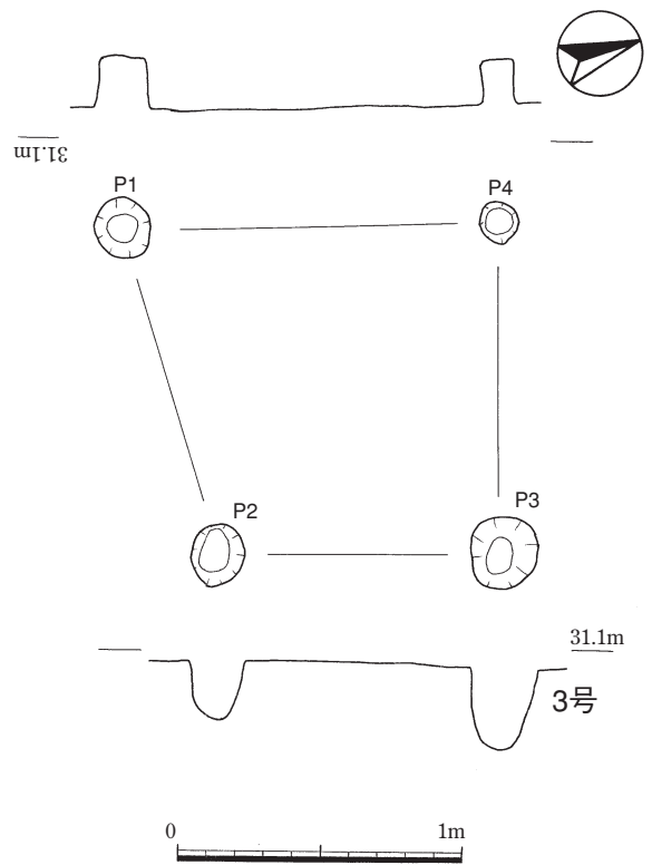
第34図 縄文時代晩期掘立柱建物跡
