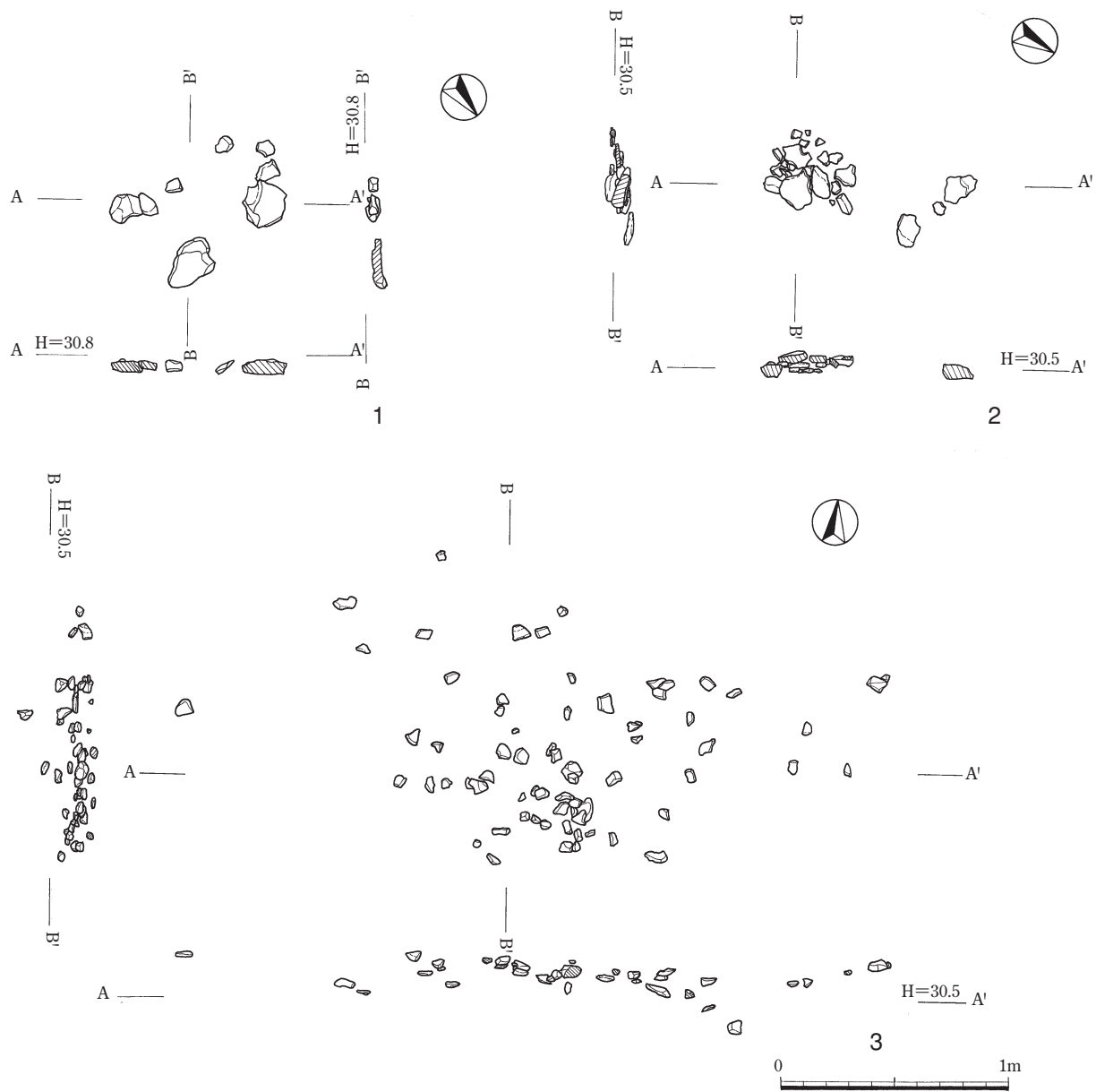
第21図 縄文時代草創期集石遺構 1
