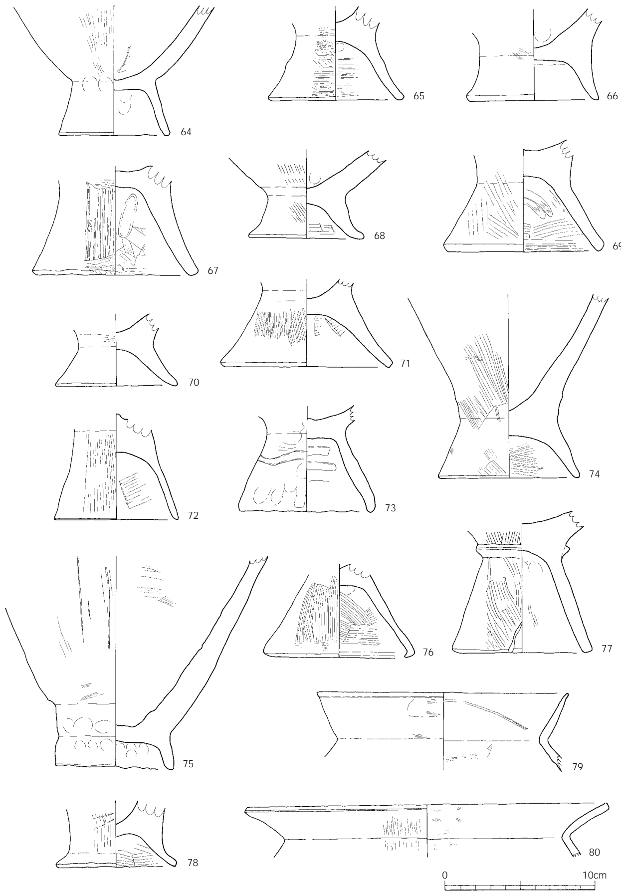
第66図 古墳時代甕形土器 (10)
