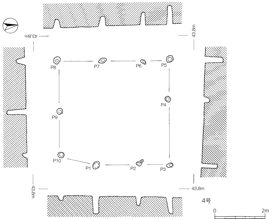
第81图 掘立柱建物跡 3, 4号
