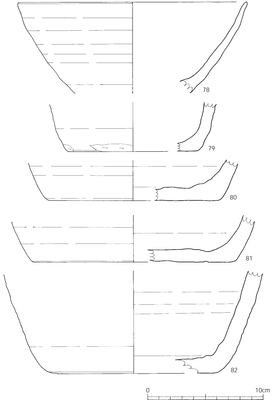
第104図 古代土師器（6）鉢
