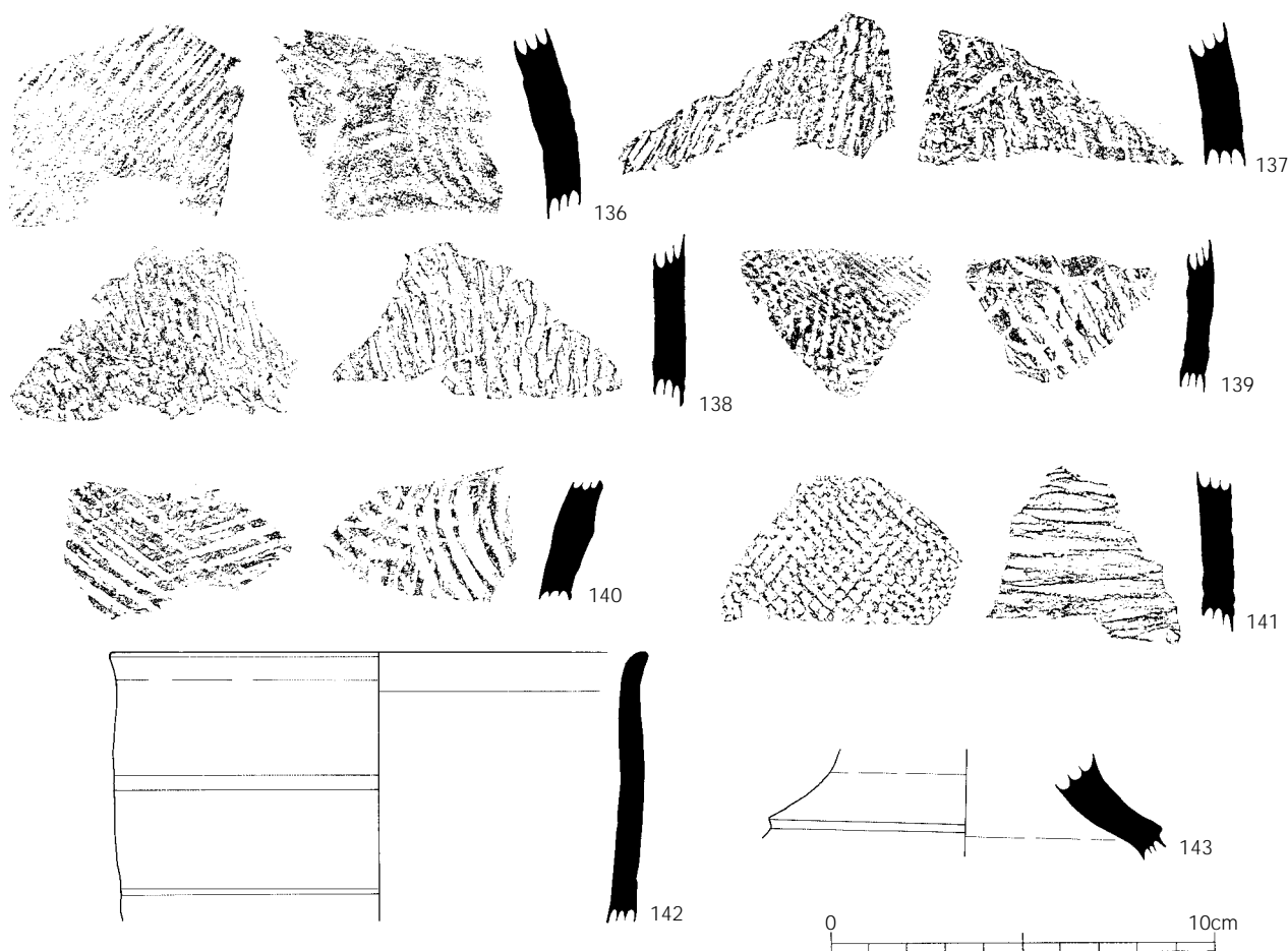
第111図 古代須恵器(3) 甕, 鉢, 壺
