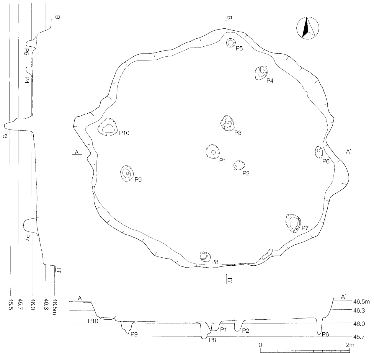
第2図 弥生時代1号住居跡
