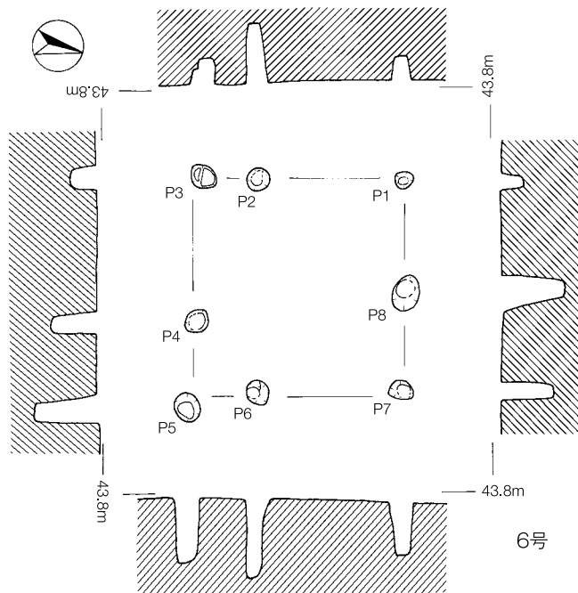
第82図 掘立柱建物跡 5, 6号
