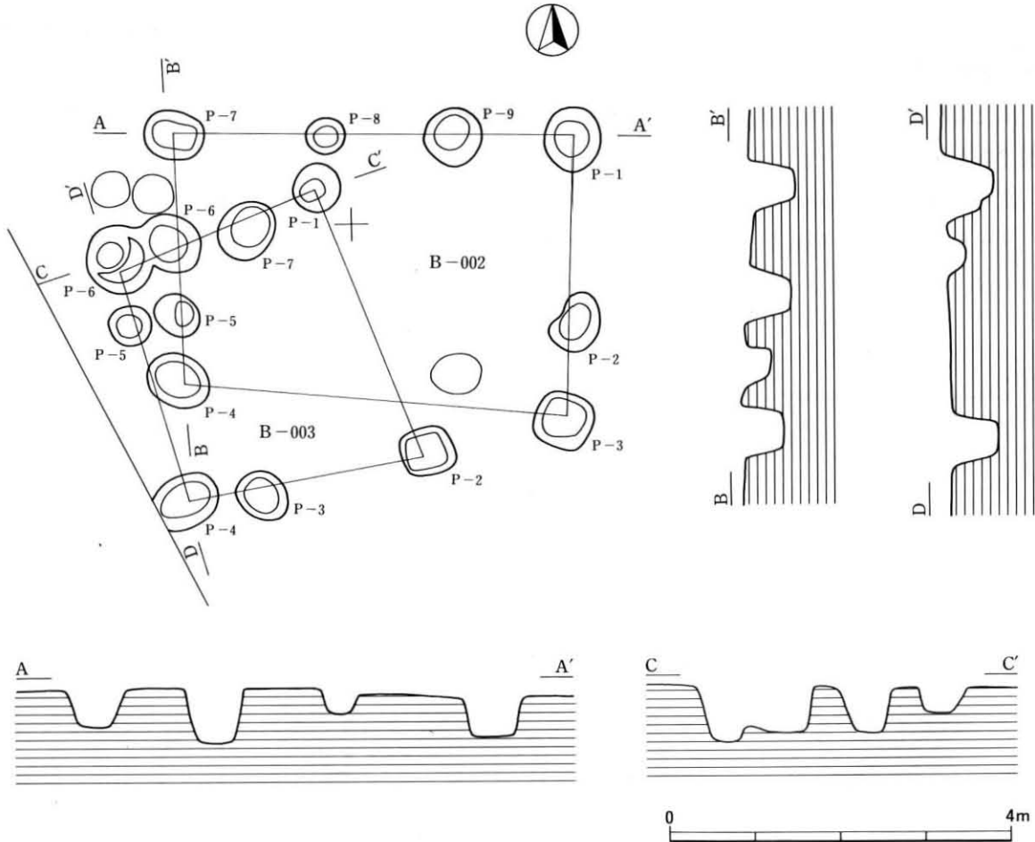
第10図 B-002号・003号実測図
