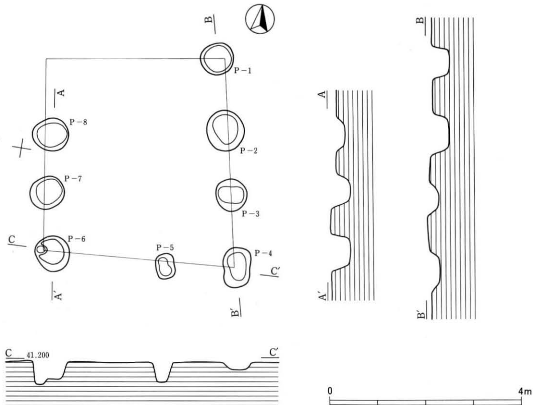
第9図 B-001号実測図
