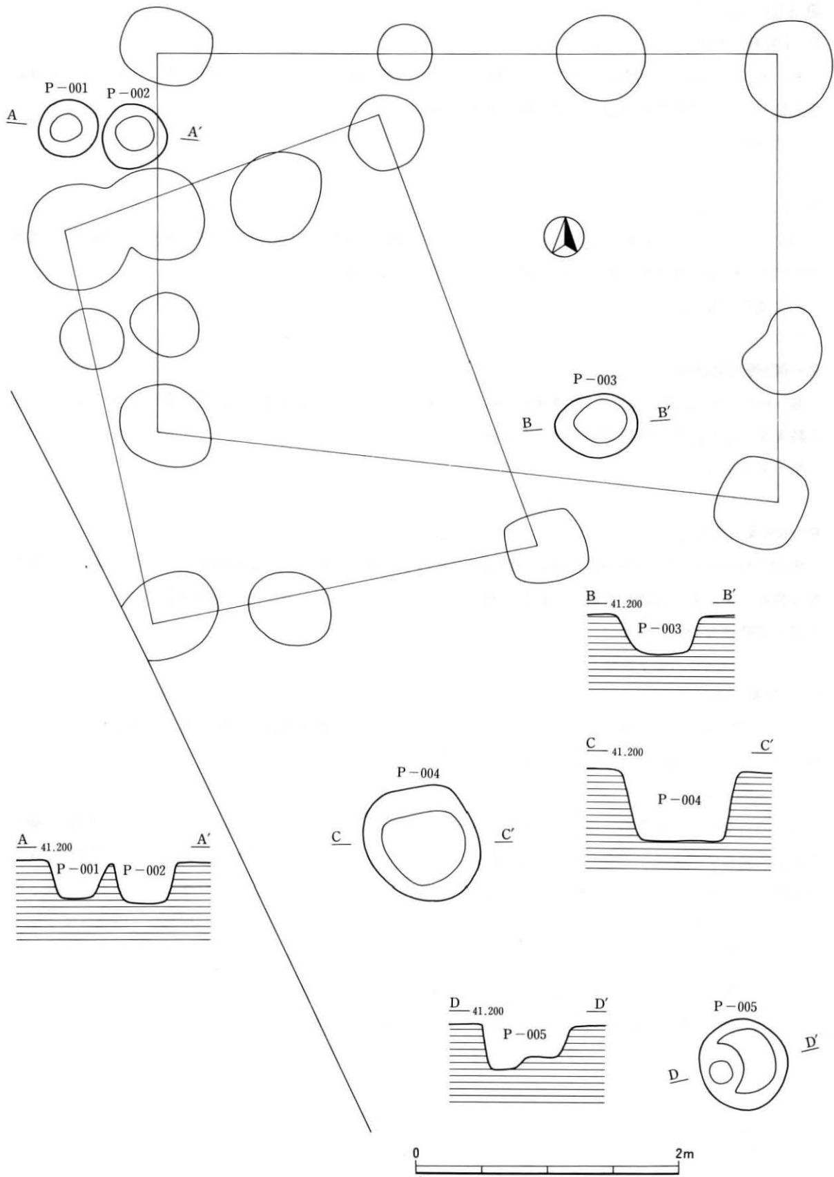
第11図 P-001号~P-005号実測図
