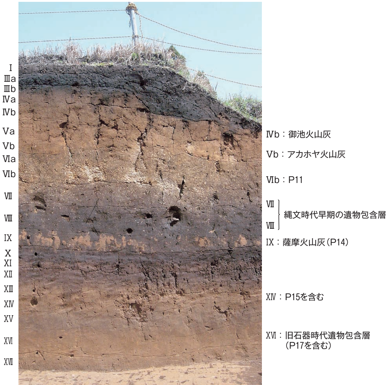
土層断面
