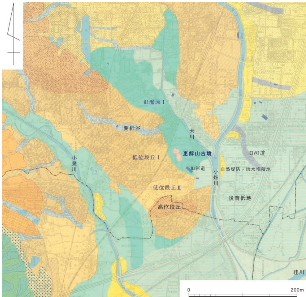
第2図 恵解山古墳周辺の地形条件図 (1/20000)
