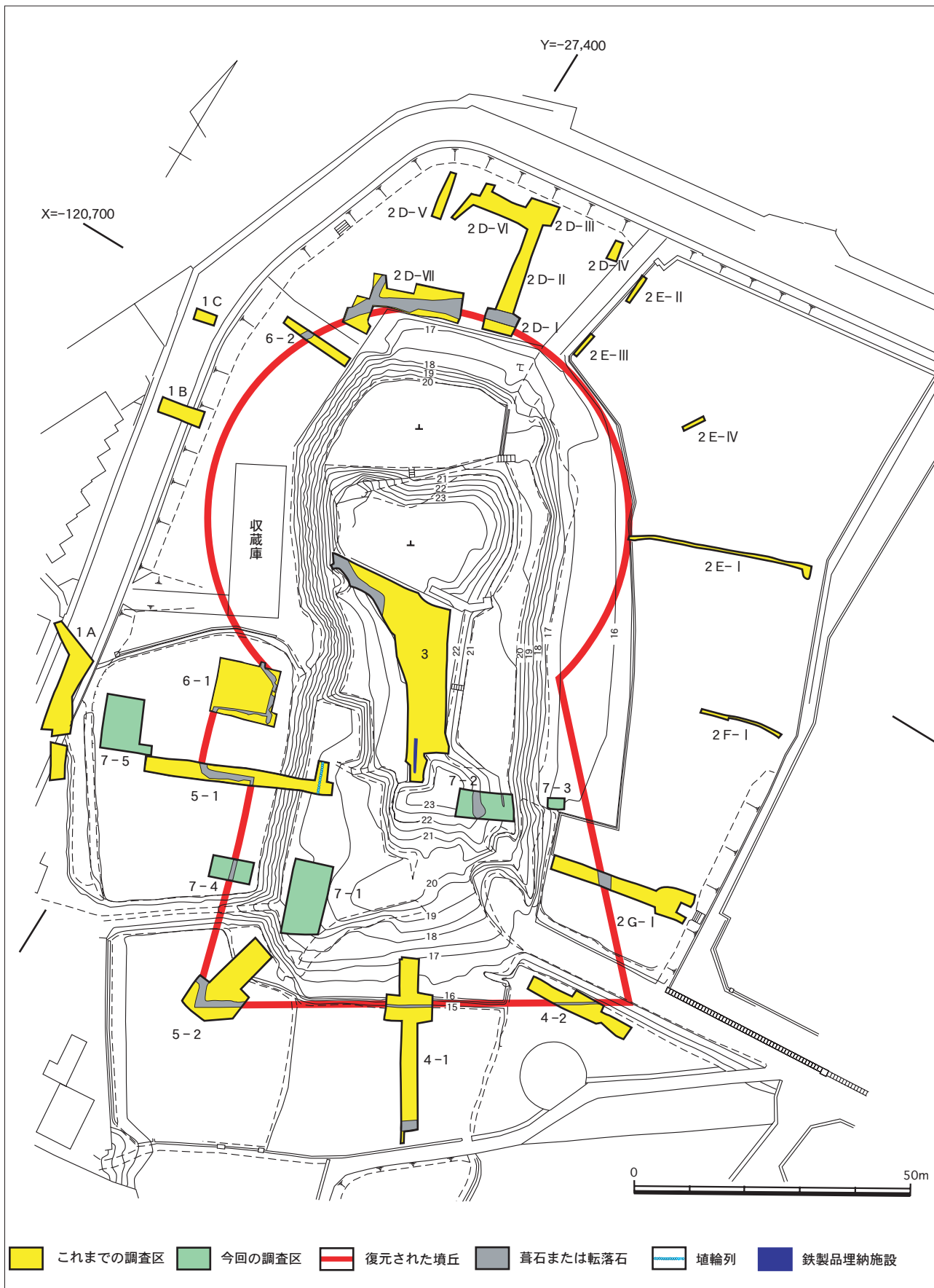
10. 墳丘と調査区の配置 (1/1000)
