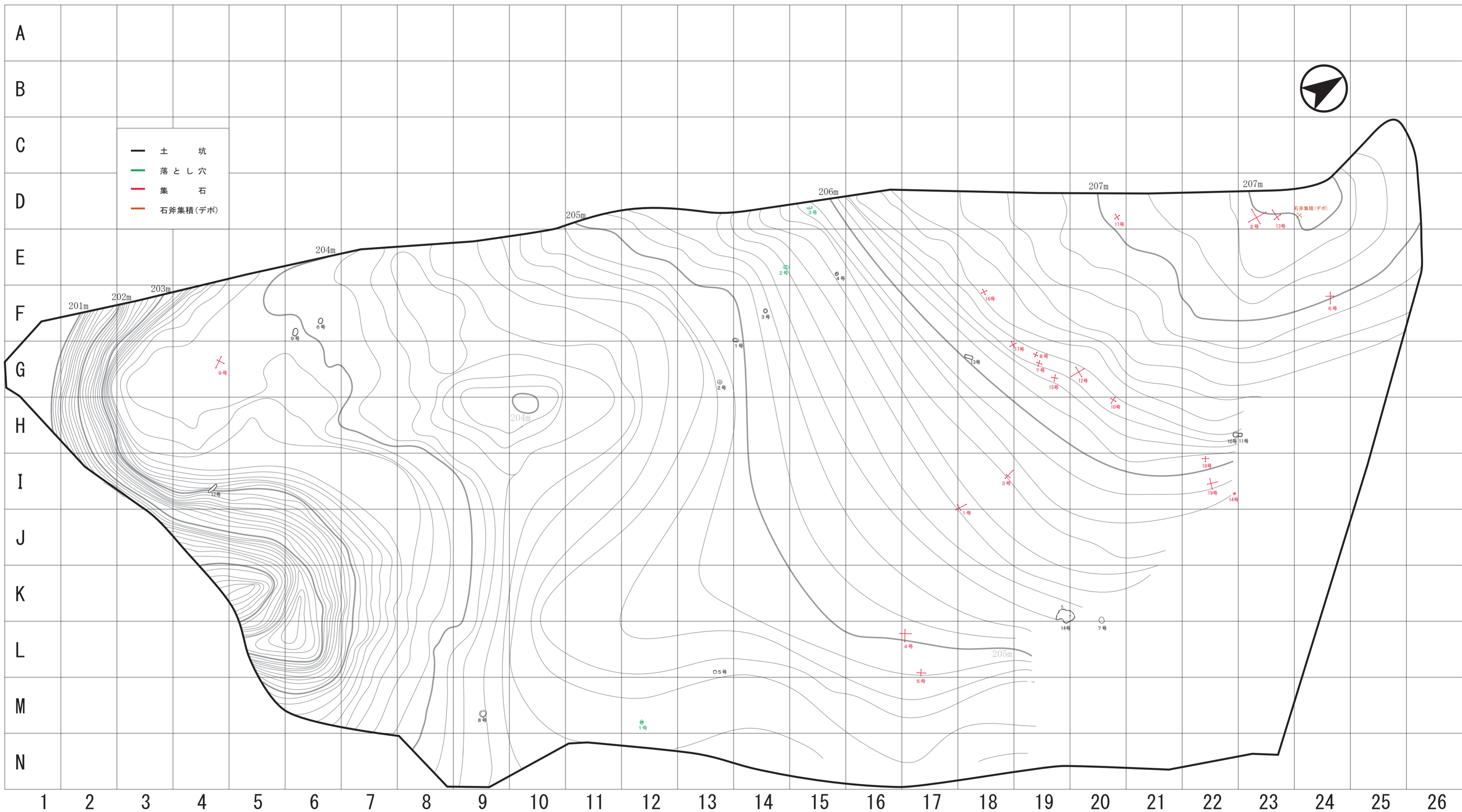
縄文時代前・中期の遺構配置図
