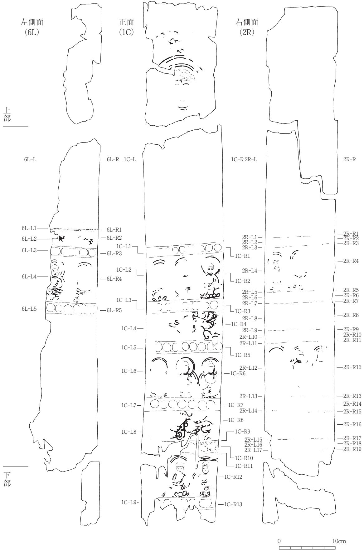
第20図 幢身の仏画画像解析のトレース図
