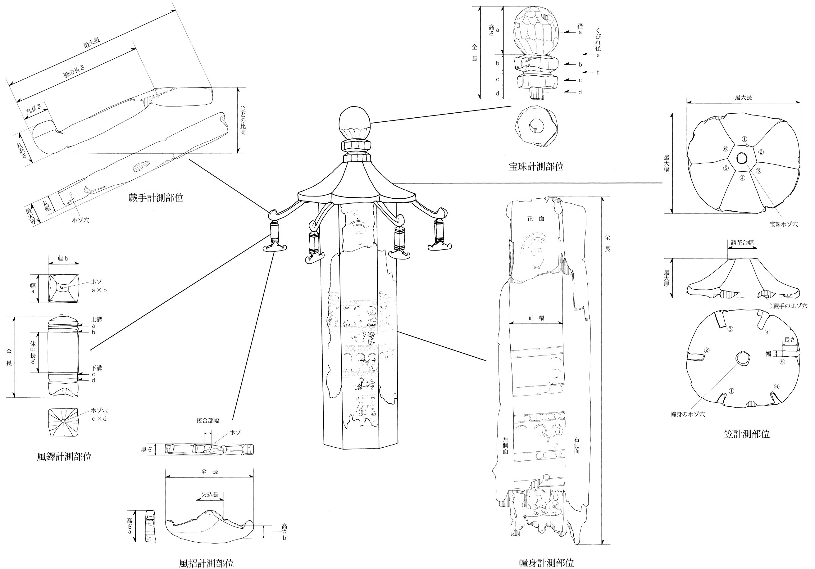
第21図 木幢属性の測定部位 (再掲)
