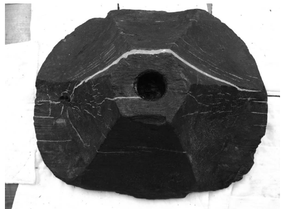
第17図 エポキシ系樹脂パテ剤による亀裂の充填
