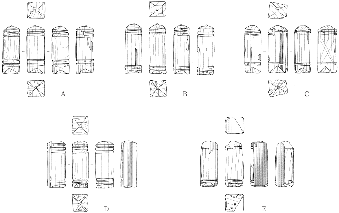
第22図 風招、風鐸年輪 (概念図 S = ¼)
