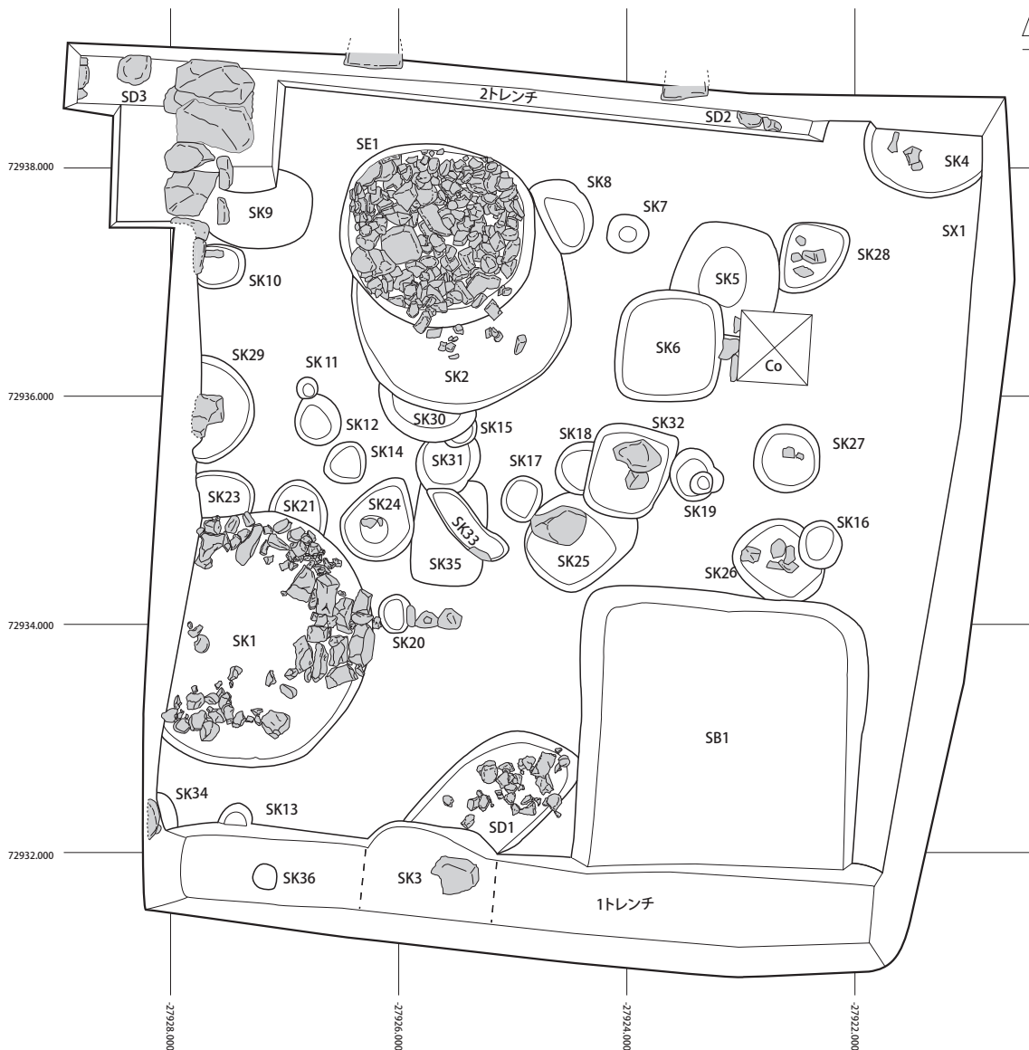
図5 遺構配置図 (1:60)
