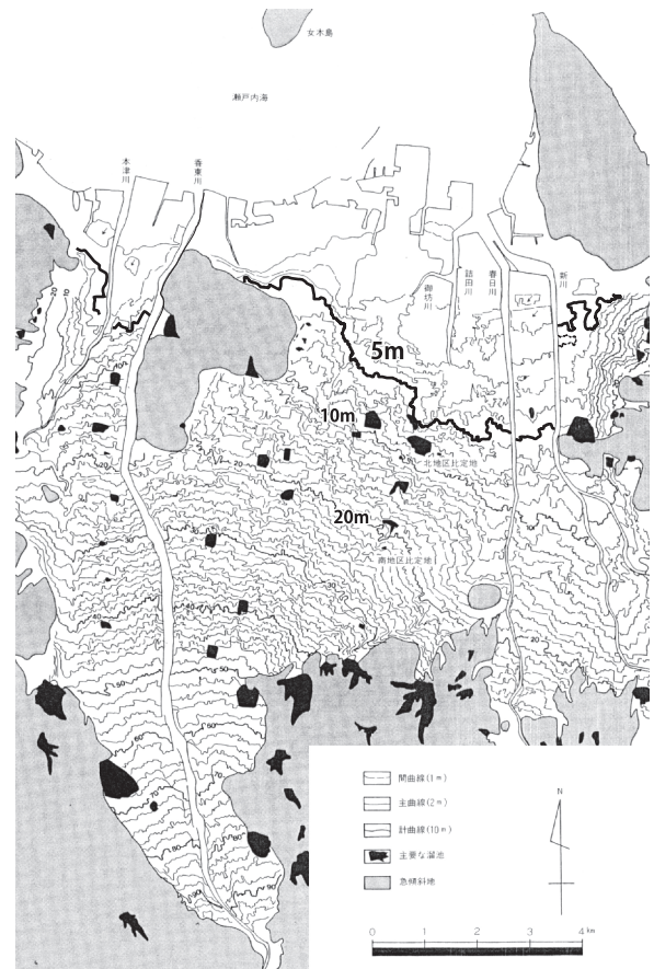
図4-3 高松平野の標高5mライン（渡邊 2016）
