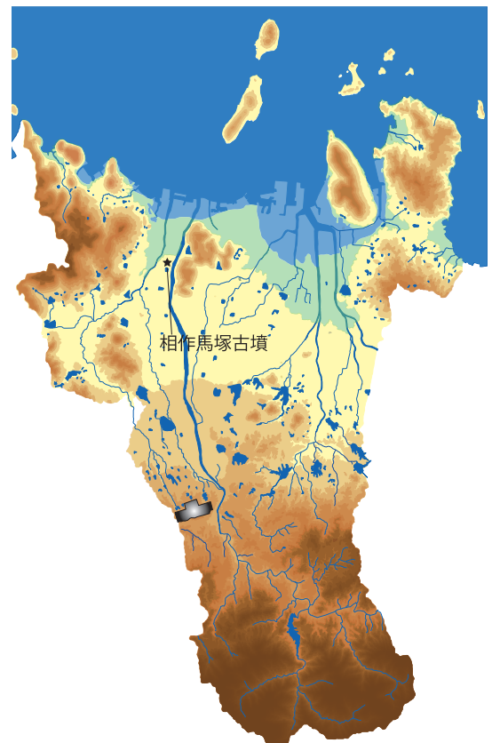
図1-1 高松市の地形図と相作馬塚古墳
