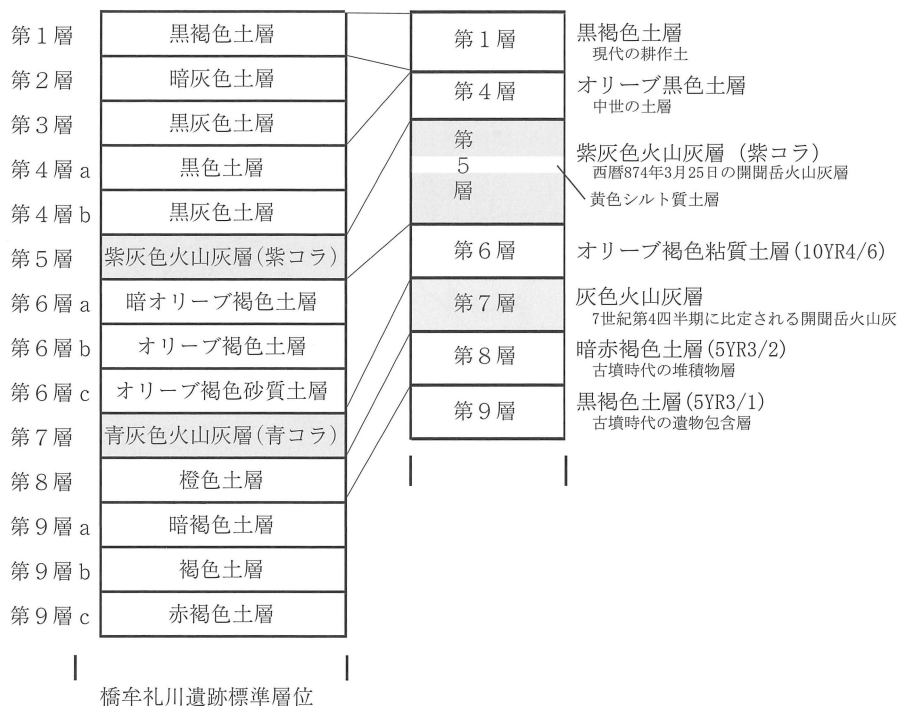
第7図 基本層序図
