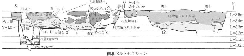
南北ベルトセクション
