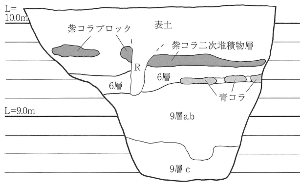
第3図 東壁土層断面図(S=1/40)
