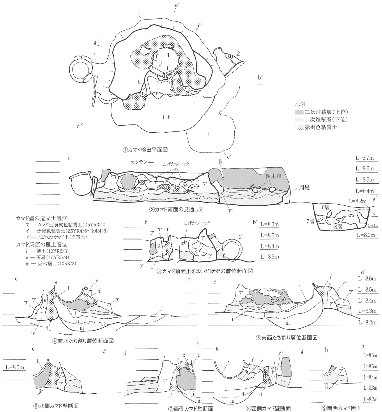
第13図 カマド図1 (S=1/20)
