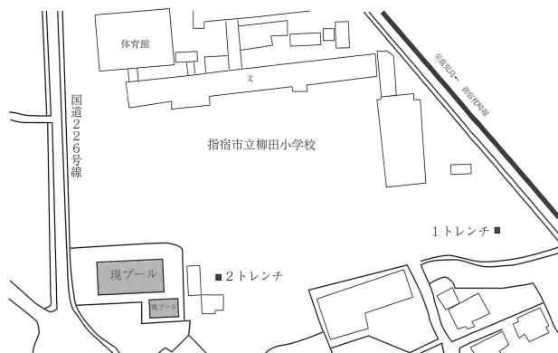
第4図 調査地点およびトレンチ配置図
