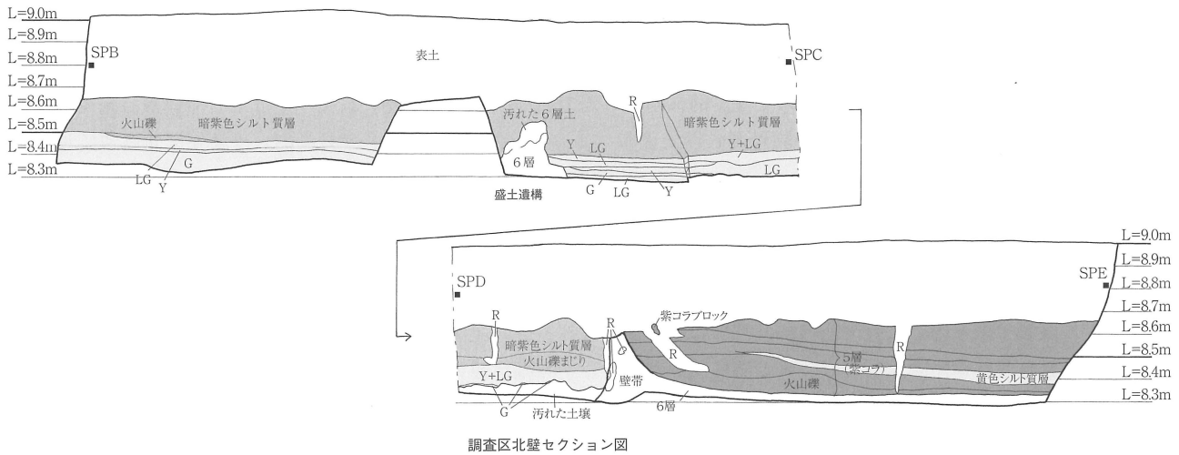
調査区北壁セクション図
