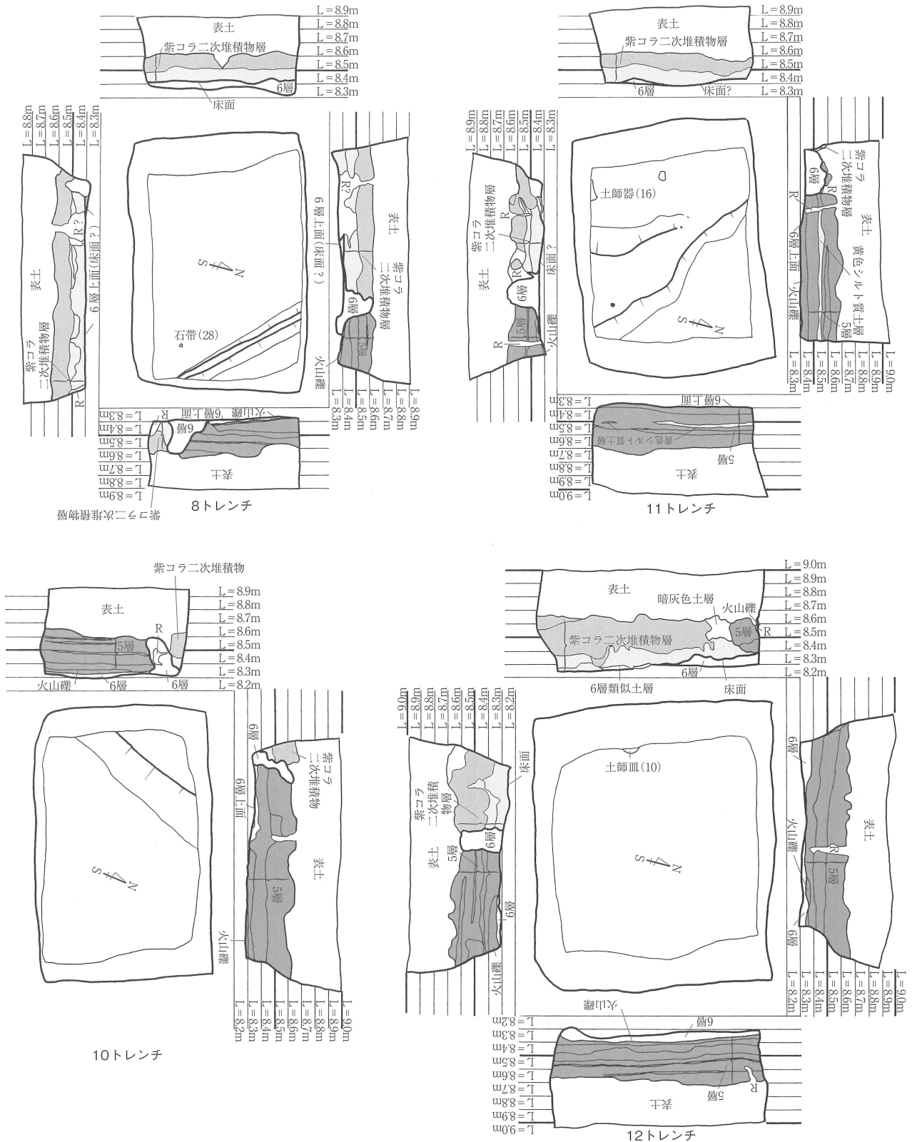
第3図 試掘トレンチ図1(S=1/40)
