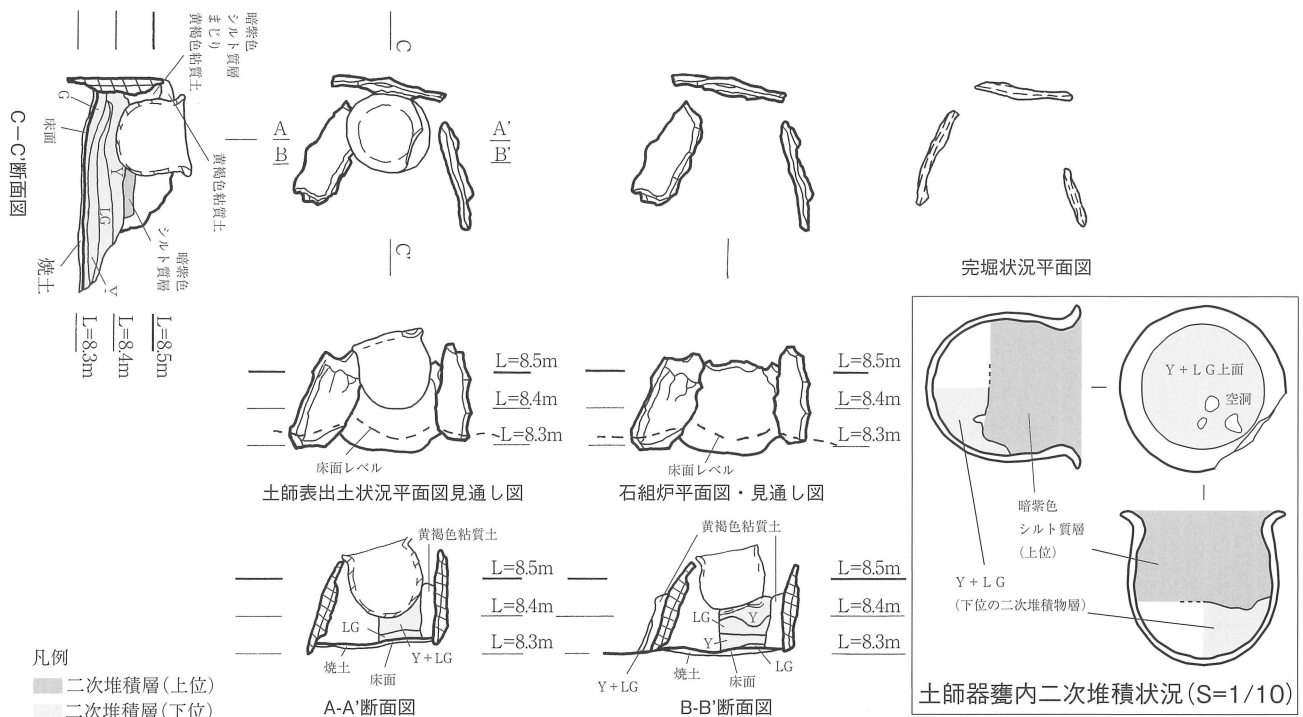
第16図 石組炉 (S=1/20)
