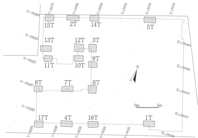
第5図 試掘トレンチの位置図(S=1/500)
