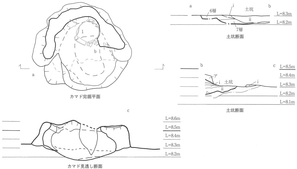
第14図 カマド図2 (S=1/20)
