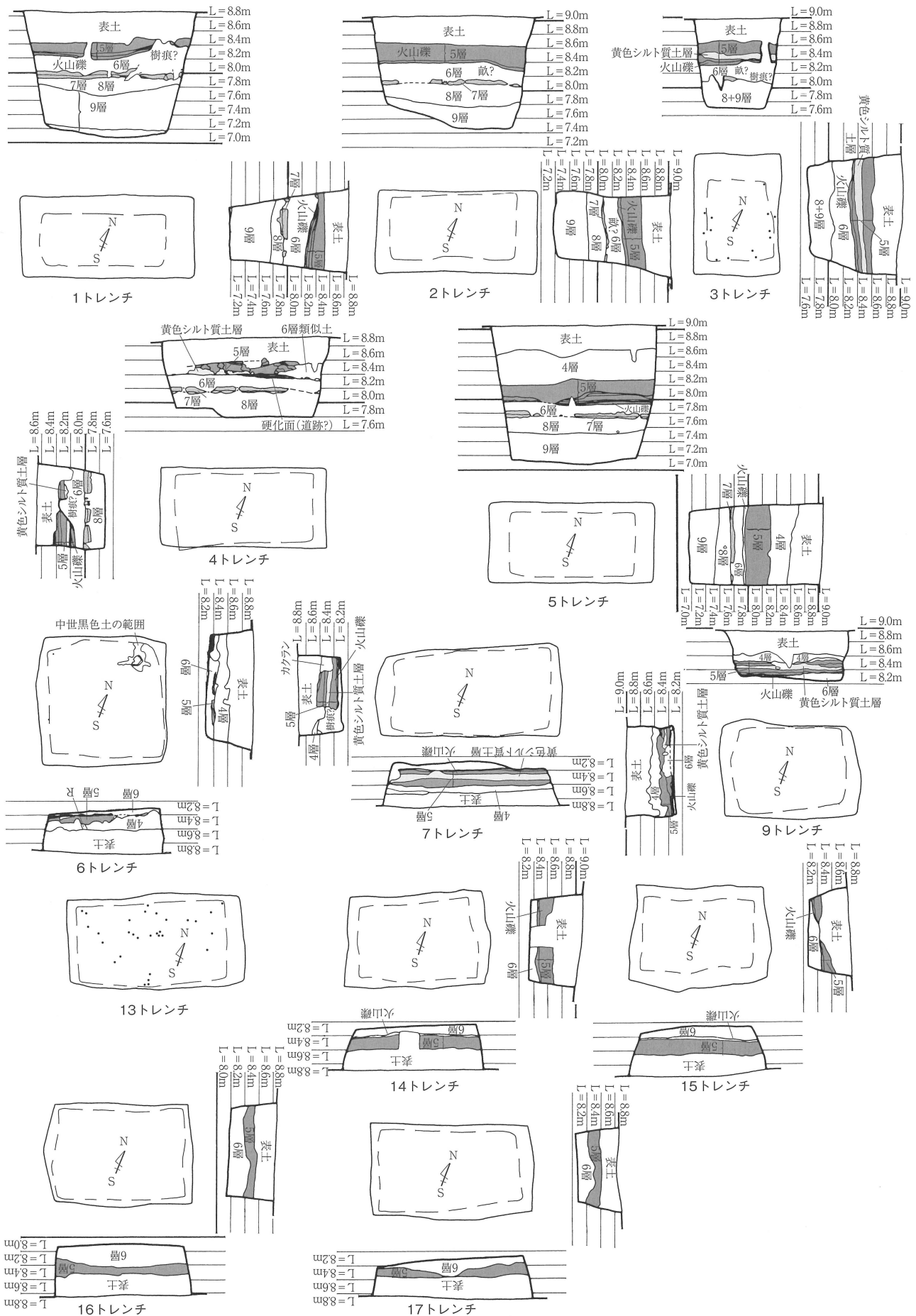
第4図 試掘トレンチ図2 (S=1/75)
