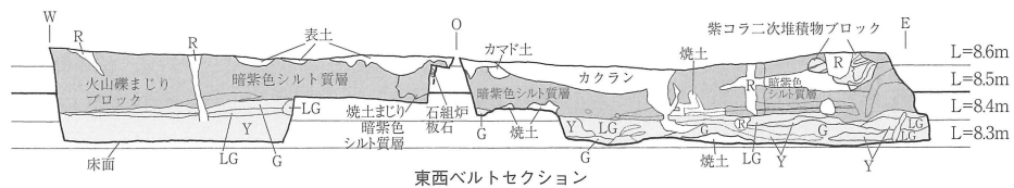
東西ベルトセクション
