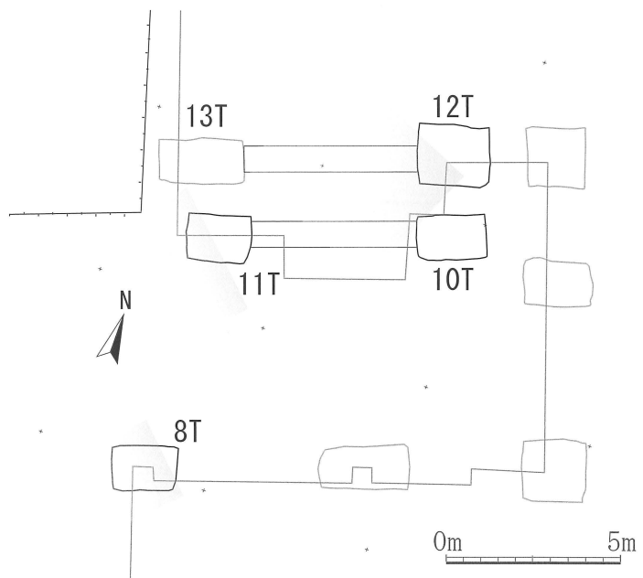
第6図 遺構配置想定図(S=1/200)
