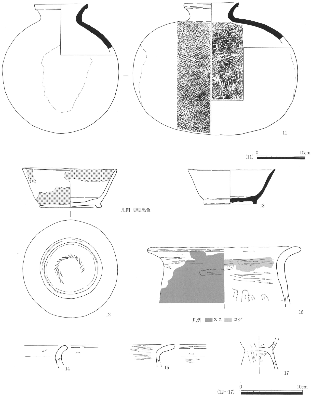
第20図 遺物図面② (11:S=1/4 12~17:S=1/3)
