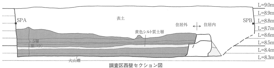
調査区西壁セクション図
