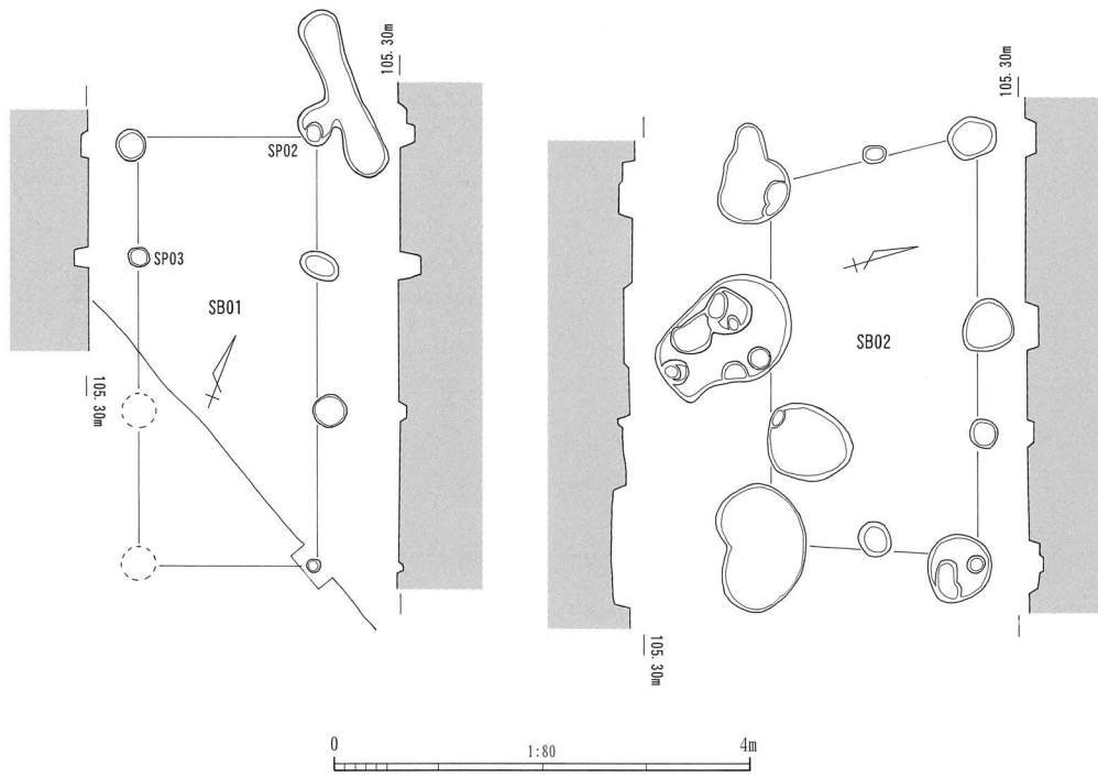
図8 SB01・02掘立柱建物
