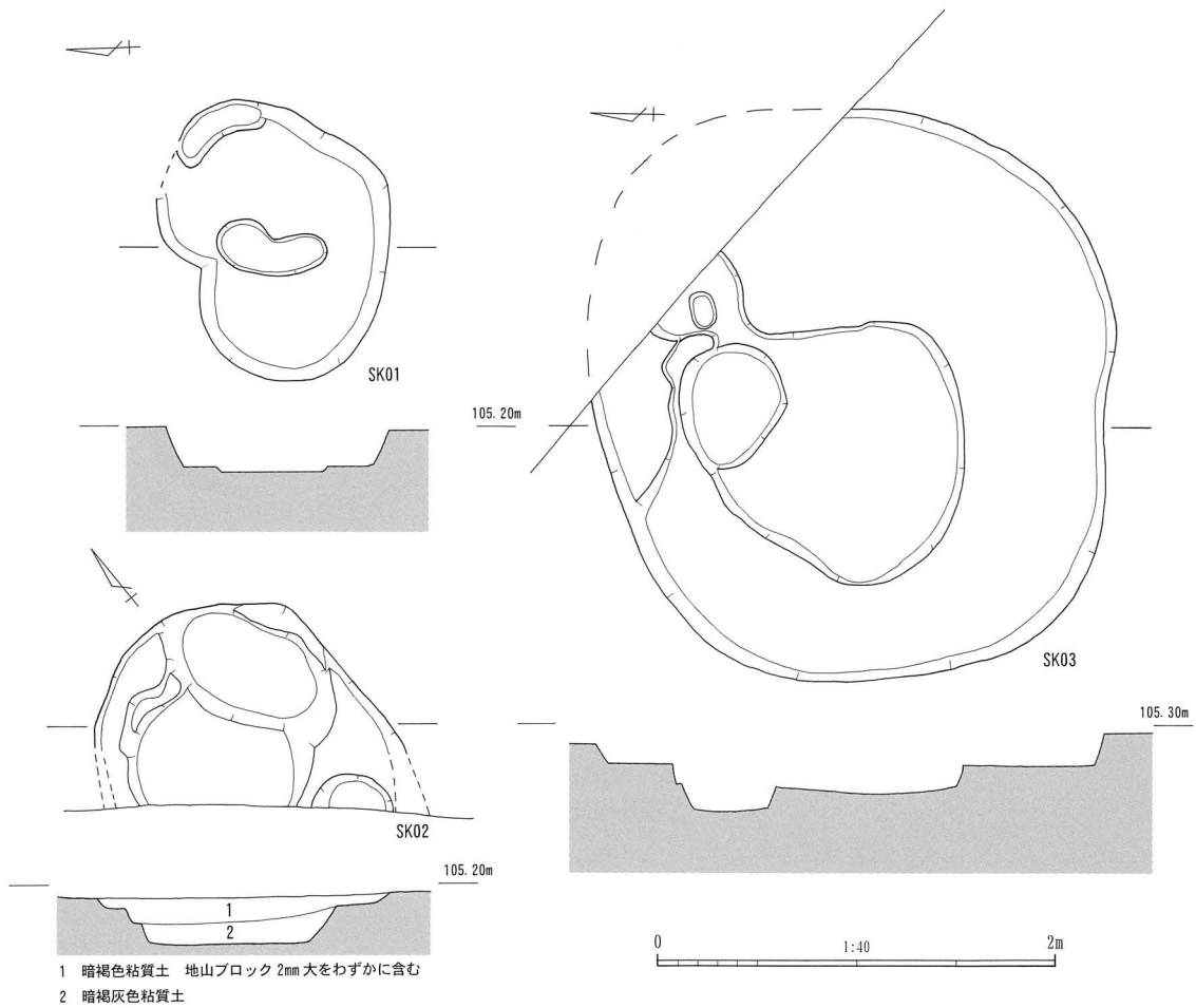
図9 SK01・02・03土坑
