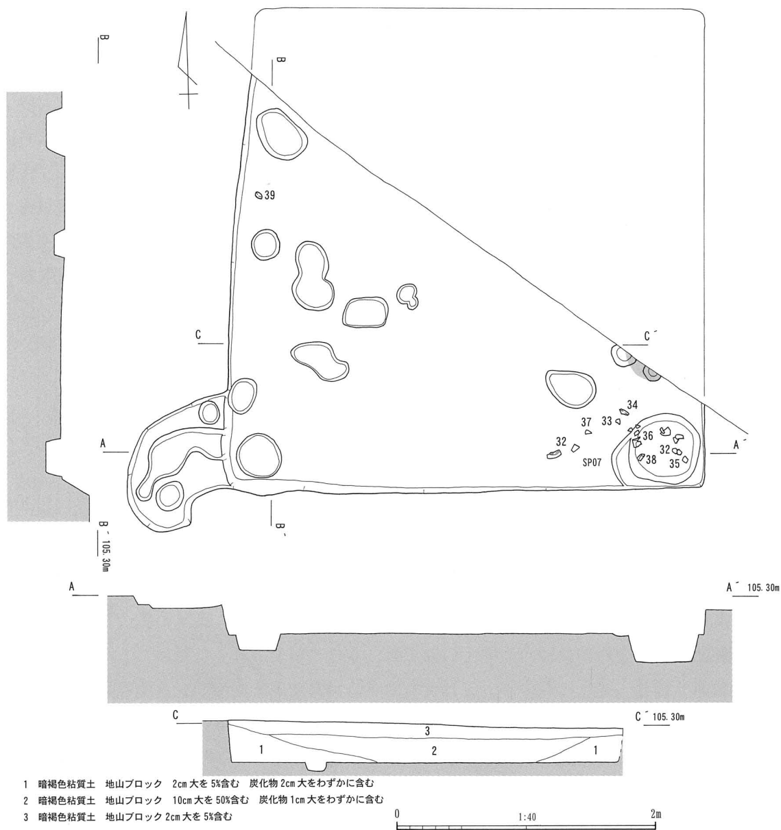
図4 SH 01 竪穴建物
