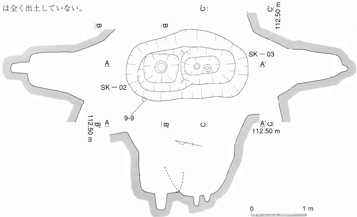
第10図 SK-02・03実測図
