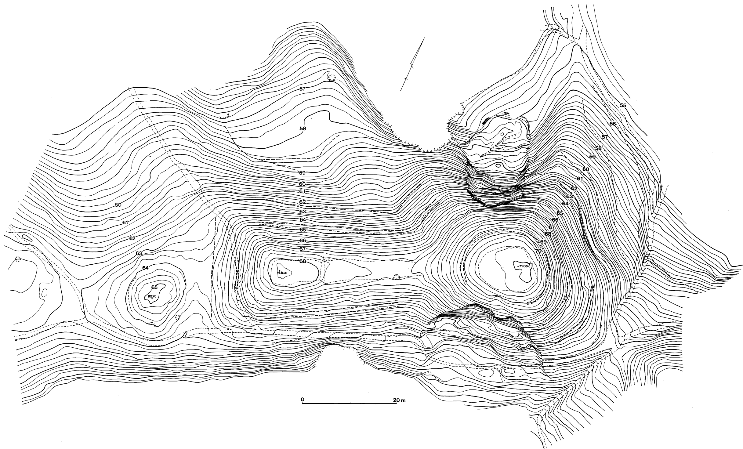
第4图 大元古墳群墳丘実測図
