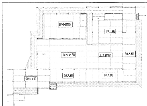
解体修理前の御書院平面図
