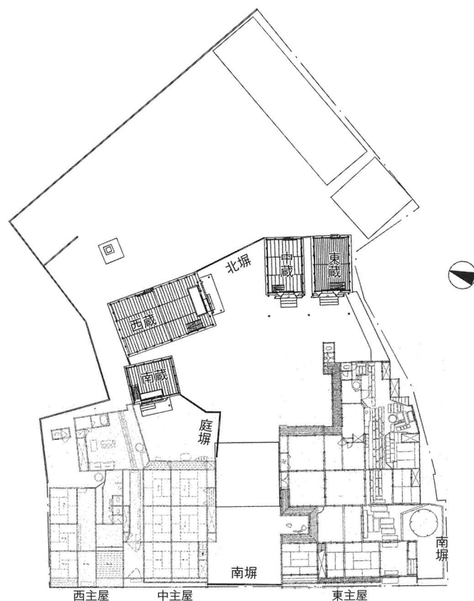
旧石橋家住宅平面図
