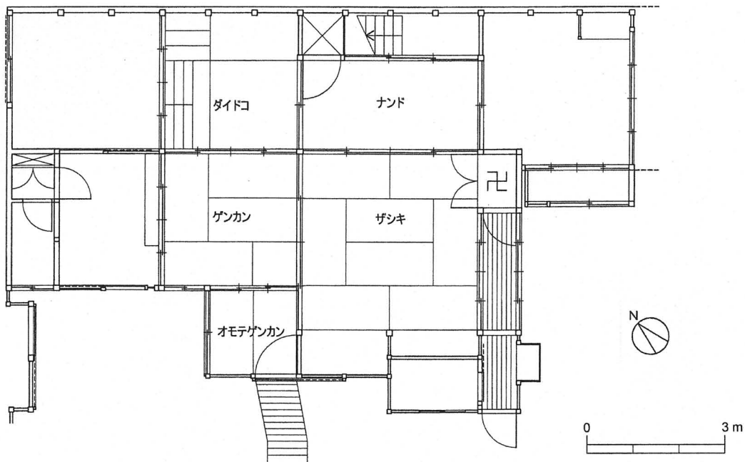
北川家住宅平面図
