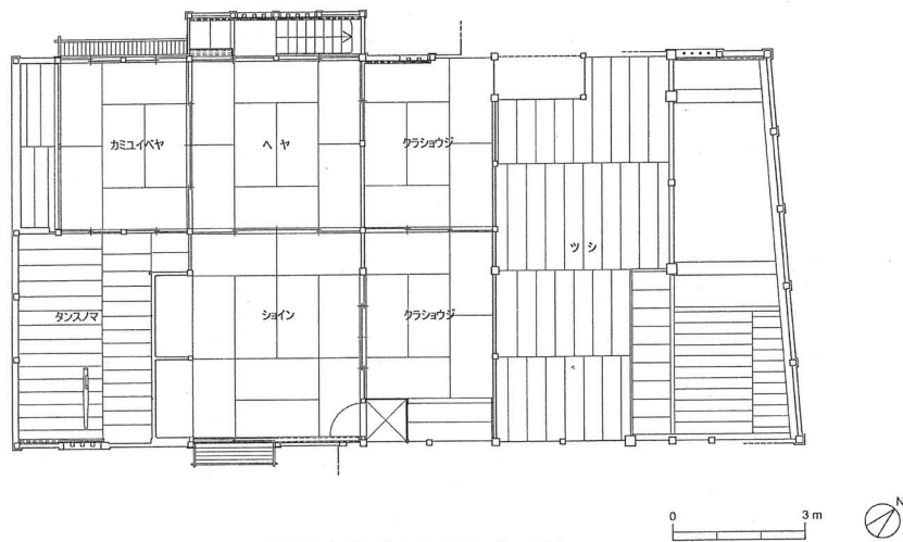
馬場家住宅平面図（2階）
