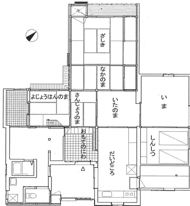
道路 旧磯崎家住宅平面図
