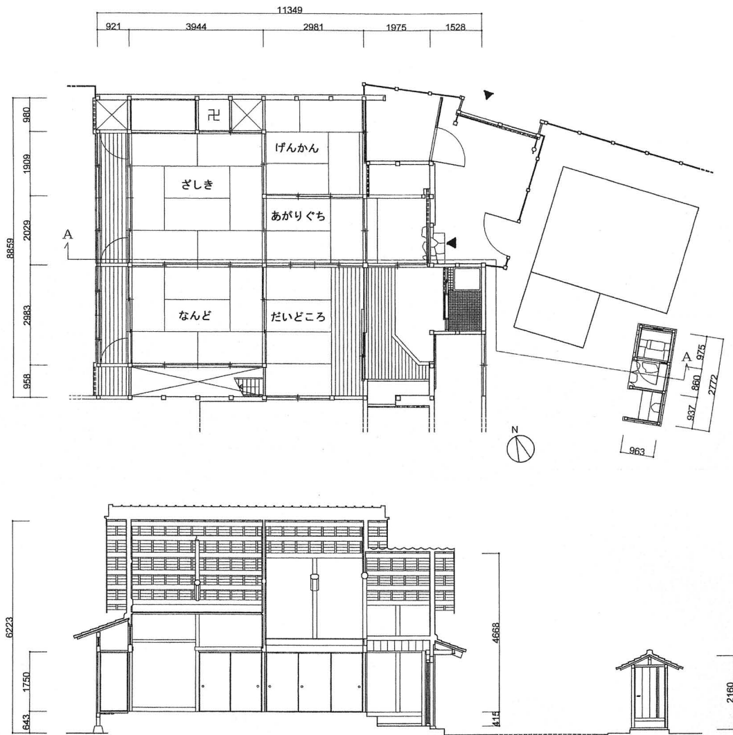
瀧谷家住宅平面図・立面図
