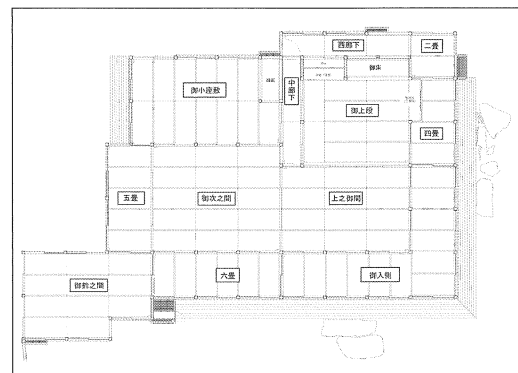
解体修理後の御書院平面図
