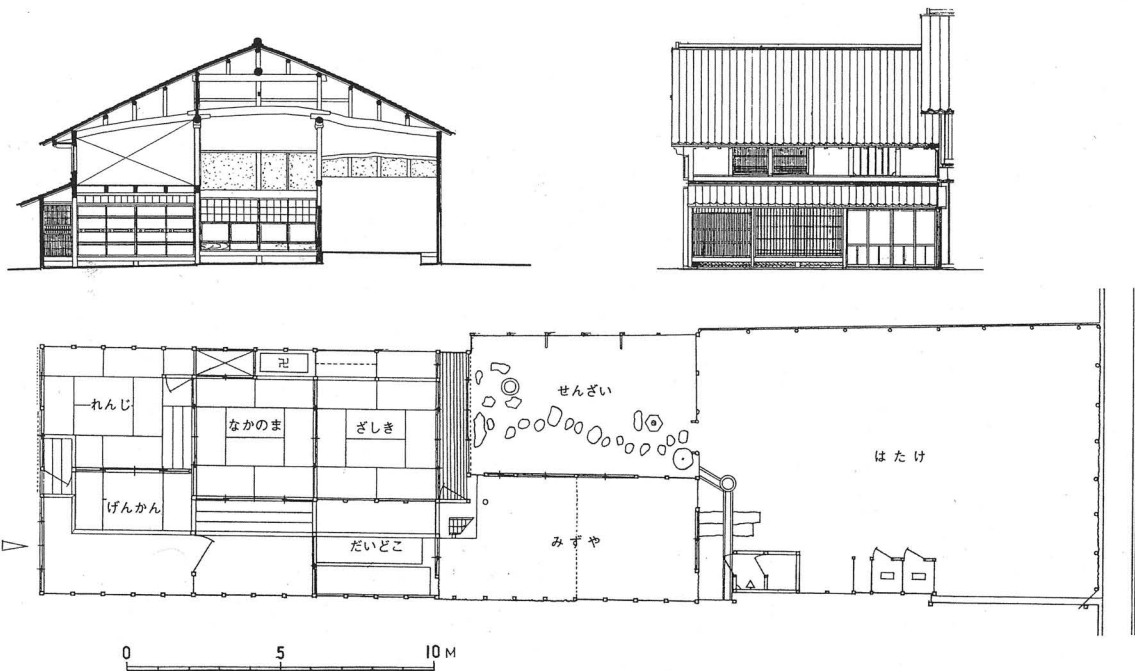
吉川家住宅平面図・立面図
