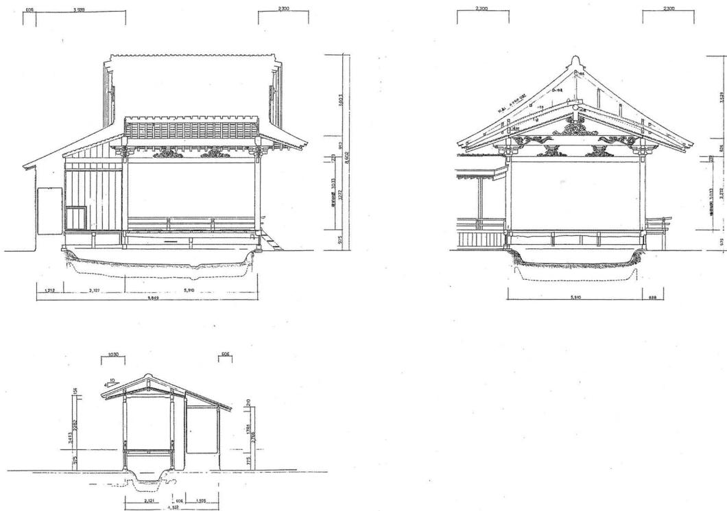
彦根城表御殿の能舞台の立面図
