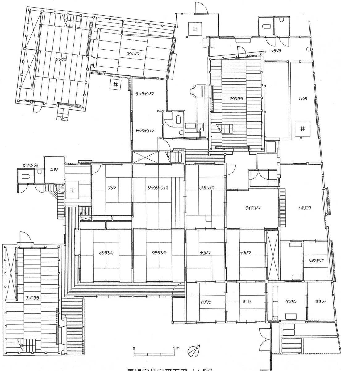
馬場家住宅平面図（1階）
