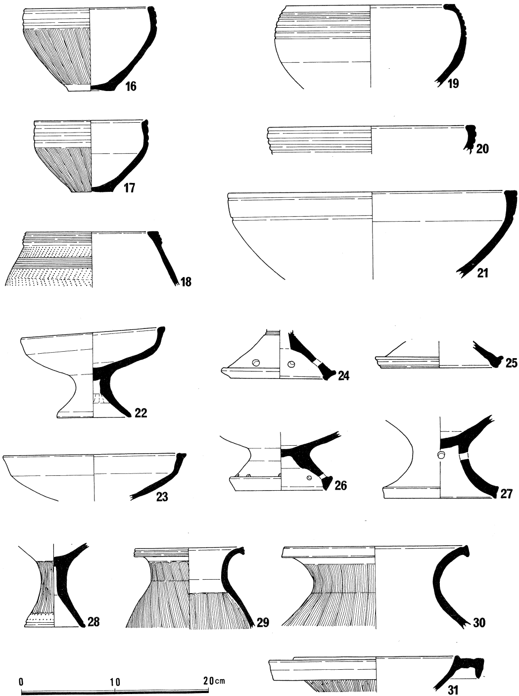
第6图 出土遺物実測図(2)
