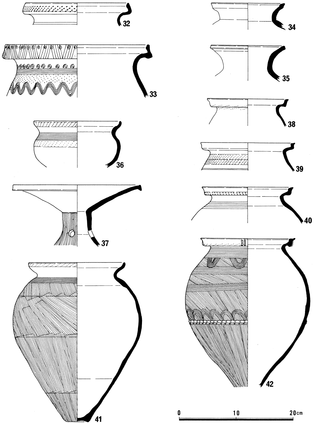
第7图 出土遺物実測図(3)
