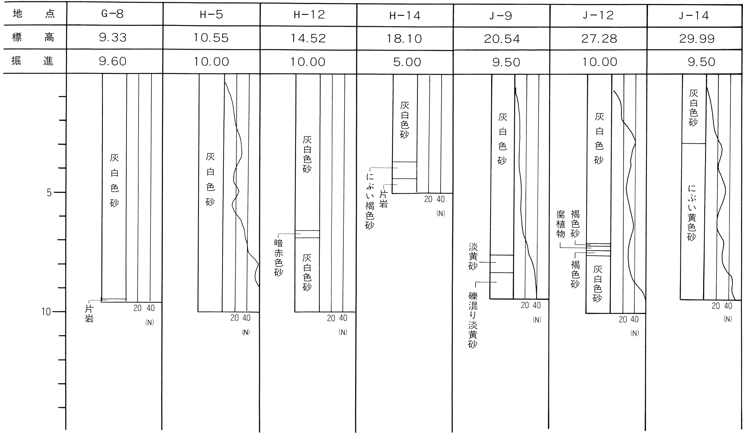
第9図 柱状図(2)
