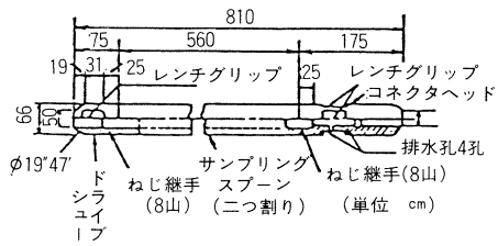
(a) 遺跡調査用サンブラー
