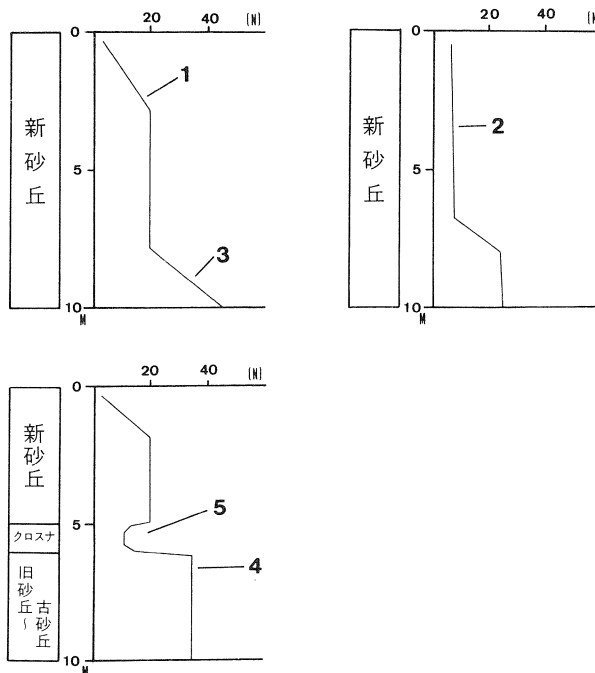
第16図 貫入試験模式図
