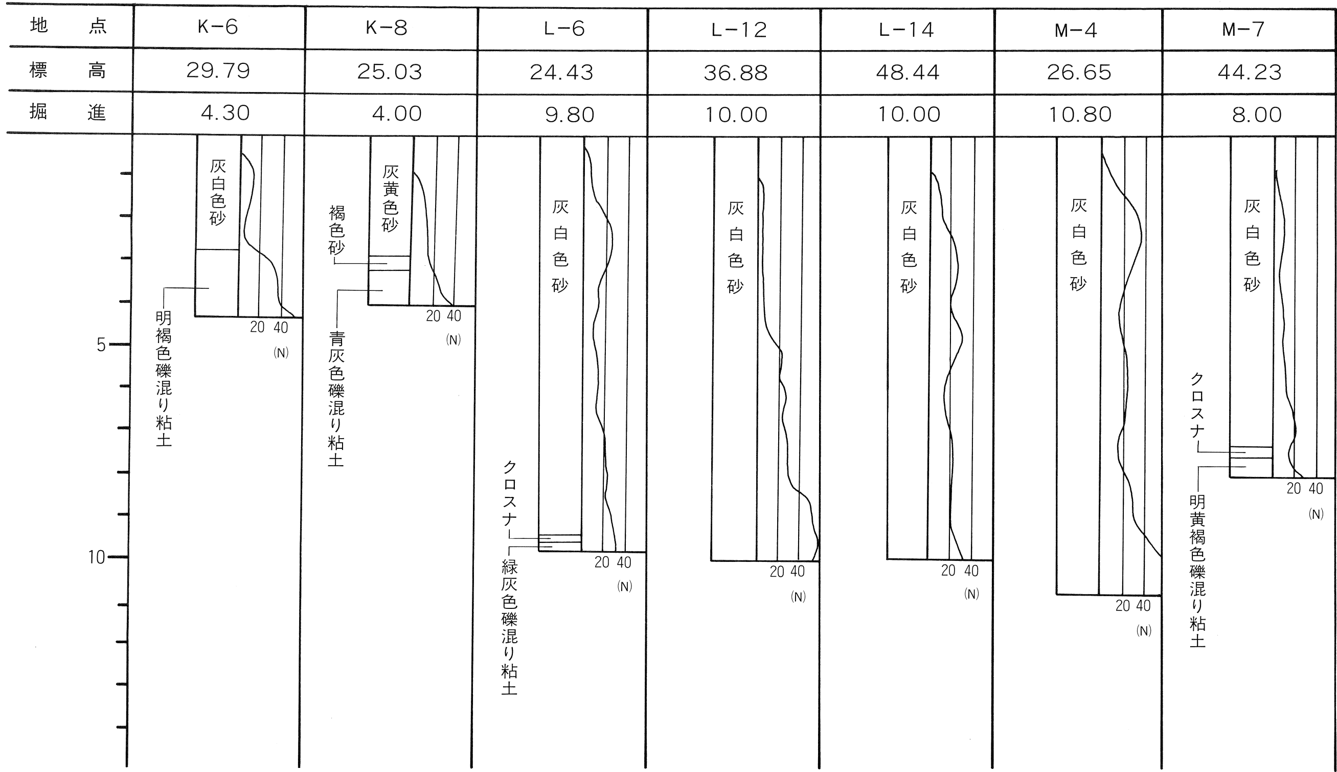
第10図 柱状図 (3)
