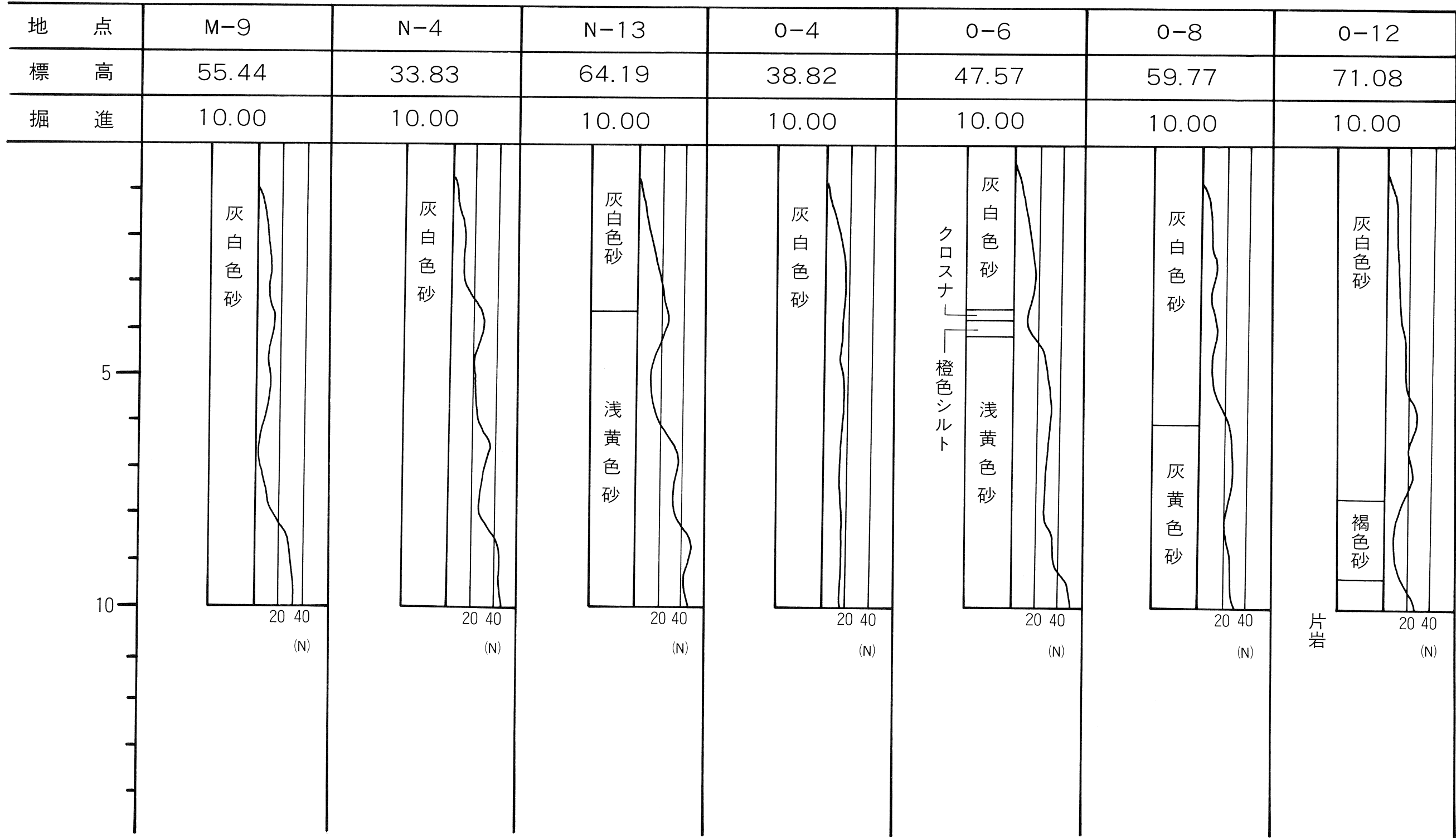
第11図 柱状図 (4)
