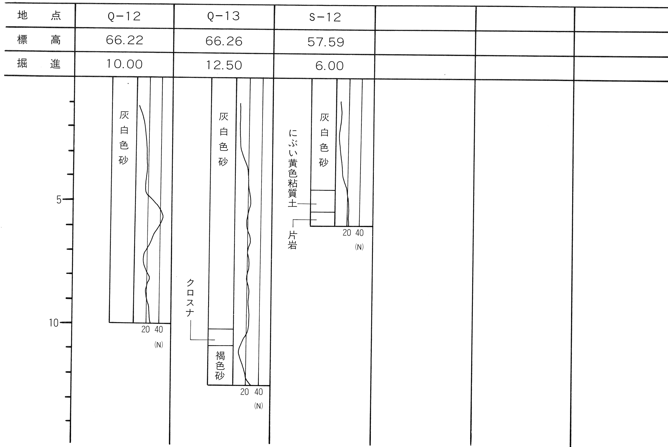
第12図 柱状図 (5)
