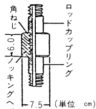
(b) ノッキングヘッド
