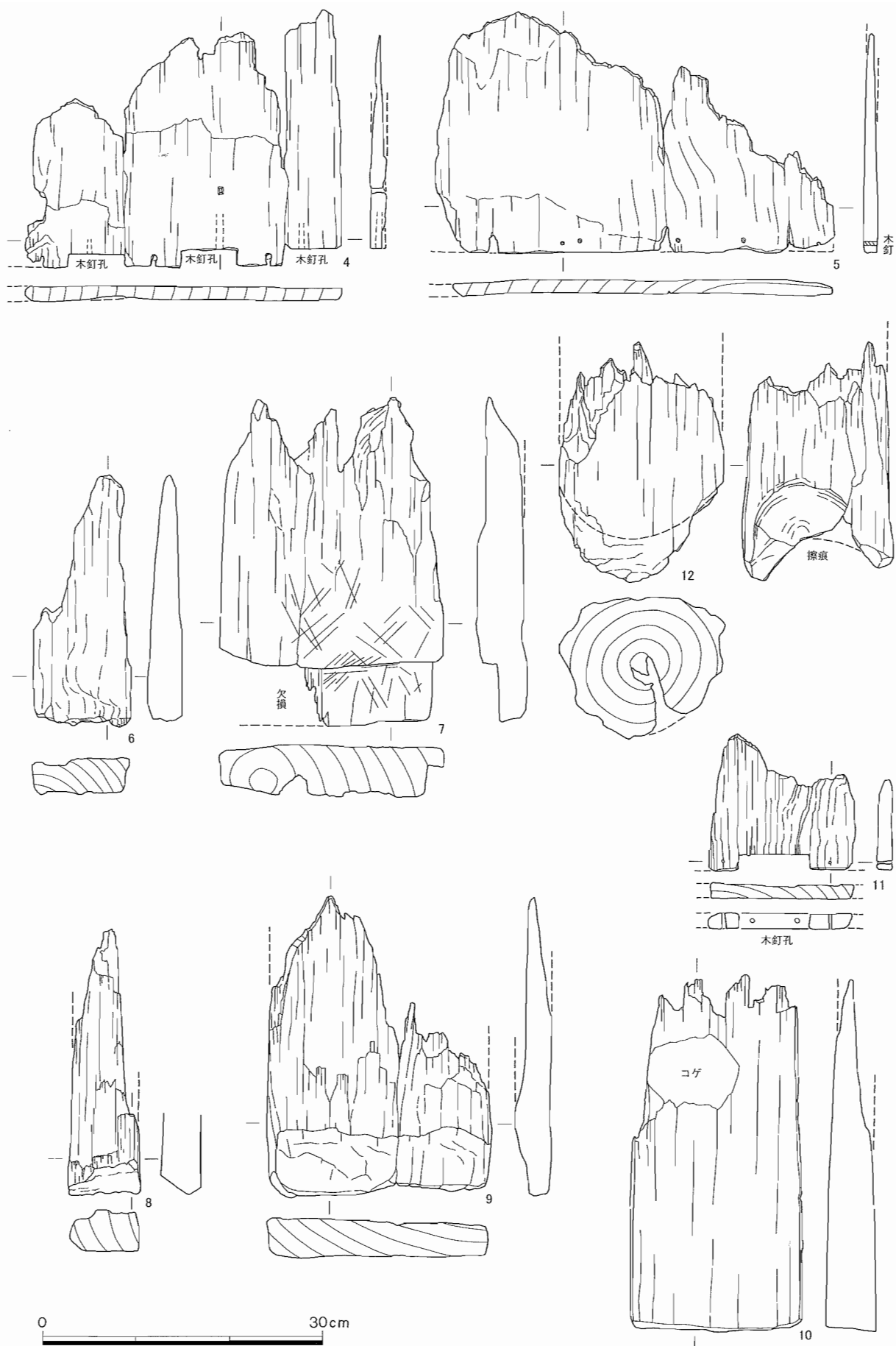
第8図 出土木製品実測図 2
