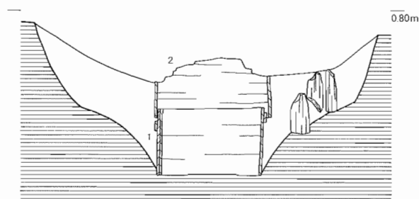
第3図 A地区遺構図 (サインポール地点)
