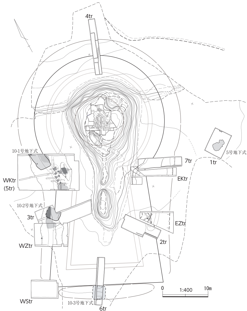
図 11 墳丘平面図
