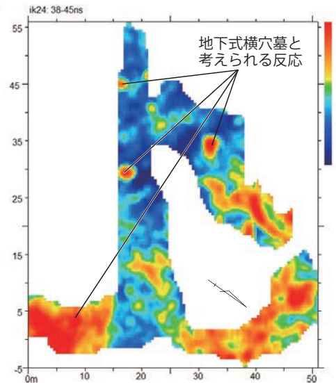
図 10 神領 10 号墳地中レーダー探査
