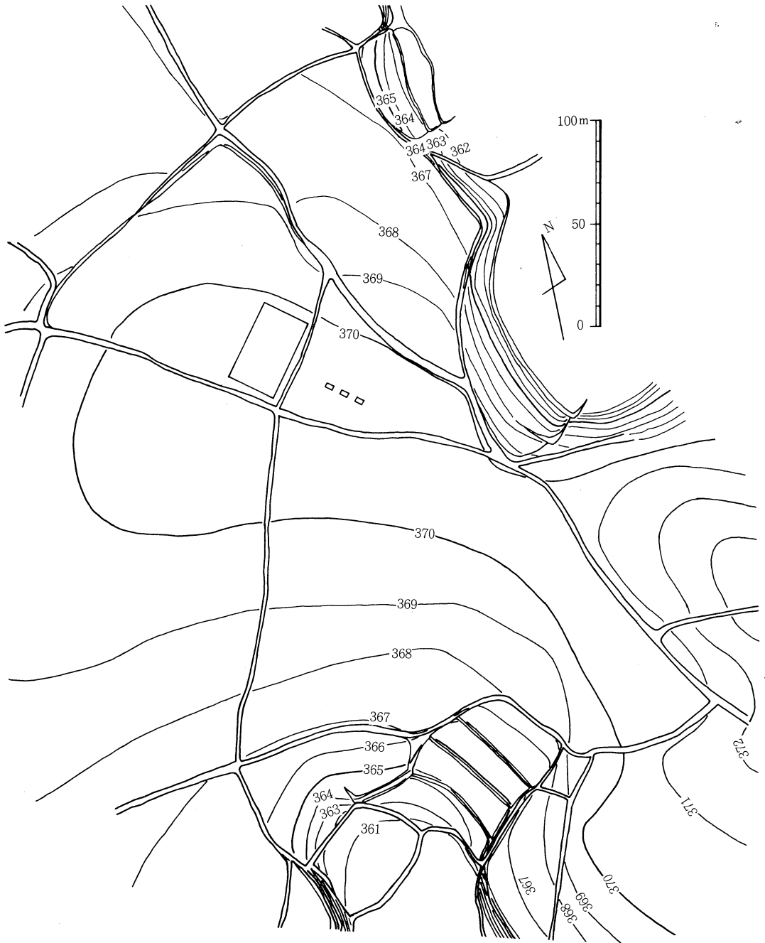
第1図 小高野遺跡地形図
