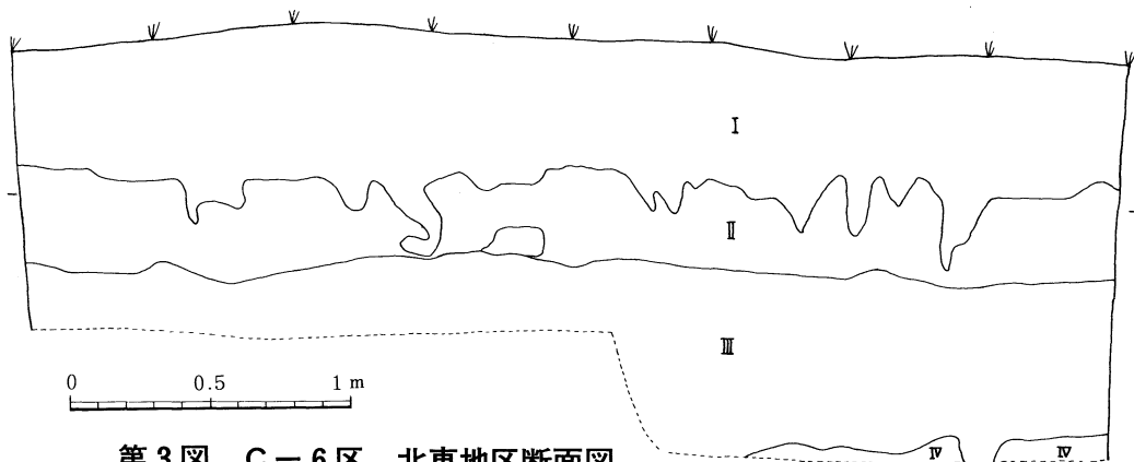
第3図 C-6区 北東地区断面図
