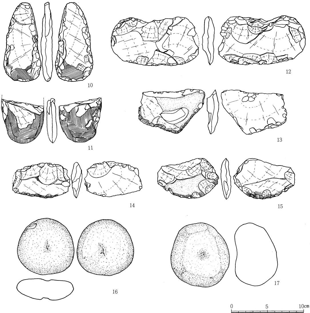
第11図 石器実測図3
