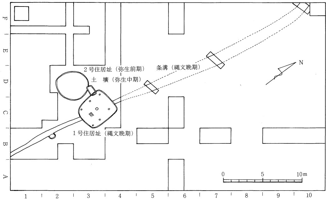
第2図 遺跡発掘実測図
