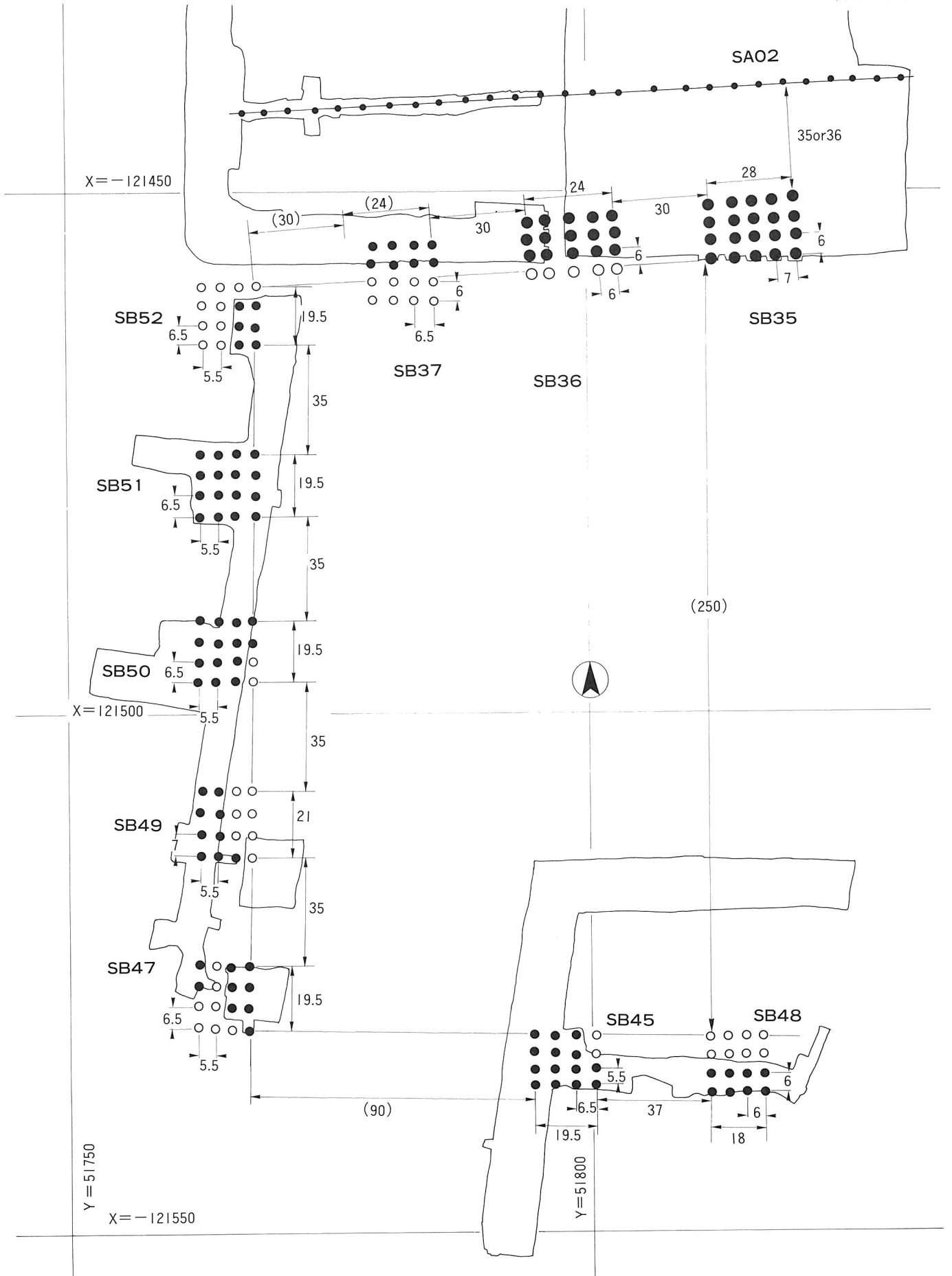
正倉配置図 (1 : 500)
