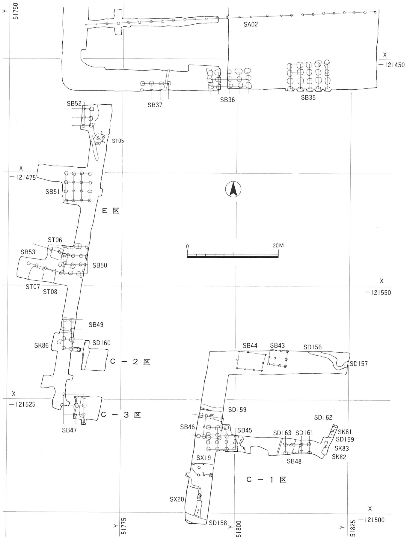
狐塚遺跡主要遺構配置図 (1:500)
