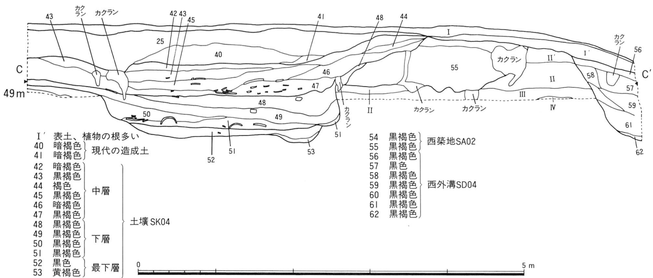
6AJA-A-5 土層断面図 (1:50)
