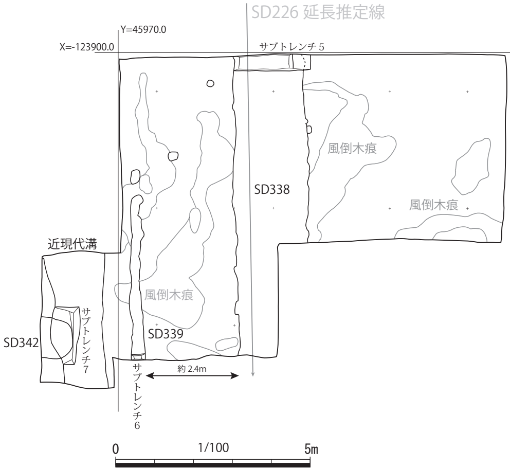
Fig.11 6AIF-F 区遺構平面図 (1:100)
