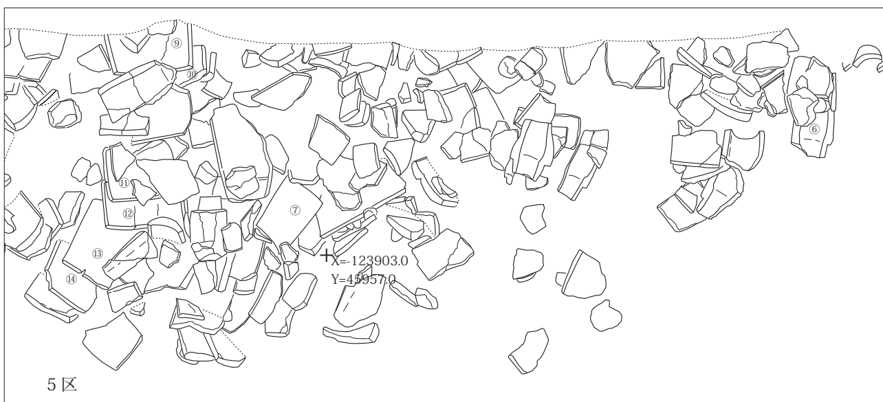
Fig.10 6AIF-A区瓦出土状況図 (1:20)
