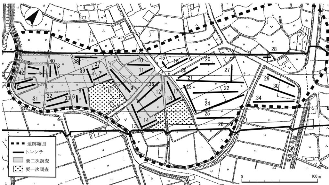
図29 釜垣内遺跡（一次）トレンチ配置図（1 : 2,500）
