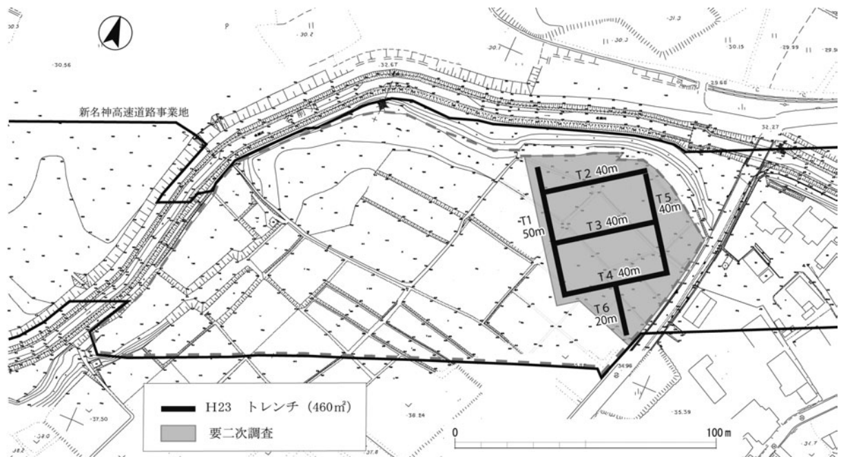
図28 トレンチ配置図（1：2,000）
