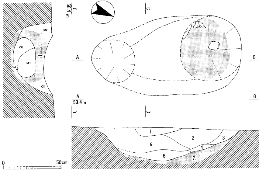
図11 SF1125実測図 (1:20)
