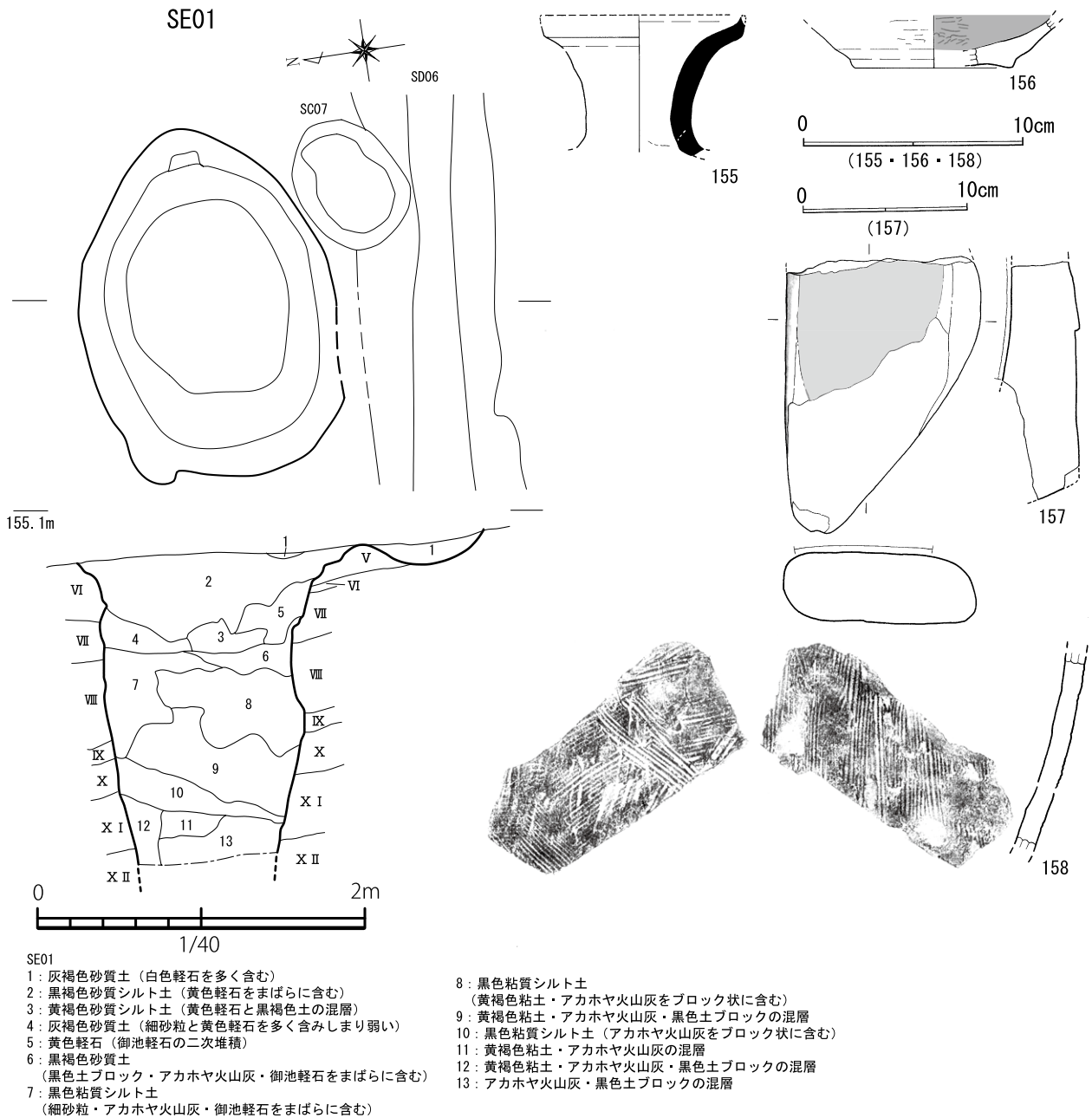
第21図 SE01実測図 (S=1/40) ・ 出土遺物実測図 (石器 : S=1/4、その他 : S=1/3)
