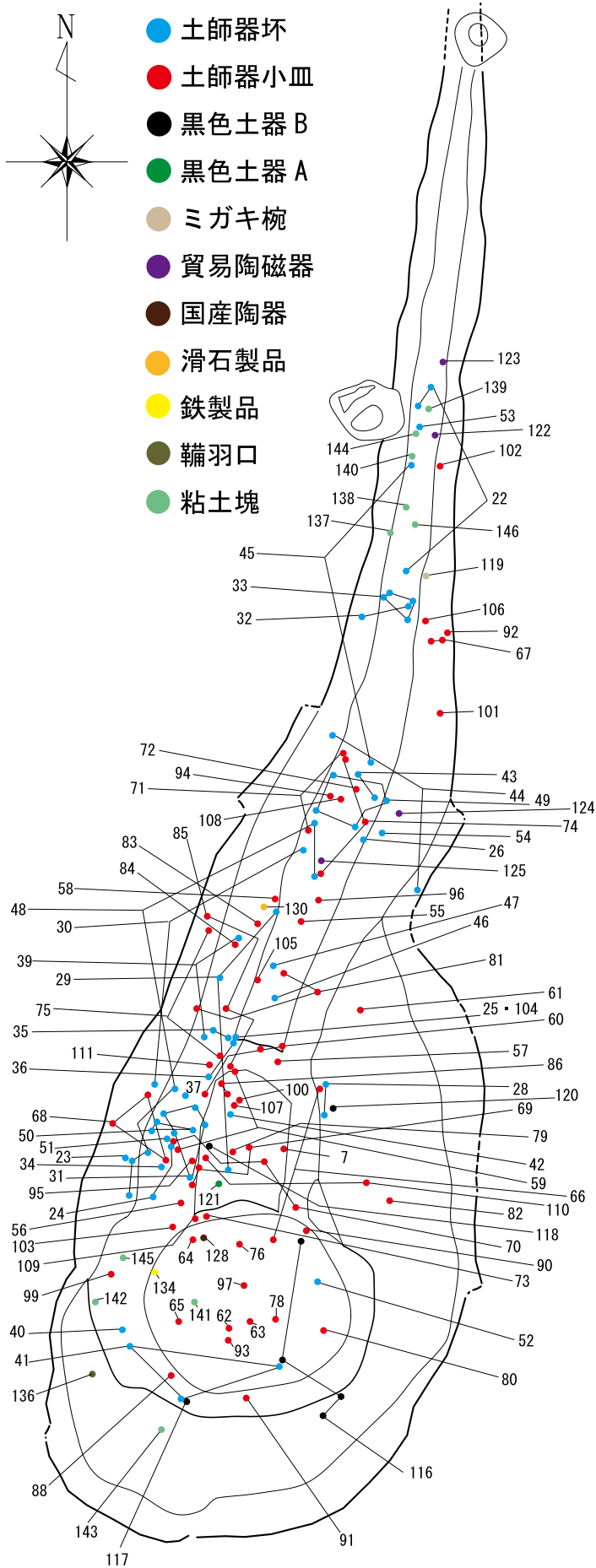
第18図 SD03 遺物出土状況 (S=1/40)
