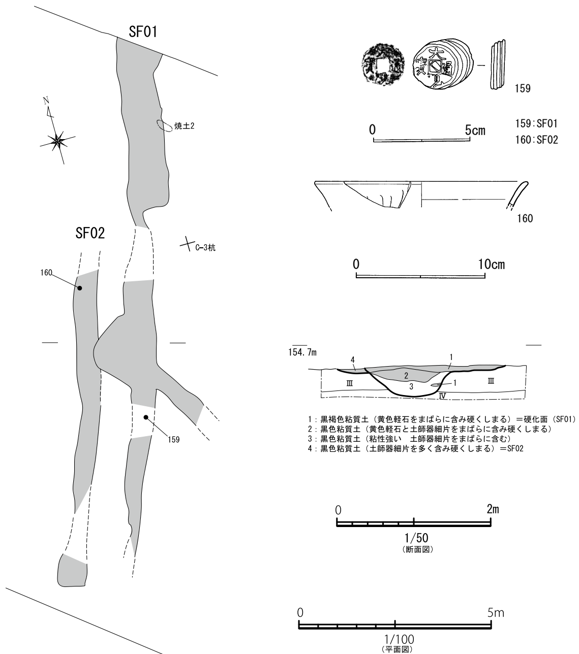
第22図 SF01・02実測図（平面図：S=1/100、断面図：S=1/50） 出土遺物実測図（古銭：S=1/2、貿易陶磁器：S=1/3）
