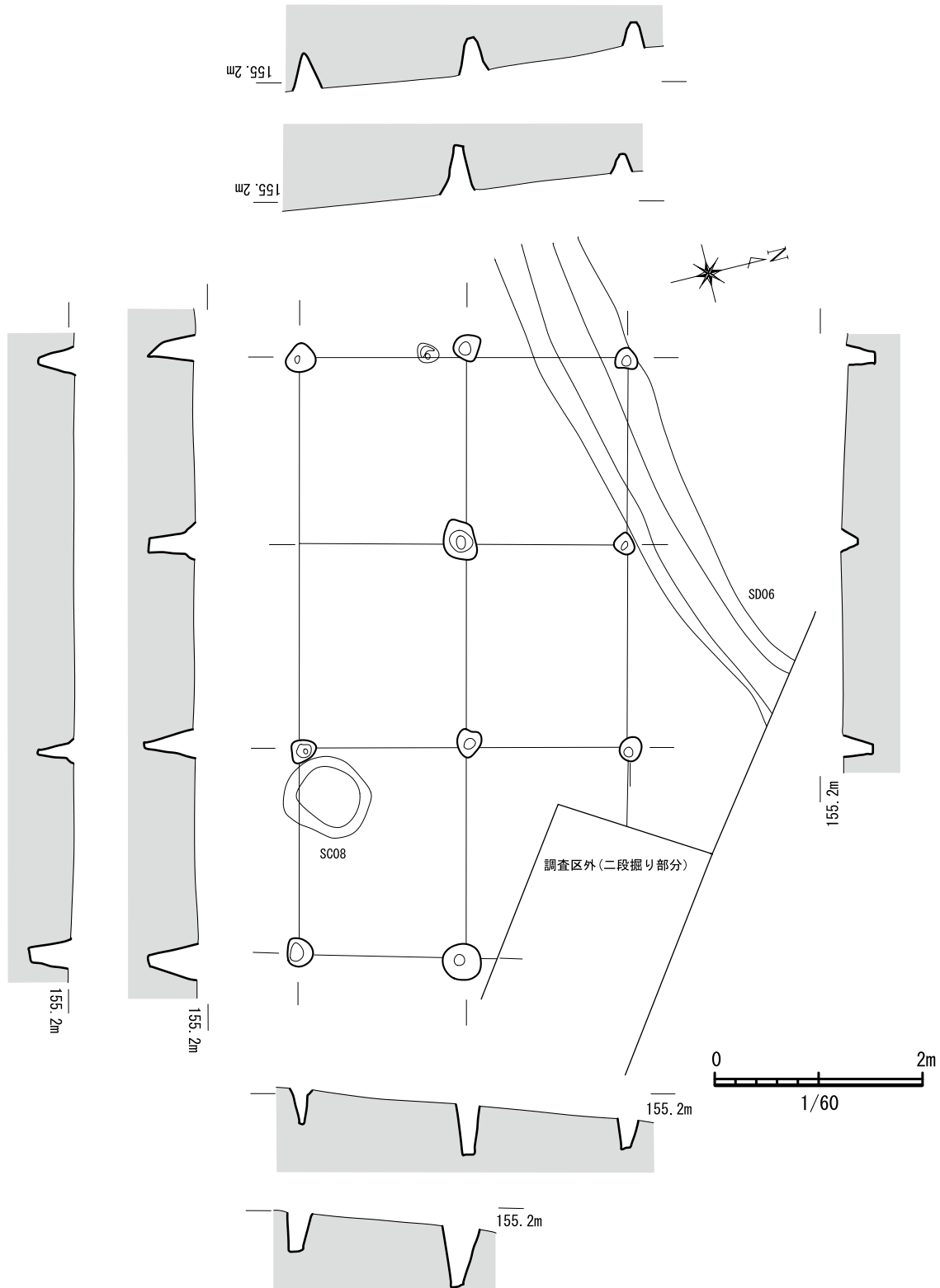
第6図 SB01実測図 (S=1/60)
