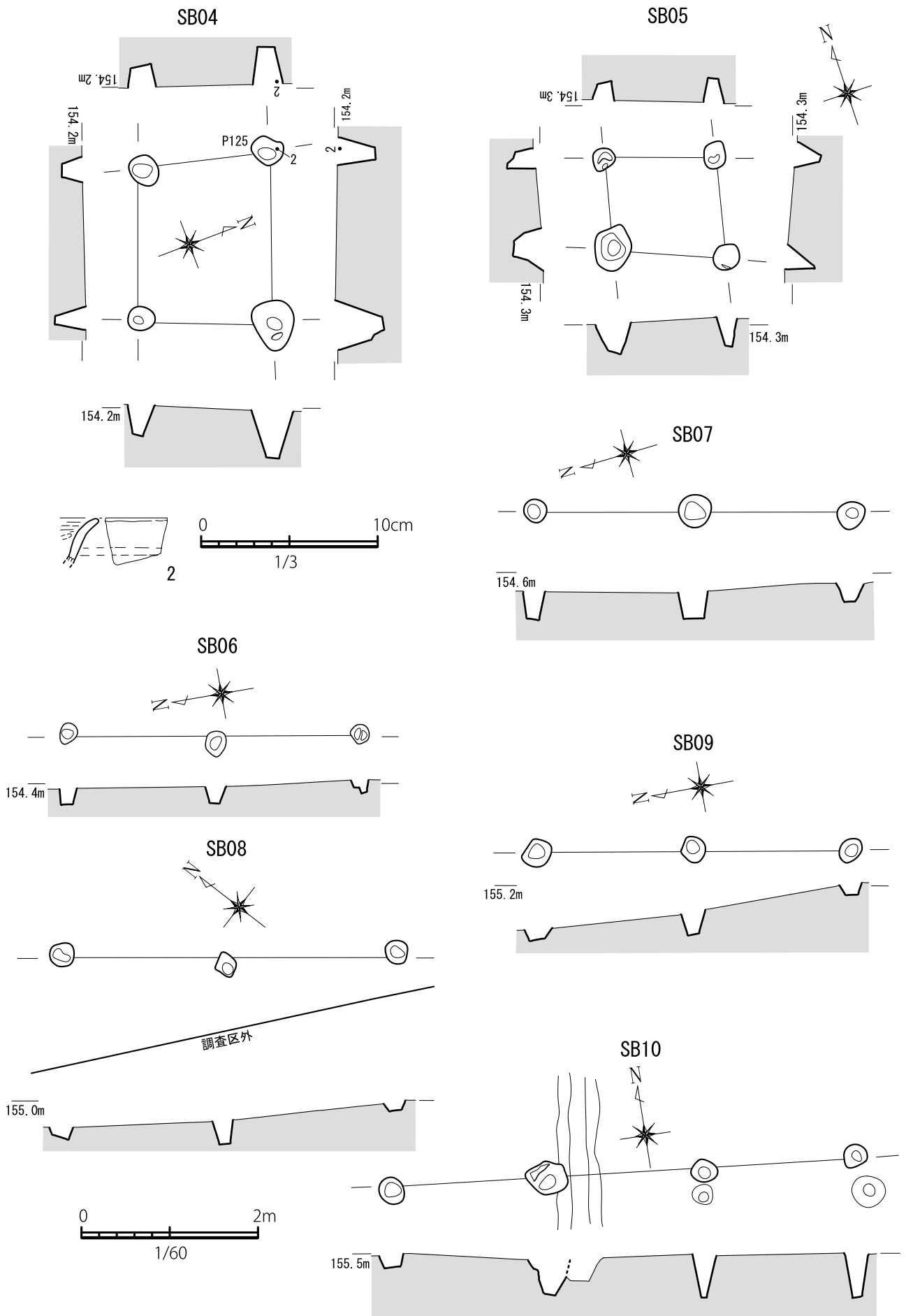
第8図 SB04~10実測図 (S=1/60) ・SB04出土遺物実測図 (S=1/3)
