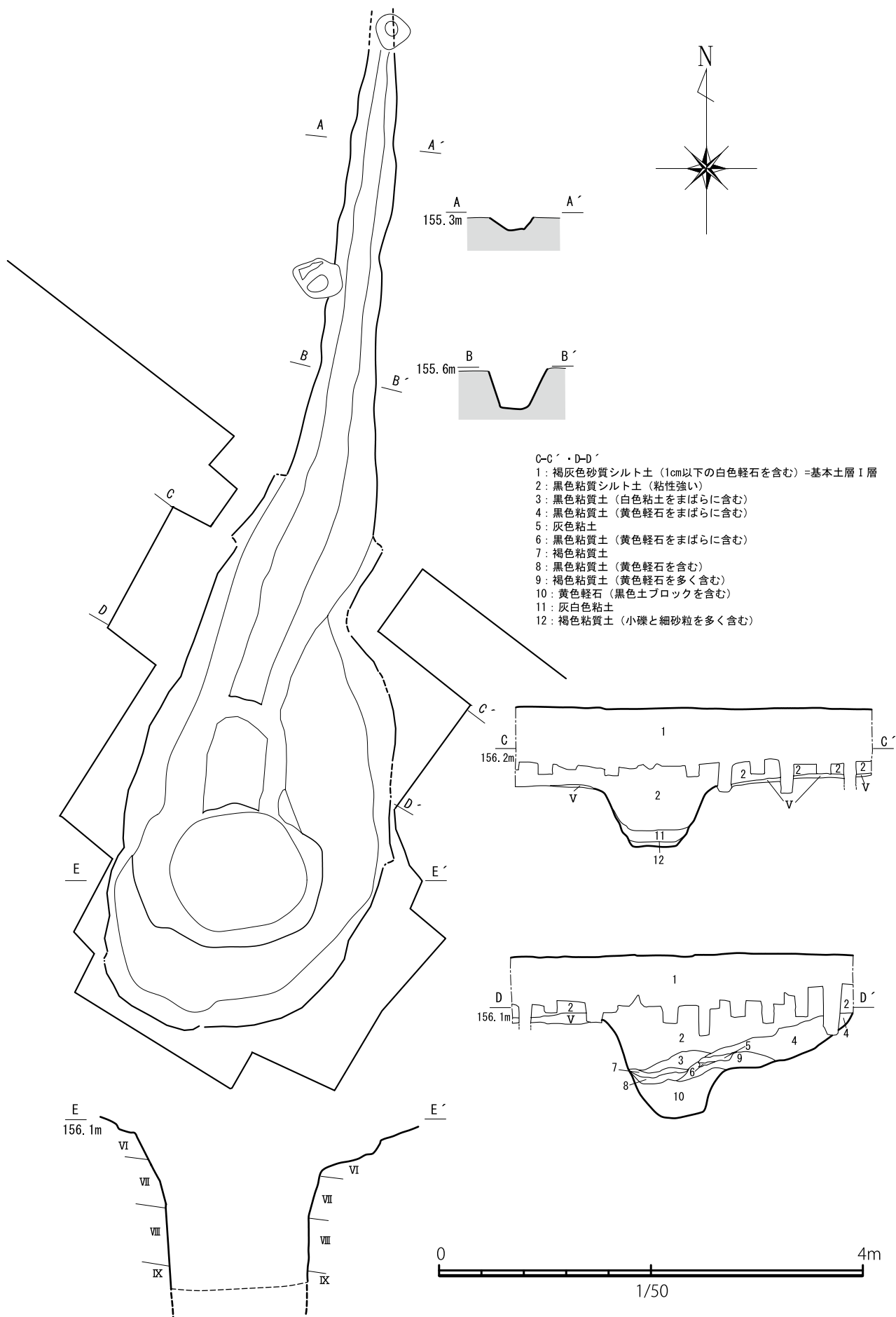
第13図 SD03実測図 (S=1/50)
