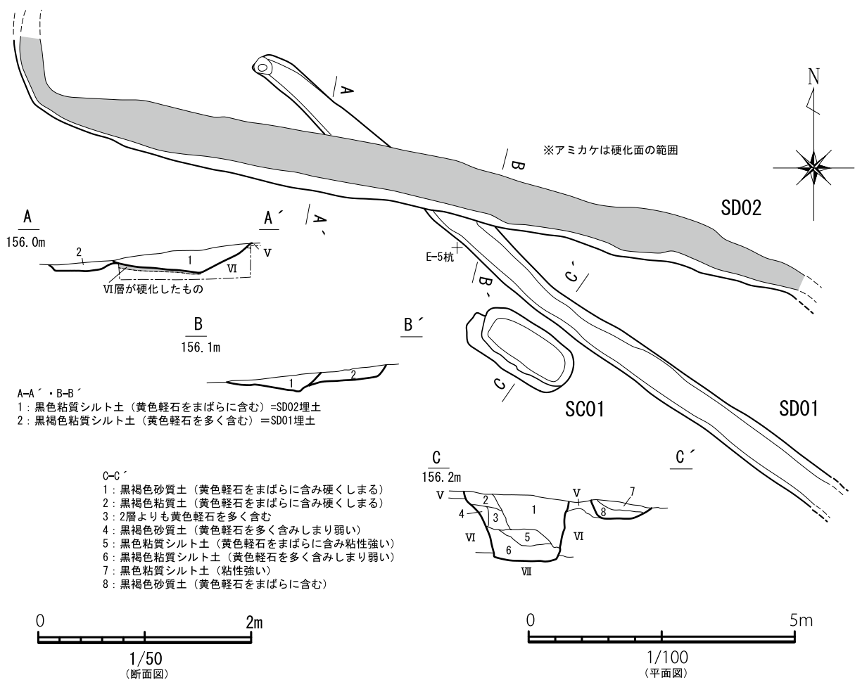
第11図 SD01・02・SC01実測図 (平面図: S=1/100、断面図: S=1/50)
