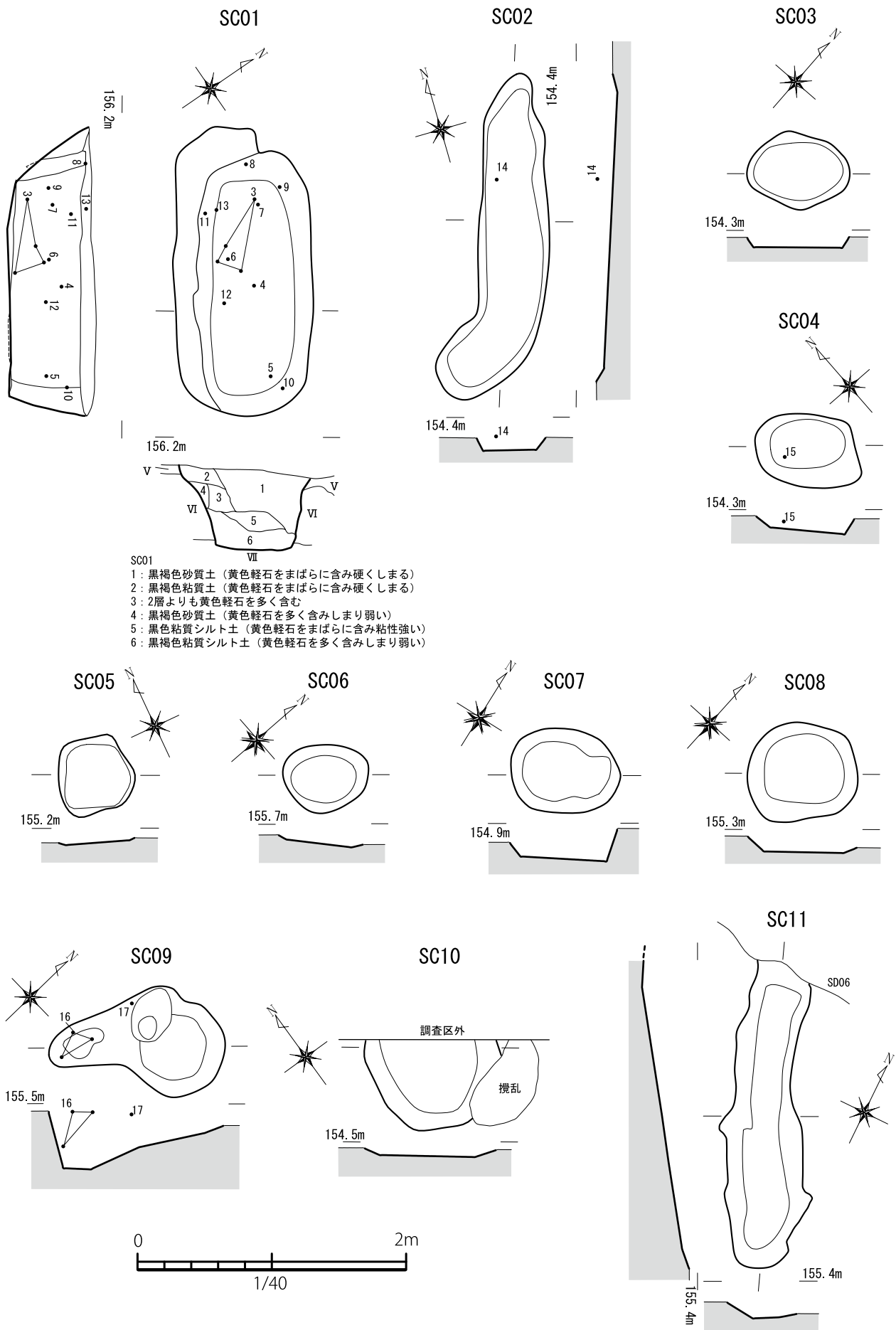
第9図 SC01~11実測図 (S=1/40)
