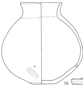
第4図 出土遺物実測図 (1) (1:4)
