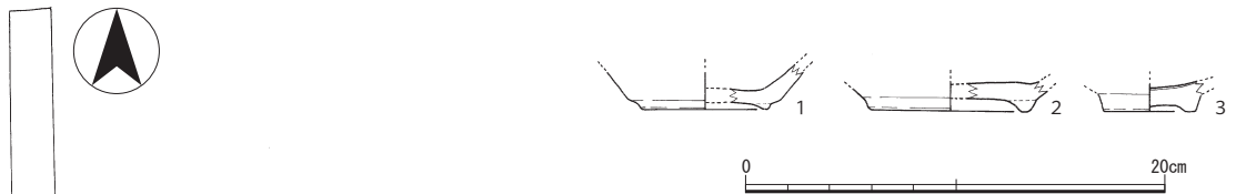
第2図 出土遺物実測図 (1:4)
