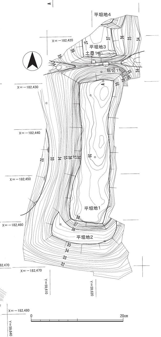
第5図 調査後地形測量図 (1:400)
