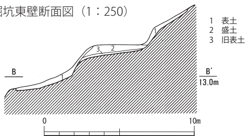
第5図 西試掘坑北壁断面図 (1:250)
