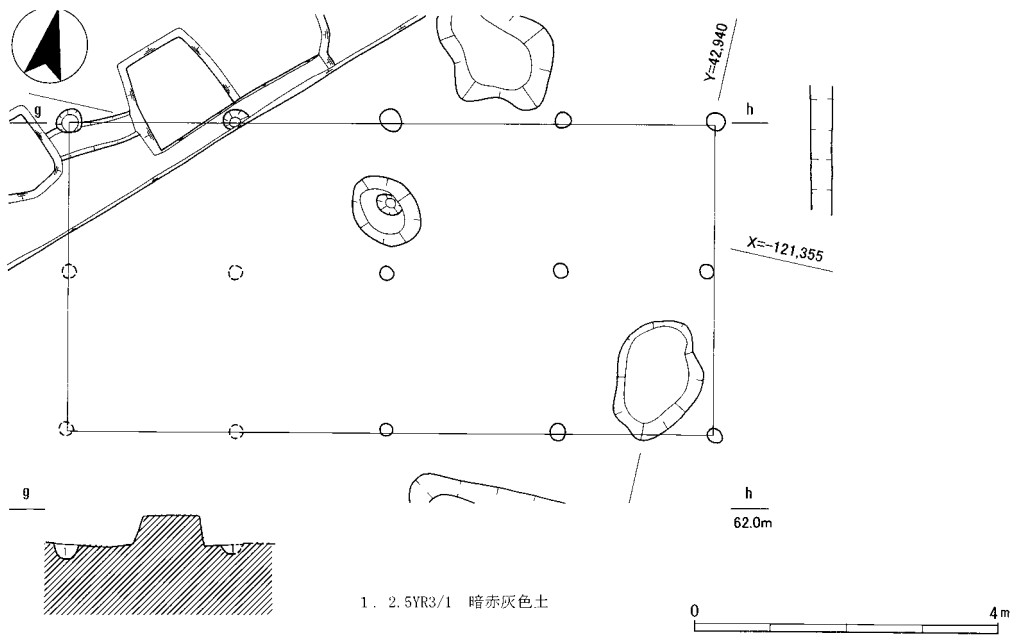
第10図 掘立柱建物SB42平面図、断面図 (1:100)
