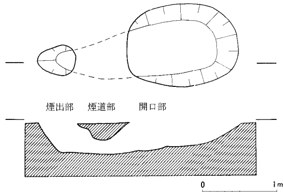
第21図 煙道付炉穴復元図 (1:50)
