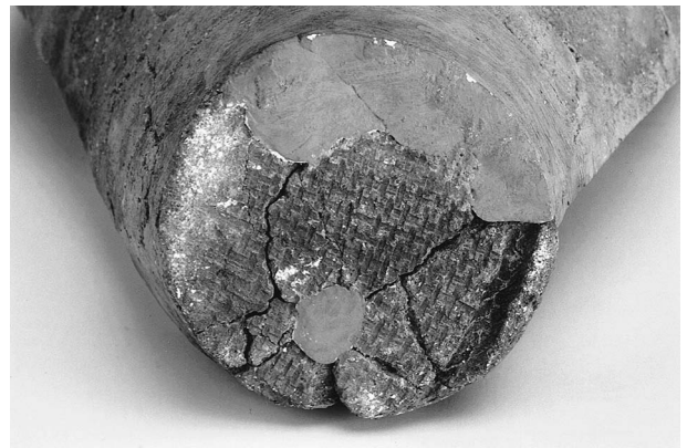
42底部
