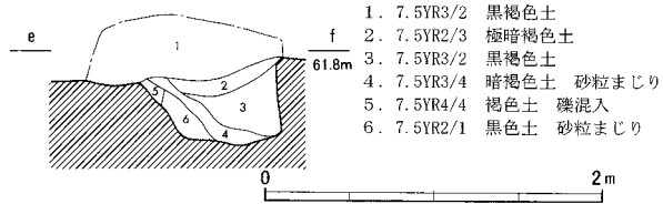
第7図 土坑SK22・26平面図、断面図 (1:50)
