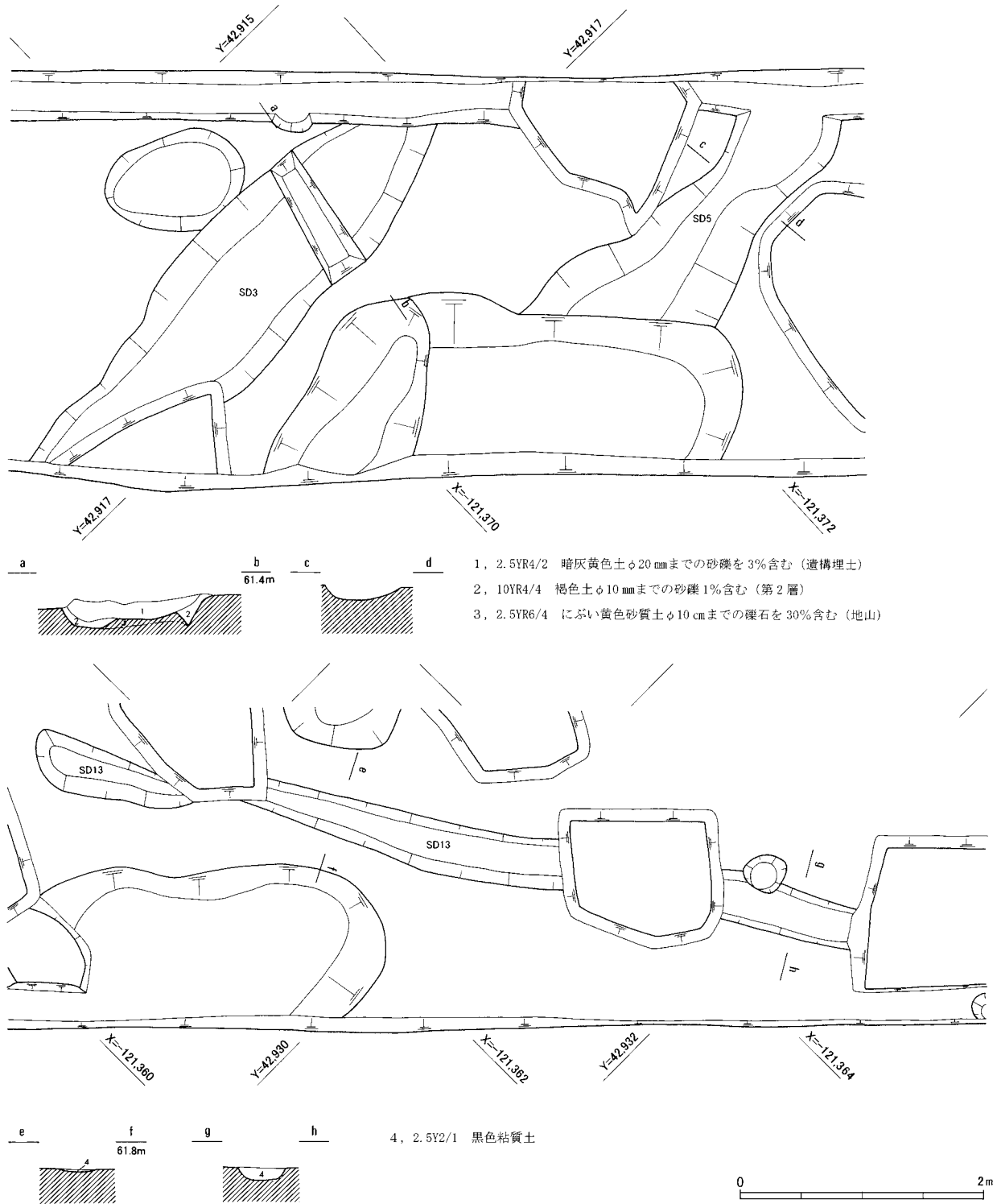
第11図 溝SD3・5・13平面図、断面図（1：50）
