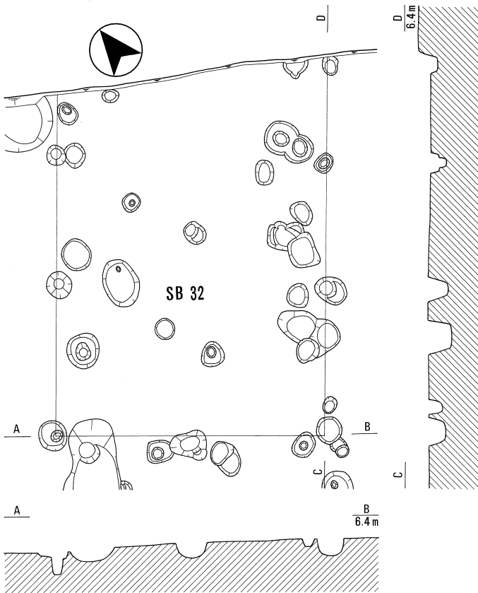
第6図 平安時代後期 掘立柱建物① SB31・32・33・36・37 1:100
