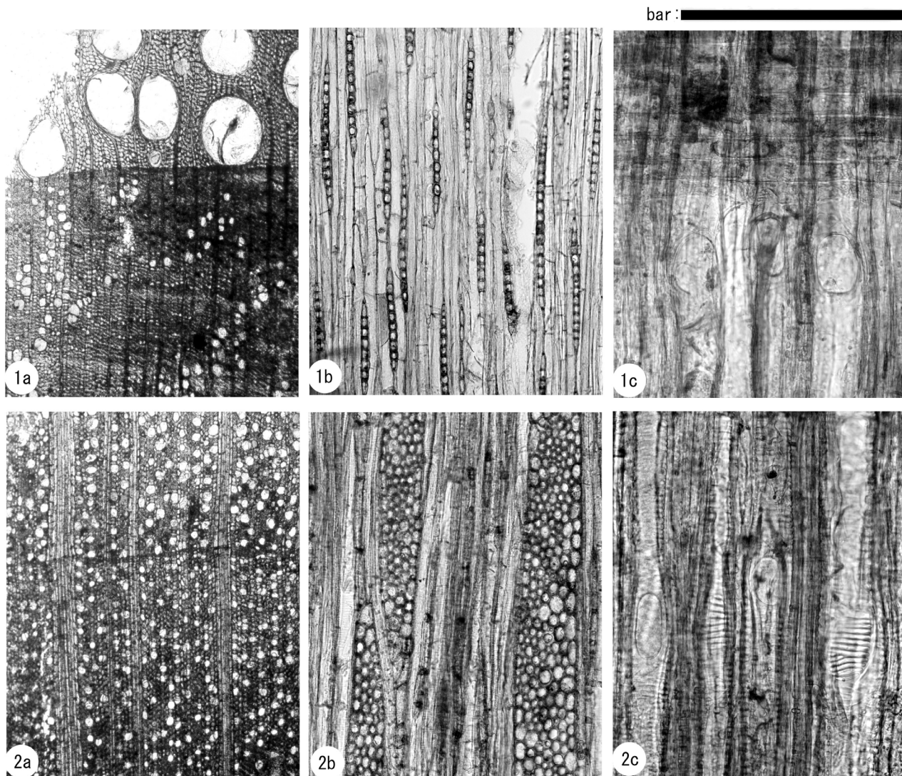
第9図 廿子遺跡出土柱根材組織の光学顕微鏡写真
