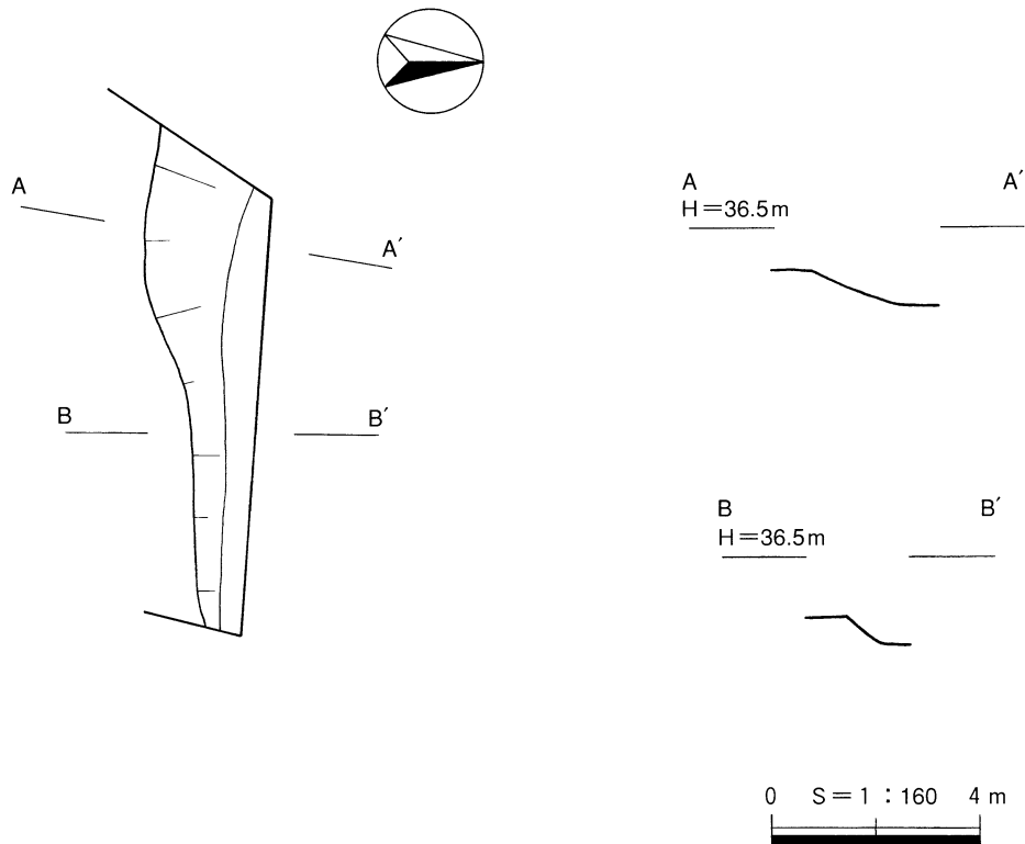
第8図 SD-02遺構図
