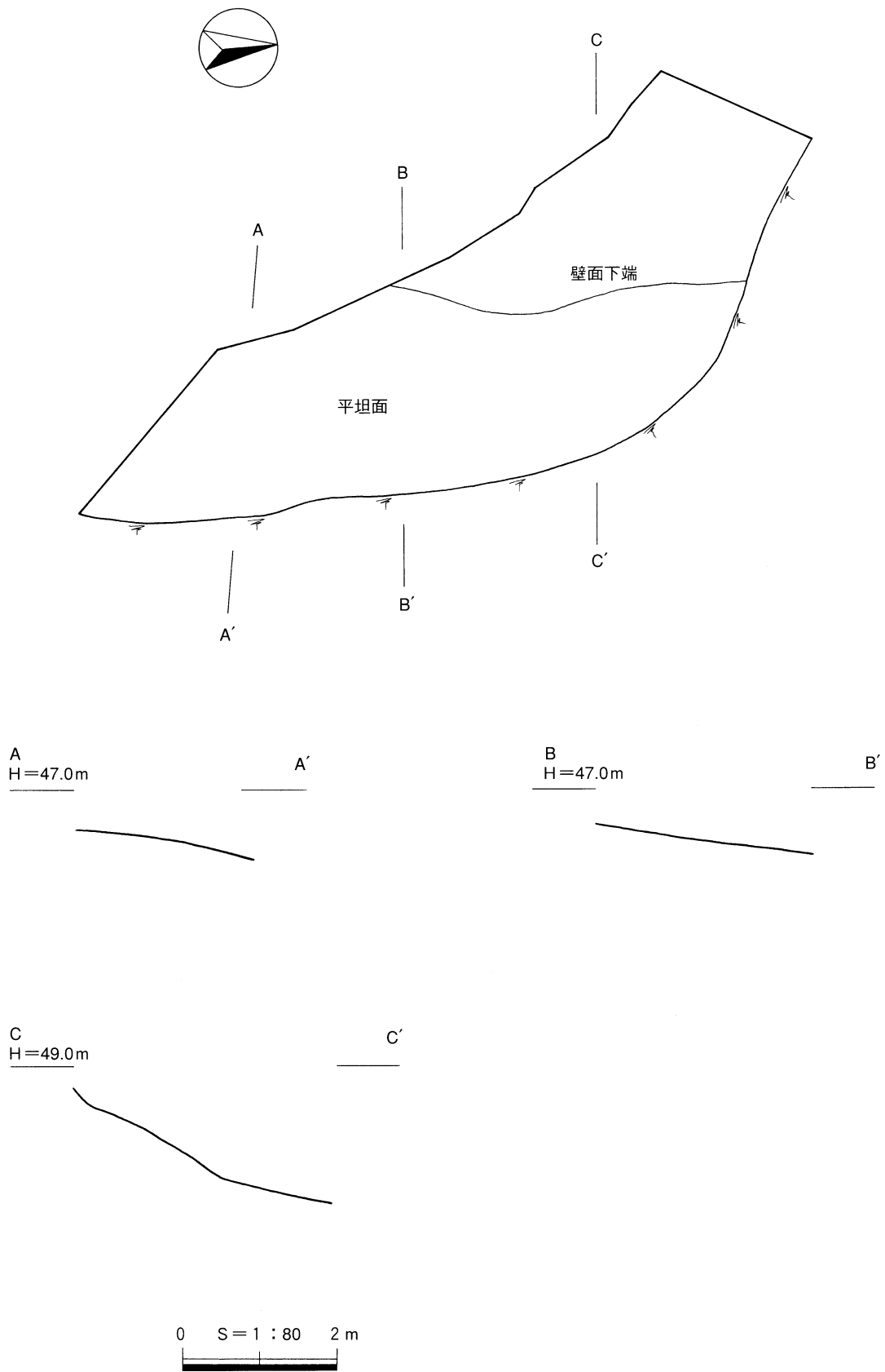
第11図 SS-01遺構図
