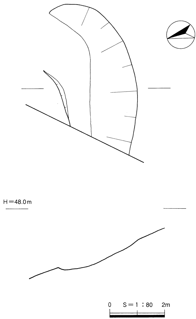
第5図 SD-01遺構図
