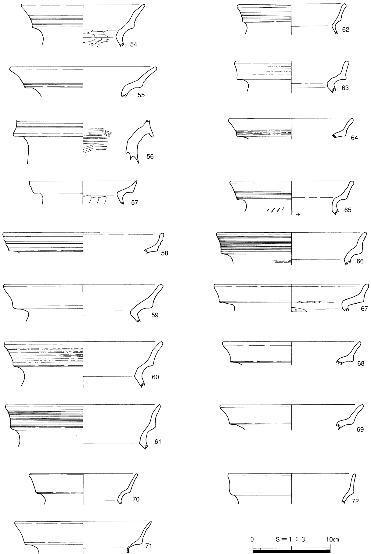
第12図 SS-01出土遺物実測図(1)
