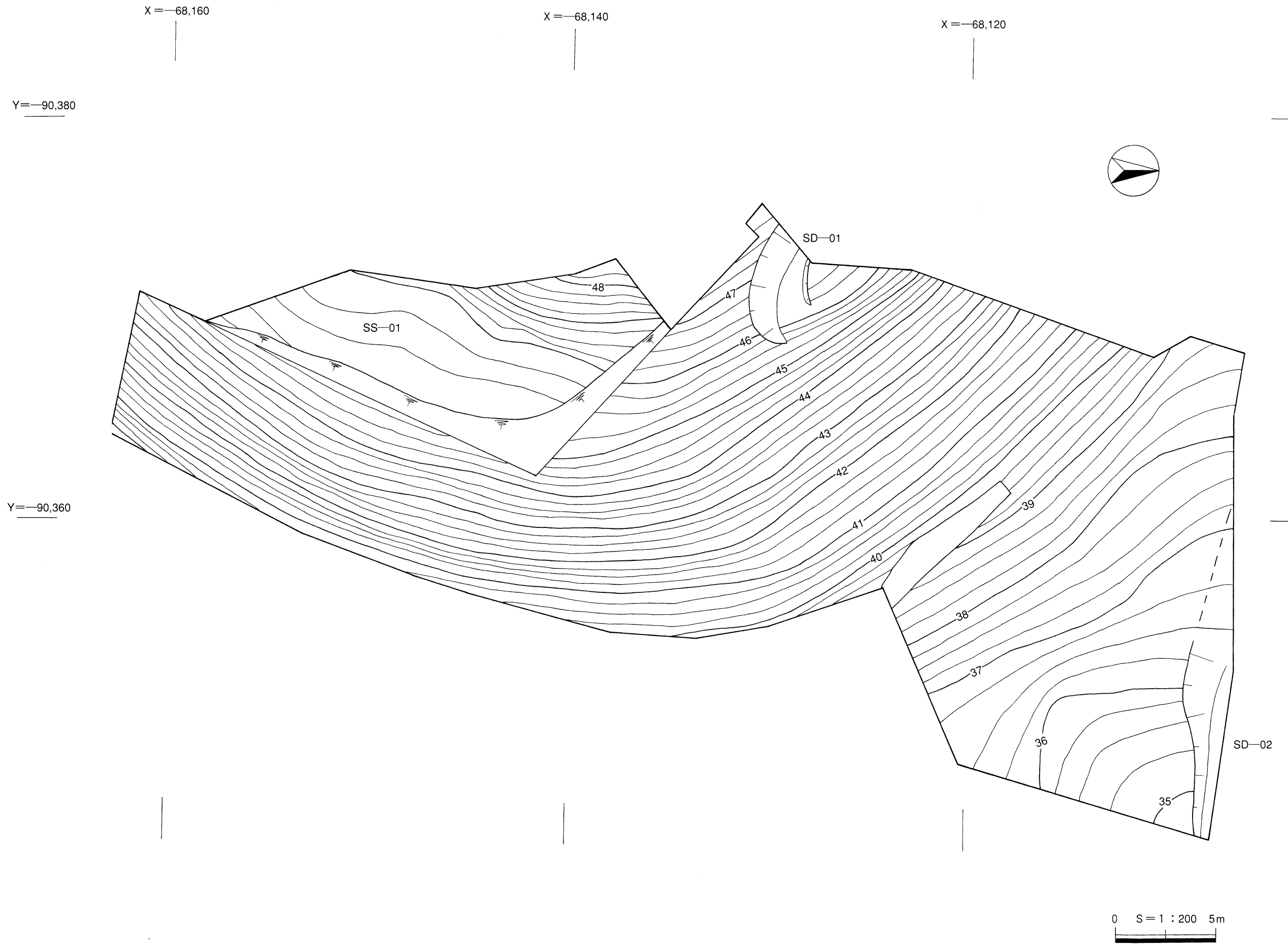
第4図 遺構配置図
