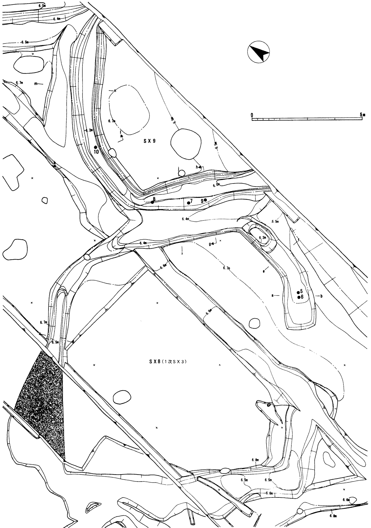
第9图 SX 8·9平面图 (S=1:100)
