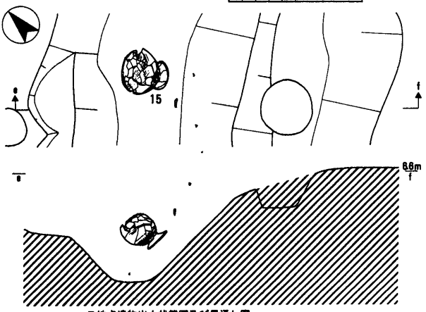
B地点遺物出土状態図及び見通し図
