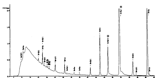
第16図 赤色物質付着壺片の元素定性スペクトル
