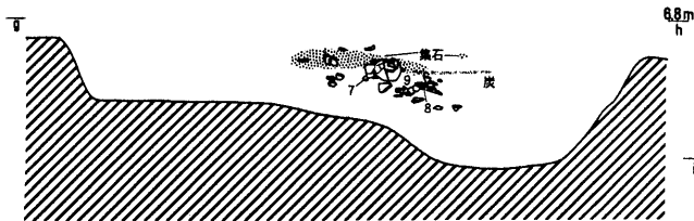
B地点遺物出土状態図及び見通し図
