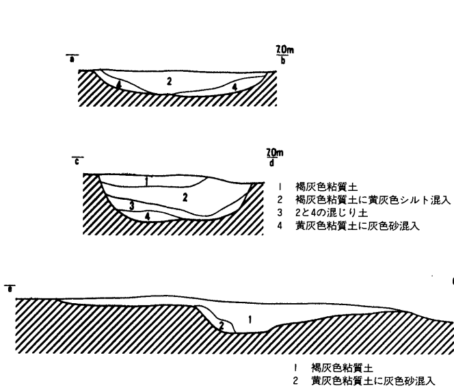
第8図 SX6・7平面図 (S=1:100) 及び土層断面図・SX7遺物出土状態図 (S=1:40)
