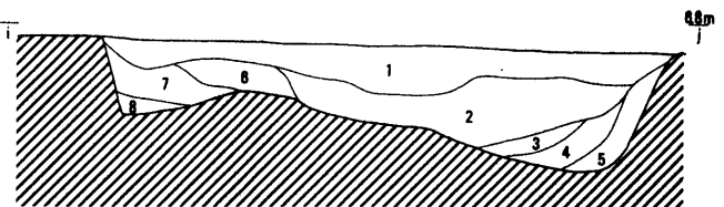
第10図 S X 8・9遺物出土状態図及び土層断面図・見通し図 (S=1:40)
