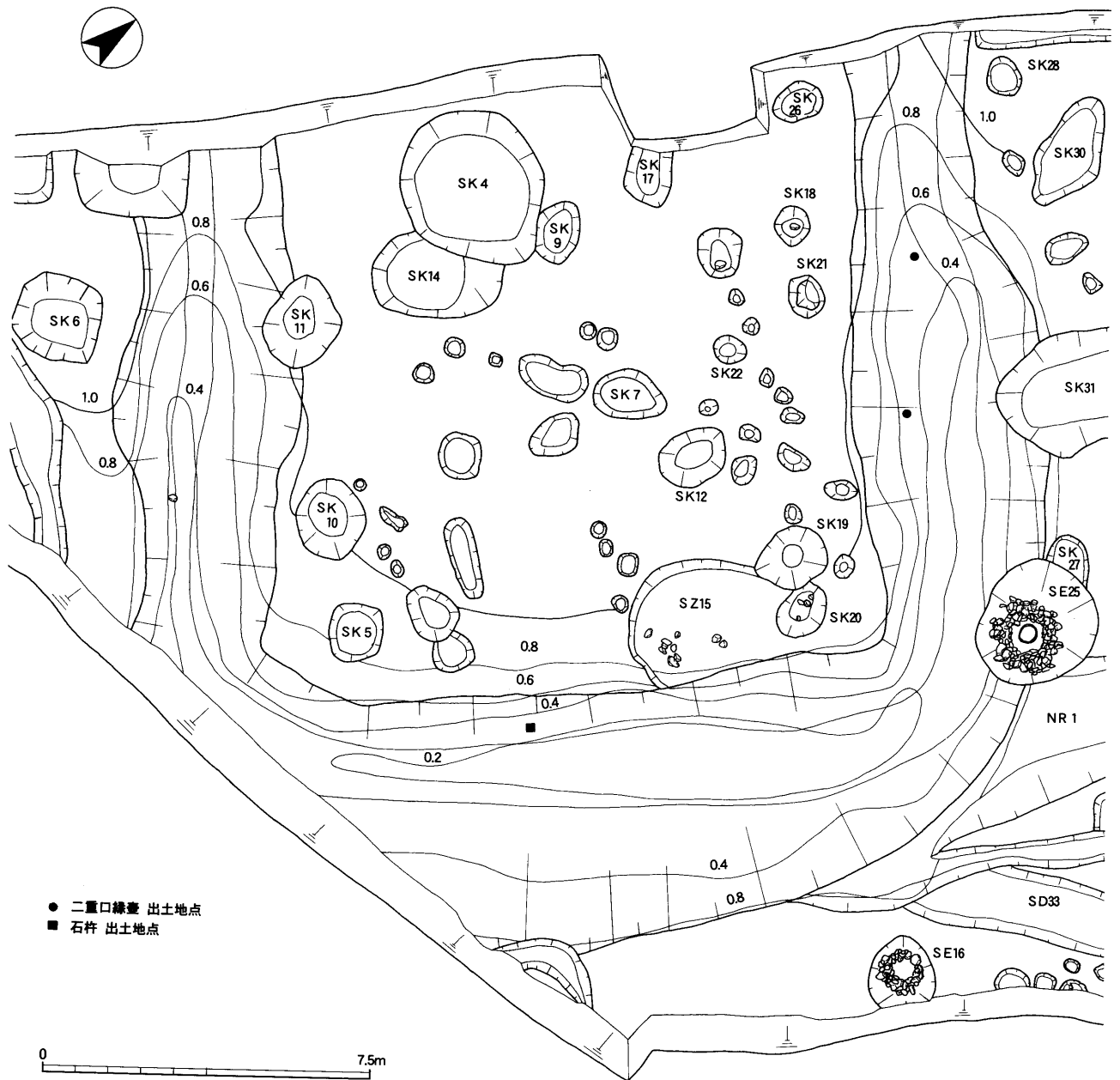
第6図 SX3 (前田町屋1号墳) 実測図 (1:150)
