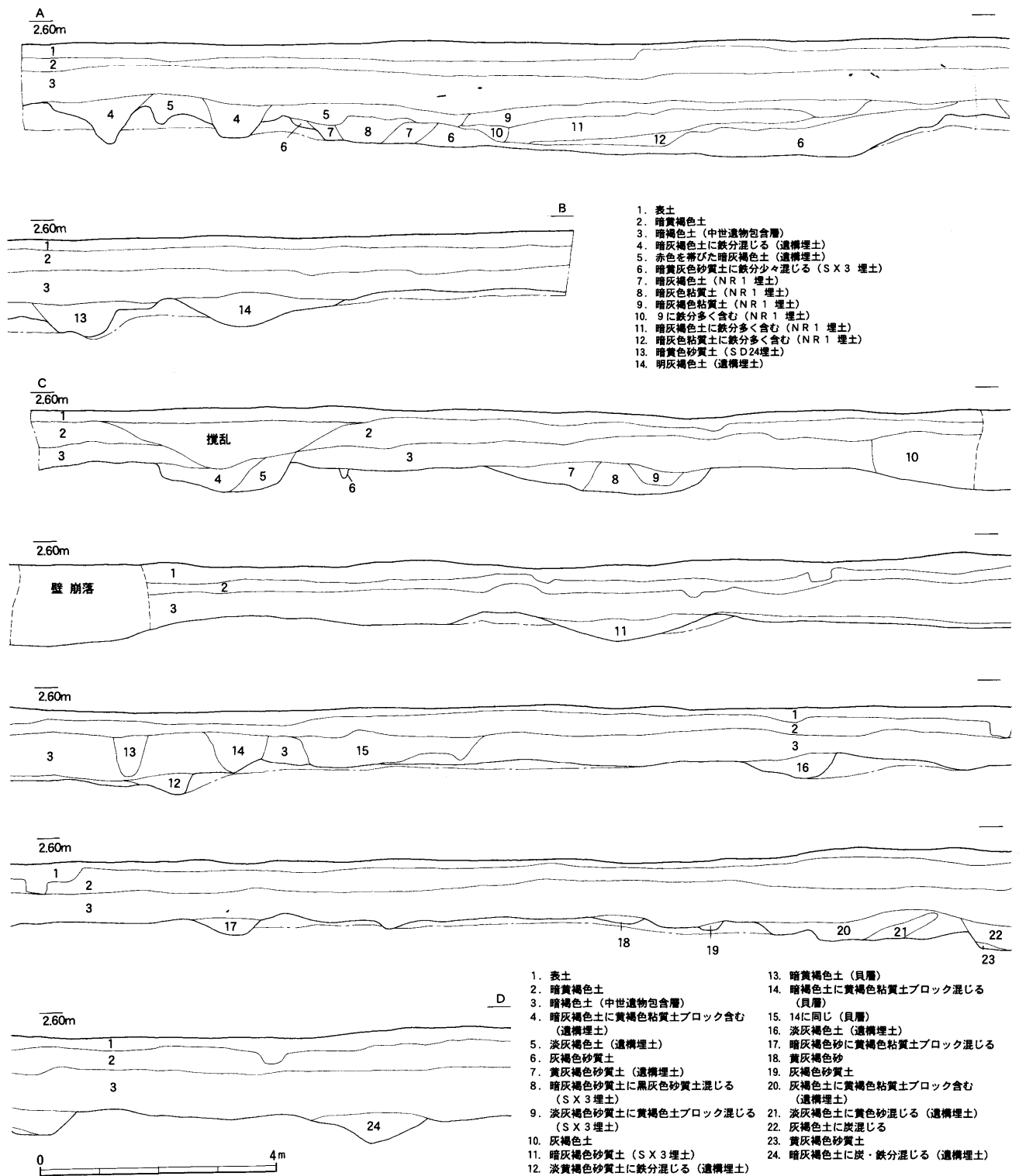
第5図 調査区 南壁・東壁 土層断面図 (1:100)
