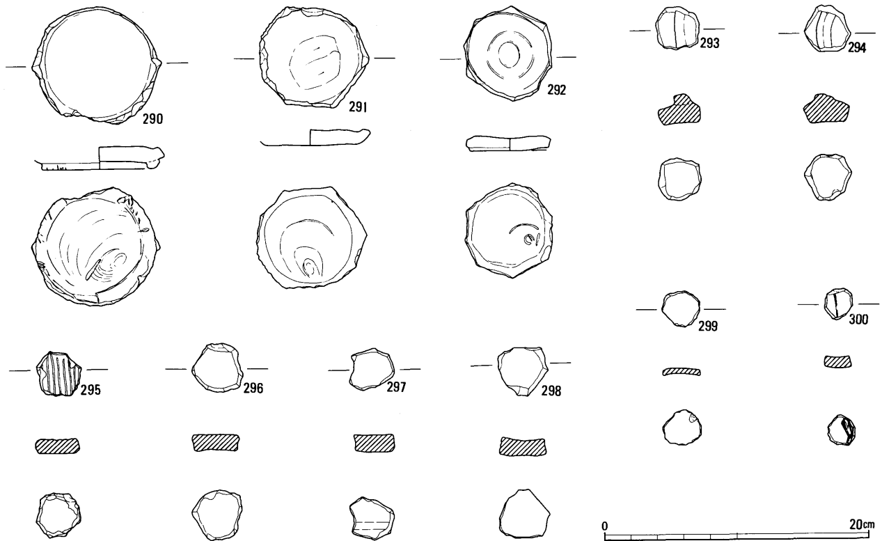
第19図 出土加工円盤 実測図 (1 : 4)
