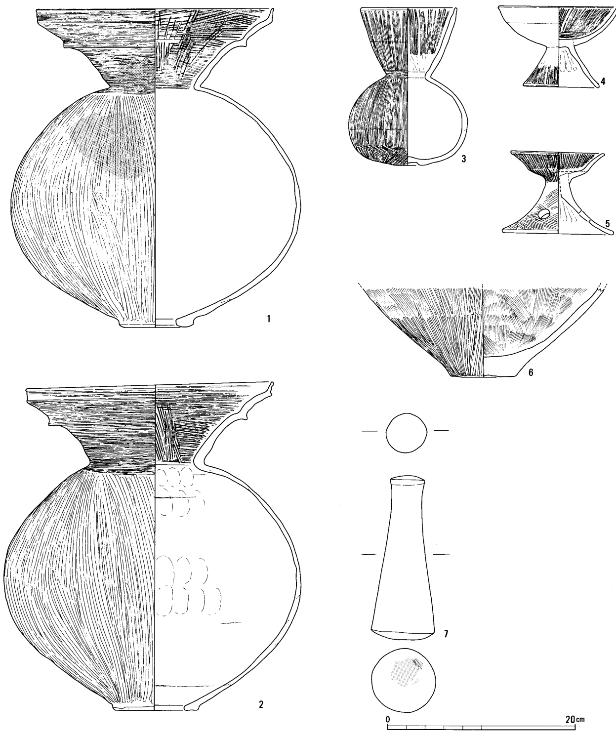
第9図 出土遺物実測図(1) (1:4) SX3
