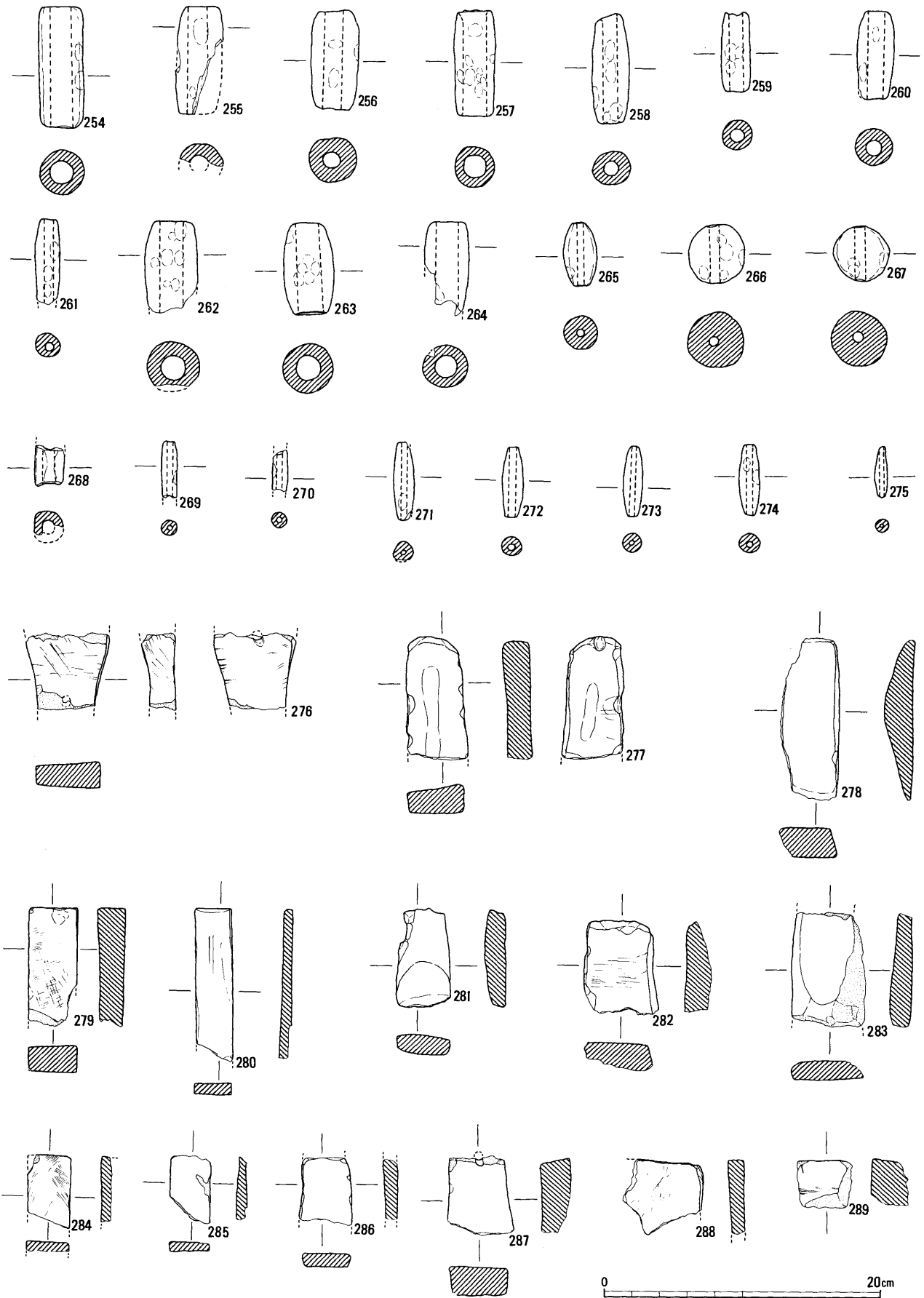
第18図 出土土錘・砥石 実測図 (1 : 4)
