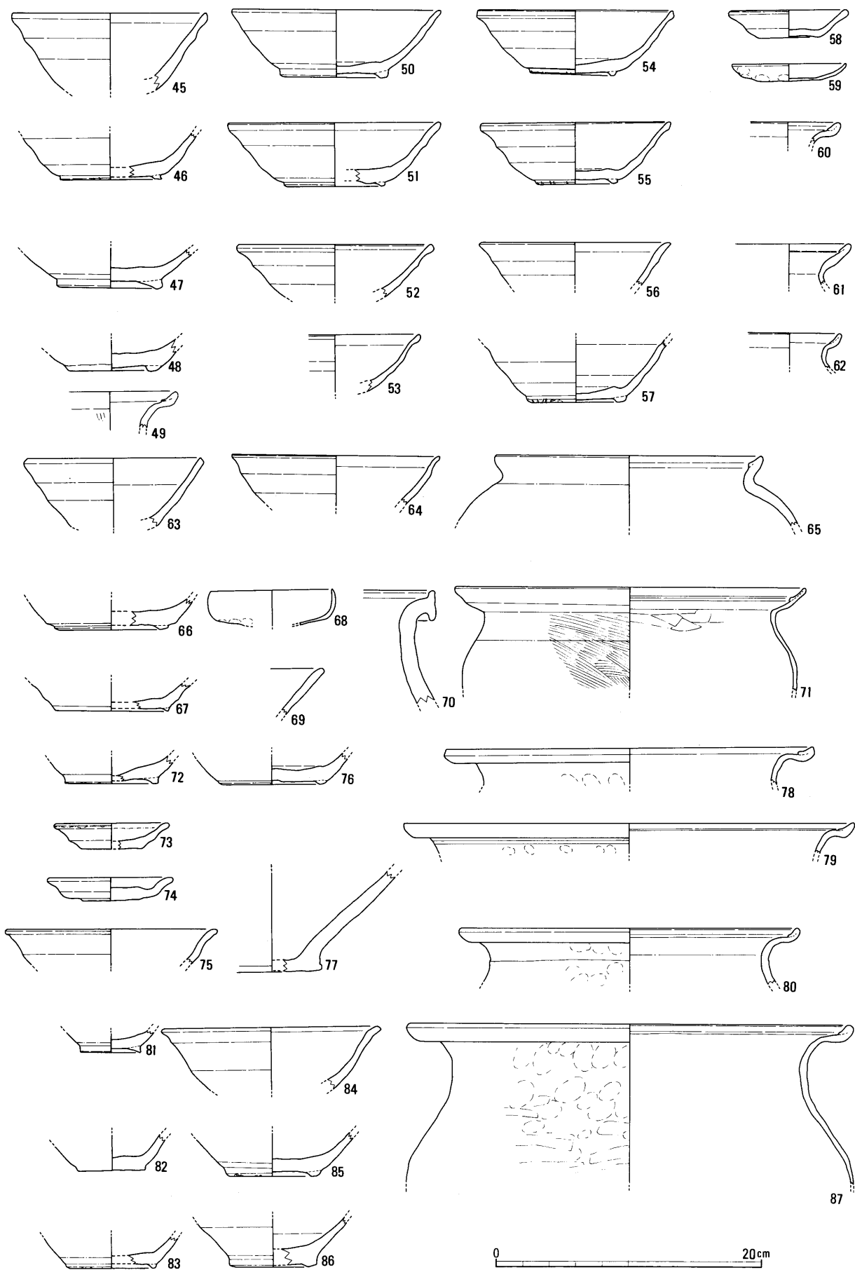
第11図 出土遺物実測図(3) (1:4) S K 14・30・32・34・43・47・54・56~58・60・64・72
