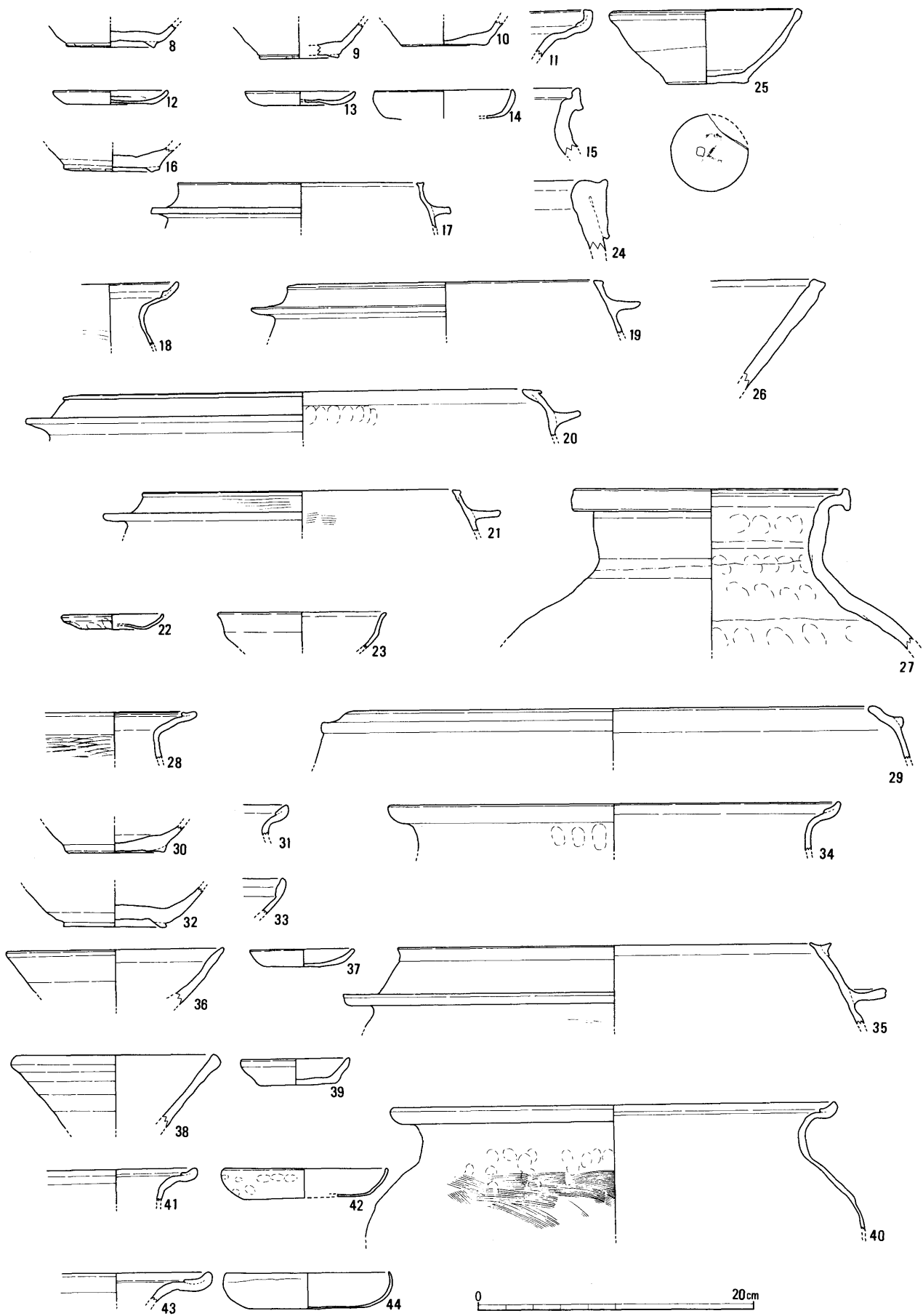
第10图 出土遺物実測図(2)(1:4) S E 31・25・82・S K 4・11・12・13・16・23
