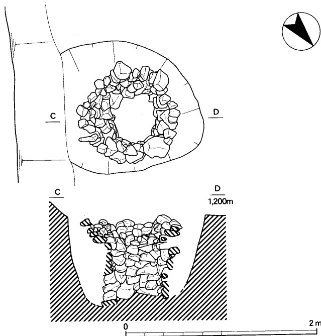
第8図 S E 16 実測図(1:40)
