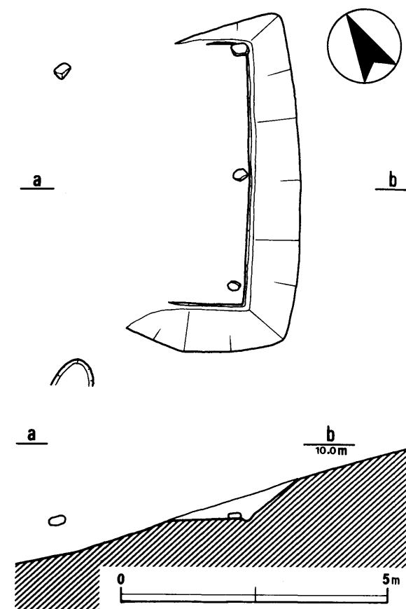
第8図 SB1平面図・立面図(1:100)
