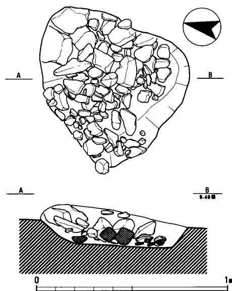
第7図 集石遺構平面図・立面図(1:20)
