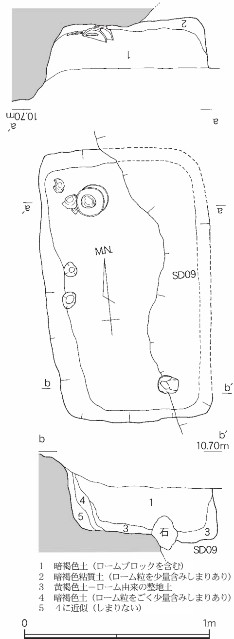
Fig.34 SR56平面図・断面図 (S=1/20)
