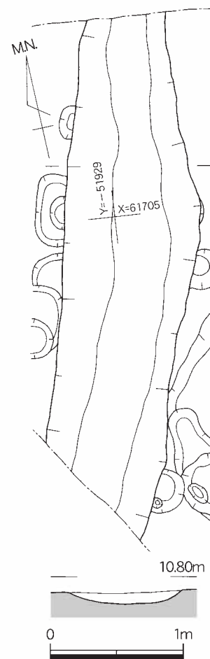
Fig.38 SD05 平面図・断面図 (S=1/40)
