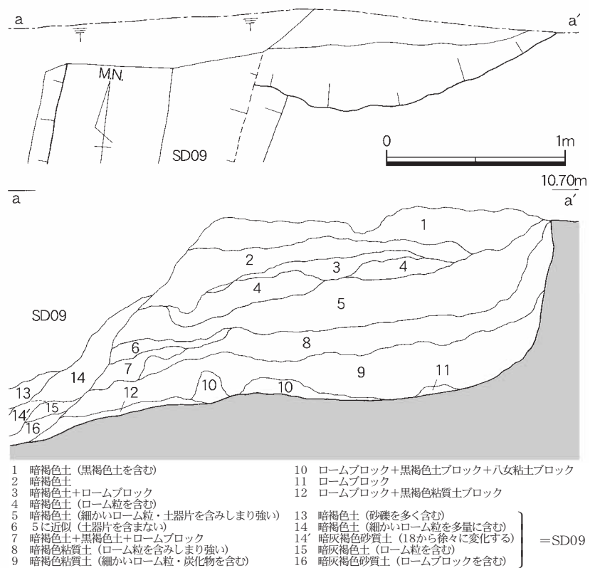
Fig.24 SX63平面図・断面図 (S=1/30)
