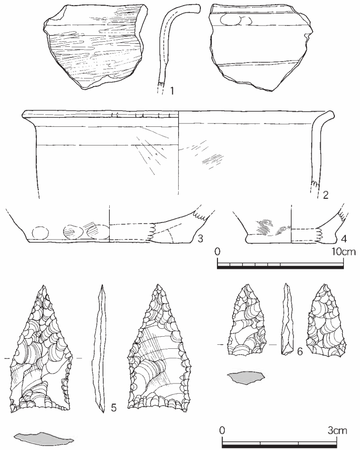
Fig.7 SK01出土遺物実測図 (S=1/1・1/3)
