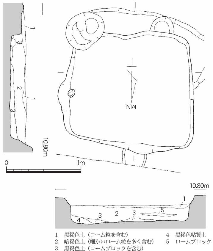
Fig.6 SK01平面図・断面図 (S=1/30)
