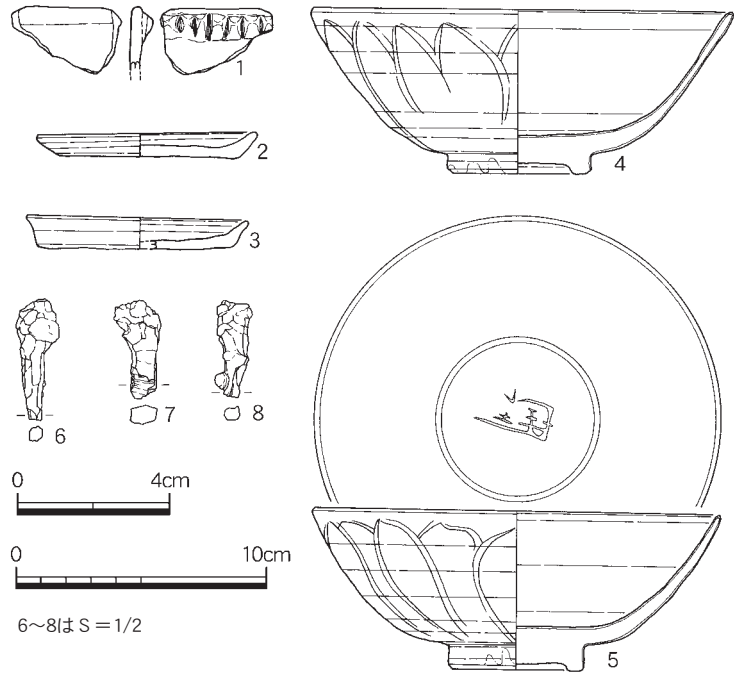
Fig.35 SR56出土遺物実測図 (S=1/2・1/3)
