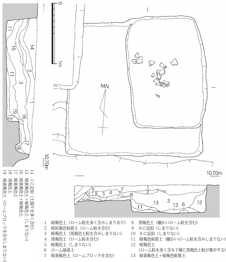
Fig.14 SK04平面図・断面図 (S=1/30)
