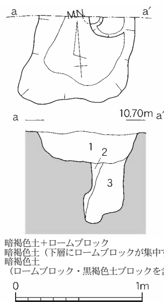
Fig.22 SP96平面図・断面図 (S=1/30)
