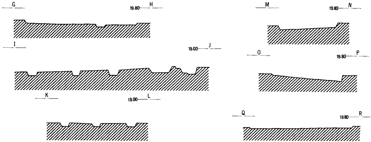
第15図 SB 6・8～10・13・14実測図（1：100）
