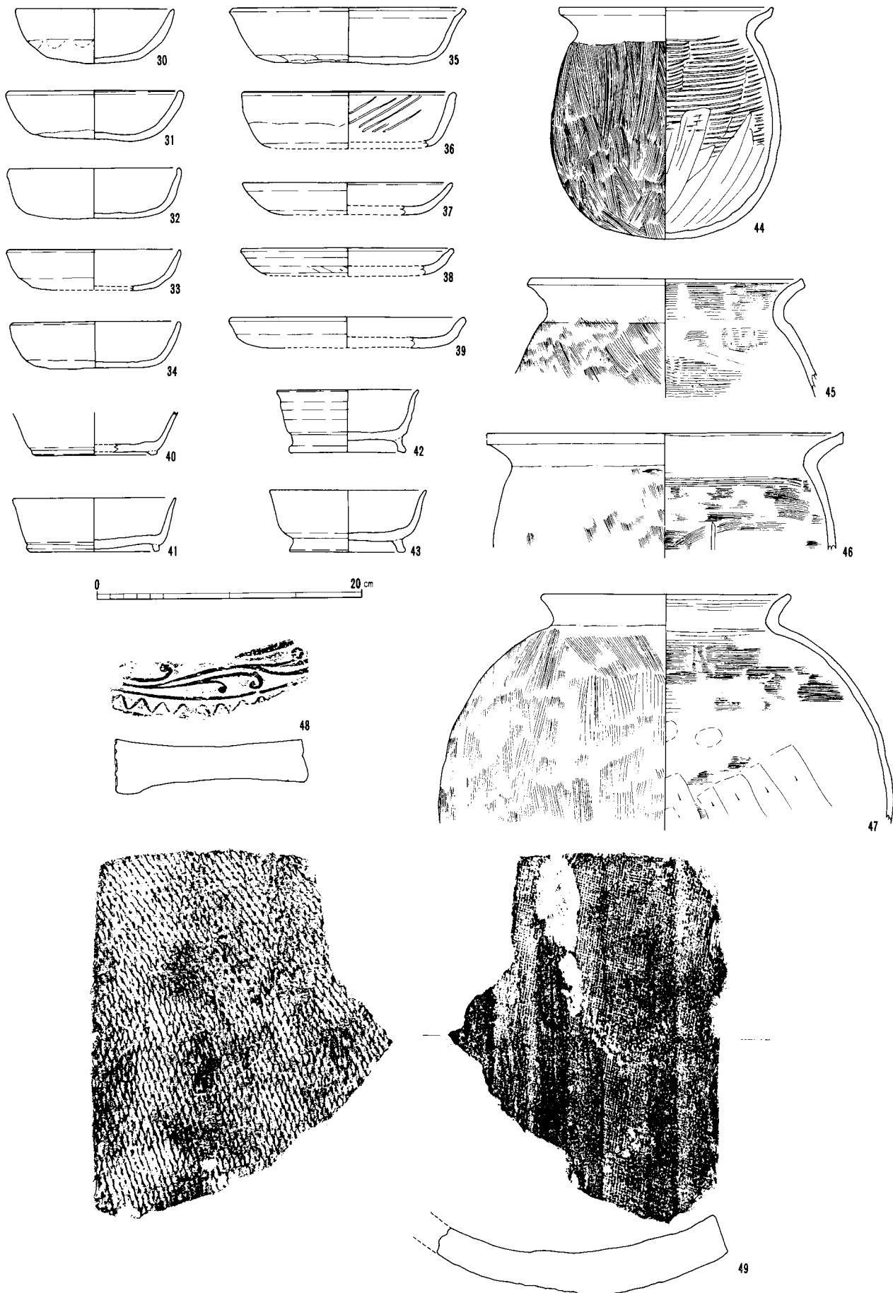
第18図 SB 8 出土遺物実測図 (1 : 4) (49は 1 : 3)
