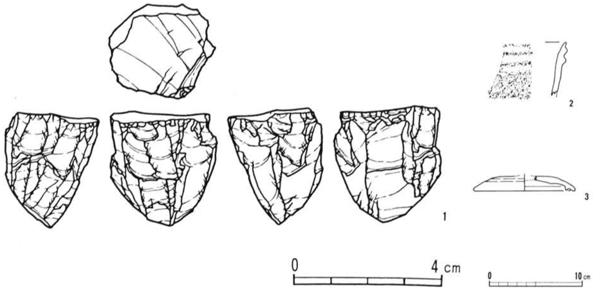
第26図 出土遺物実測図（1は1：1，2・3は1：4）
