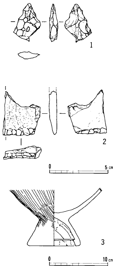
第22図 遺物実測図 (1・2…1:2, 3…1:4)
