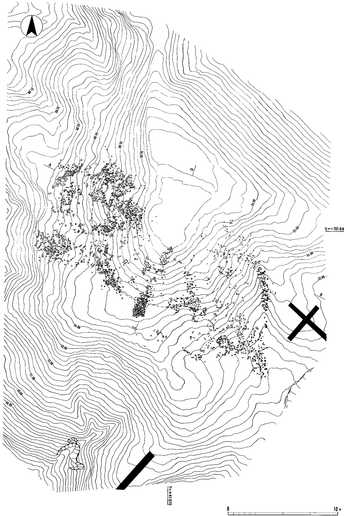
第5図 調査区平面図 (1:200)
