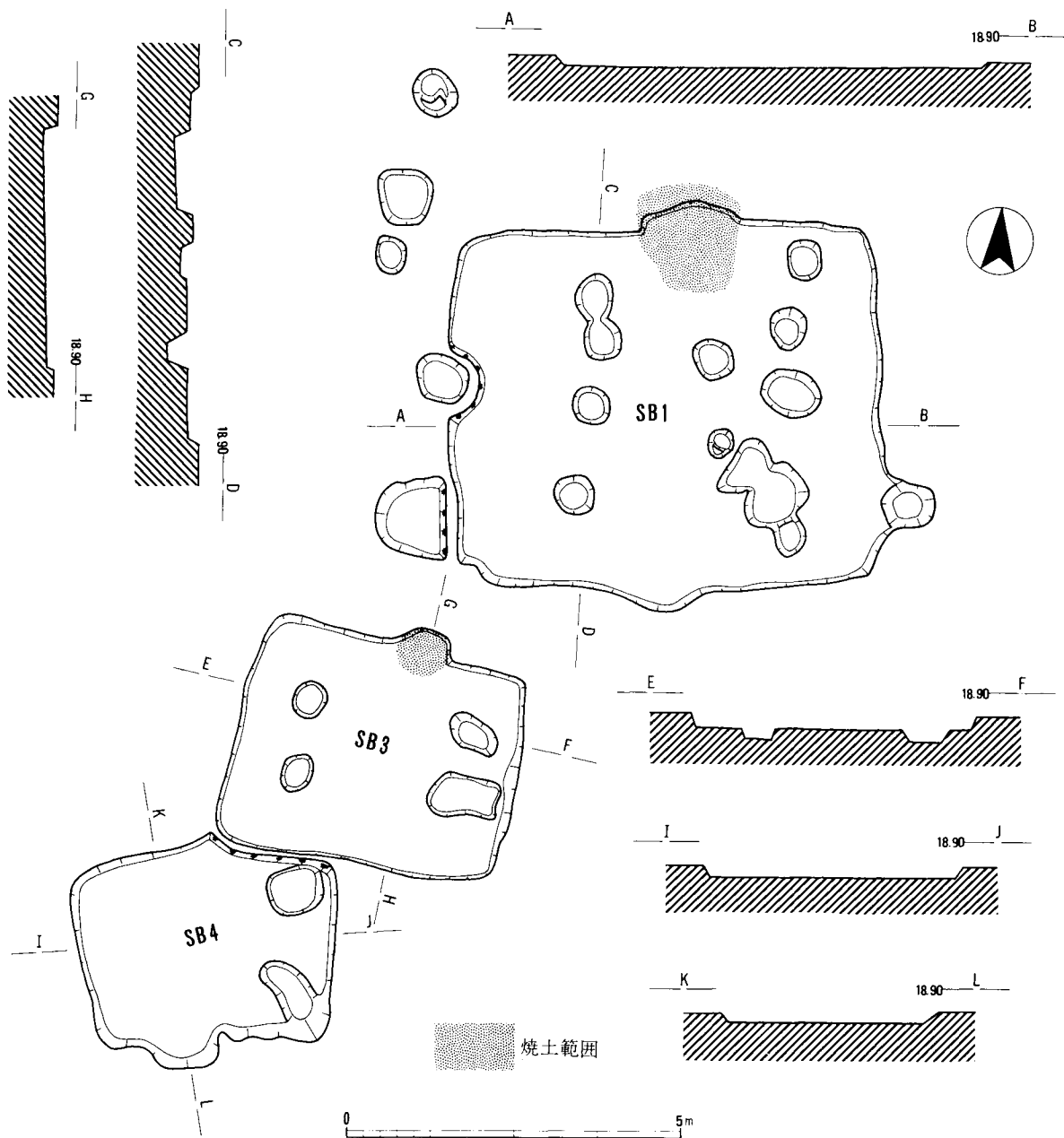
第12図 SB1・3・4実測図(1:100)
