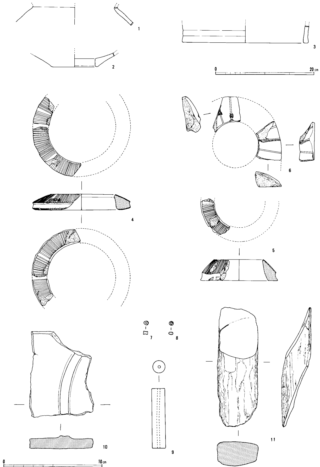
第7図 出土遺物実測図（1～3は1：4，4～11は1：2）
