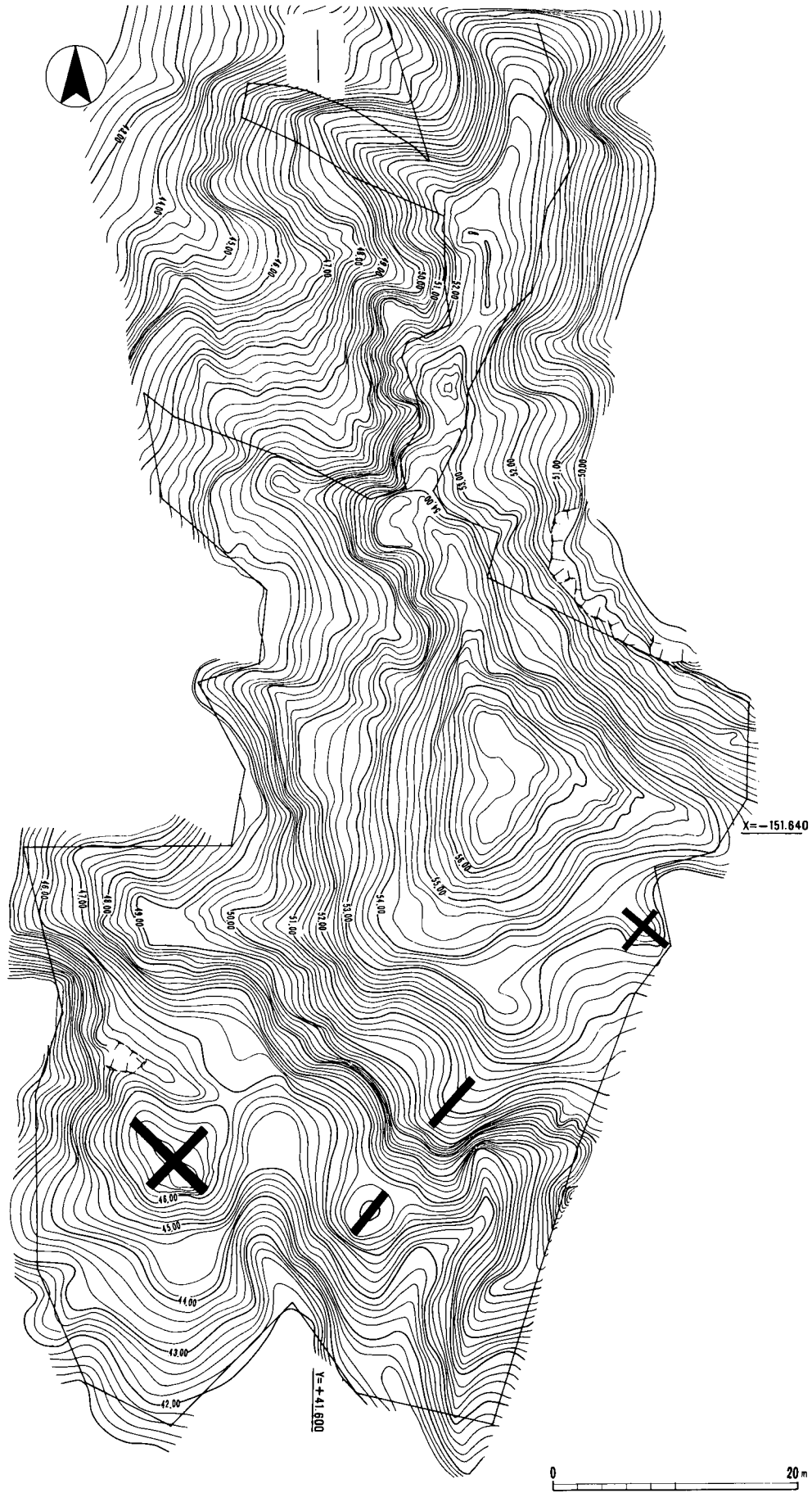
第4図 調査前測量図(1:500)
