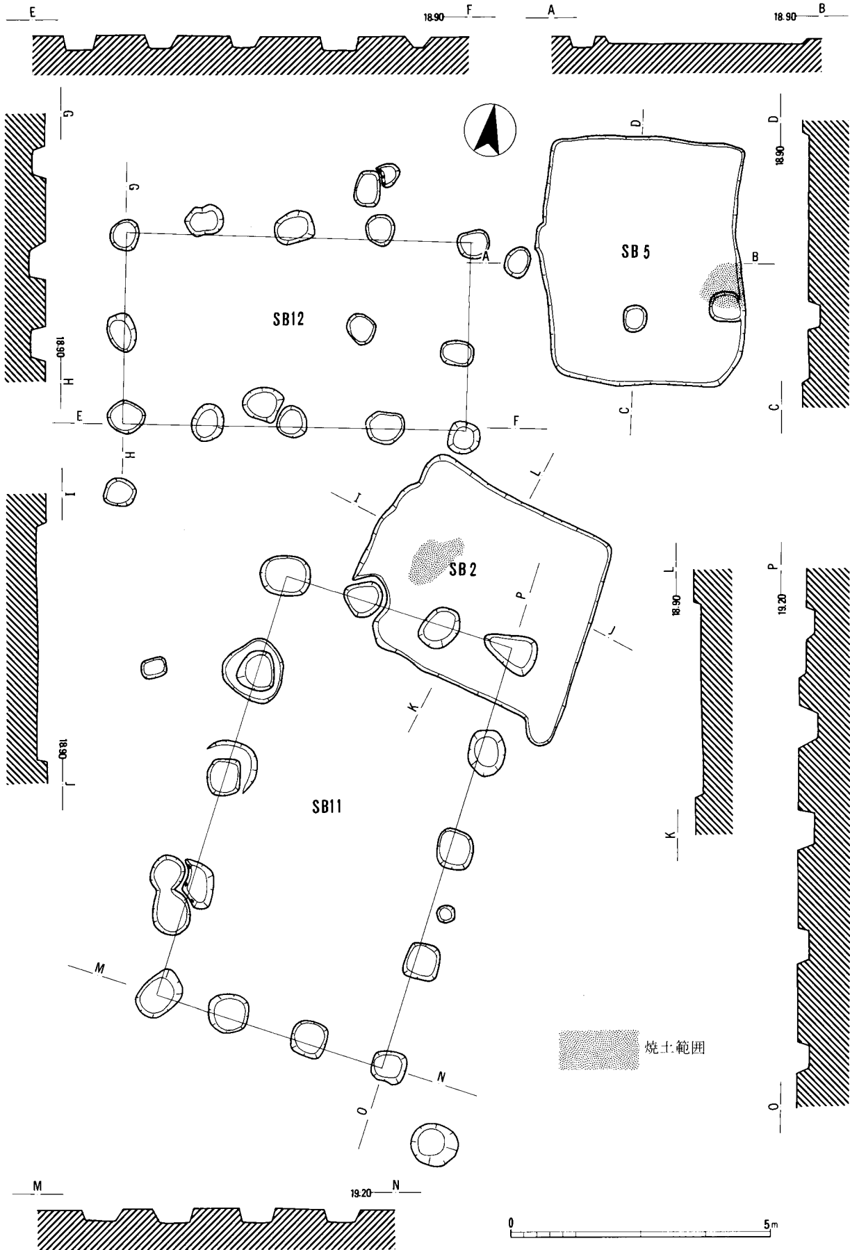
第13図 SB 2・5・11・12実測図 (1:100)
