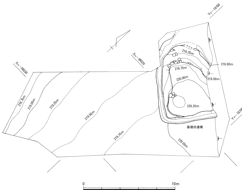
第9図 近世遺構配置図（1/200）
