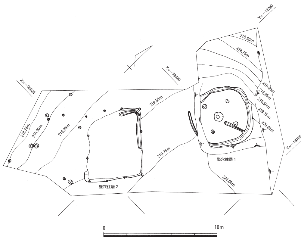
第5図 古墳時代遺構配置図 (1/200)
