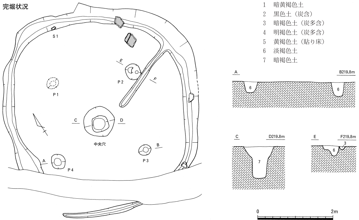
第6図 竪穴住居1 (1/60)・出土遺物 (1/4・1/3)
