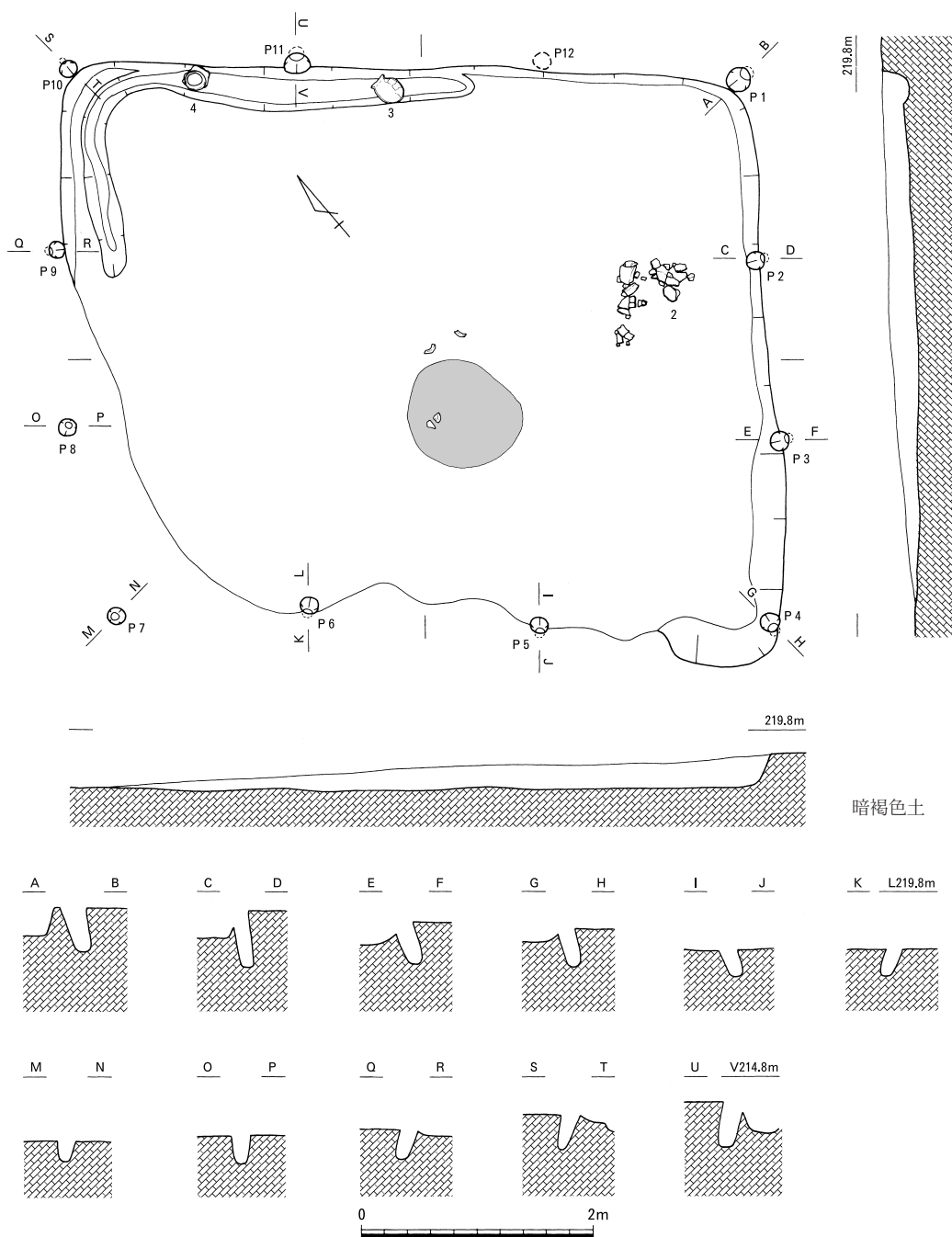
第7図 竪穴住居2 (1/60)
