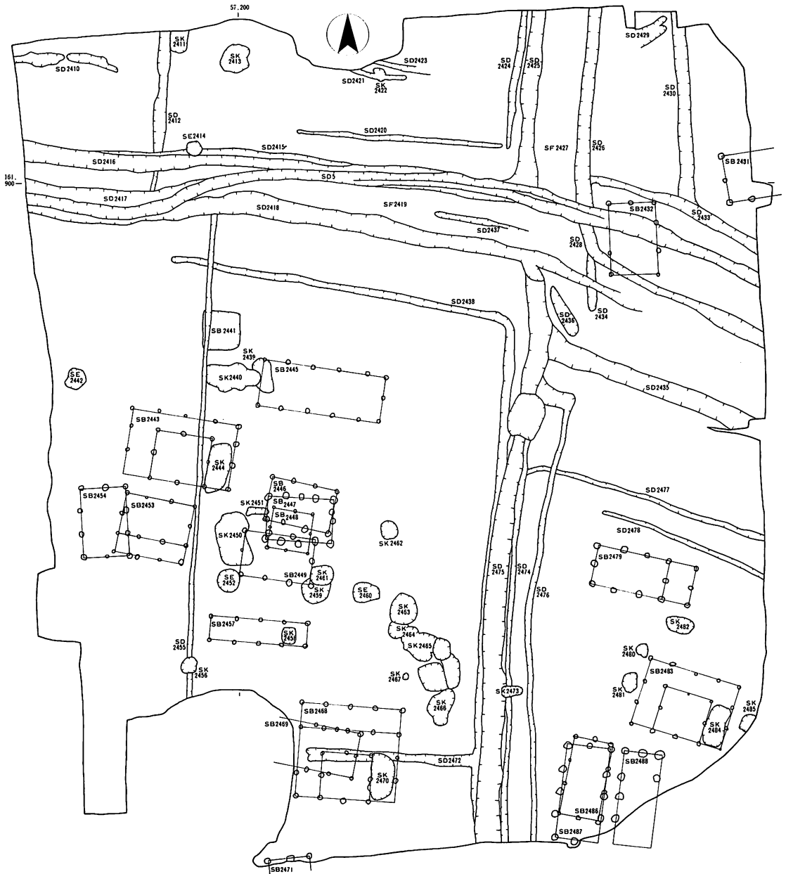
fig. 5 遺構配置図(1:500)
