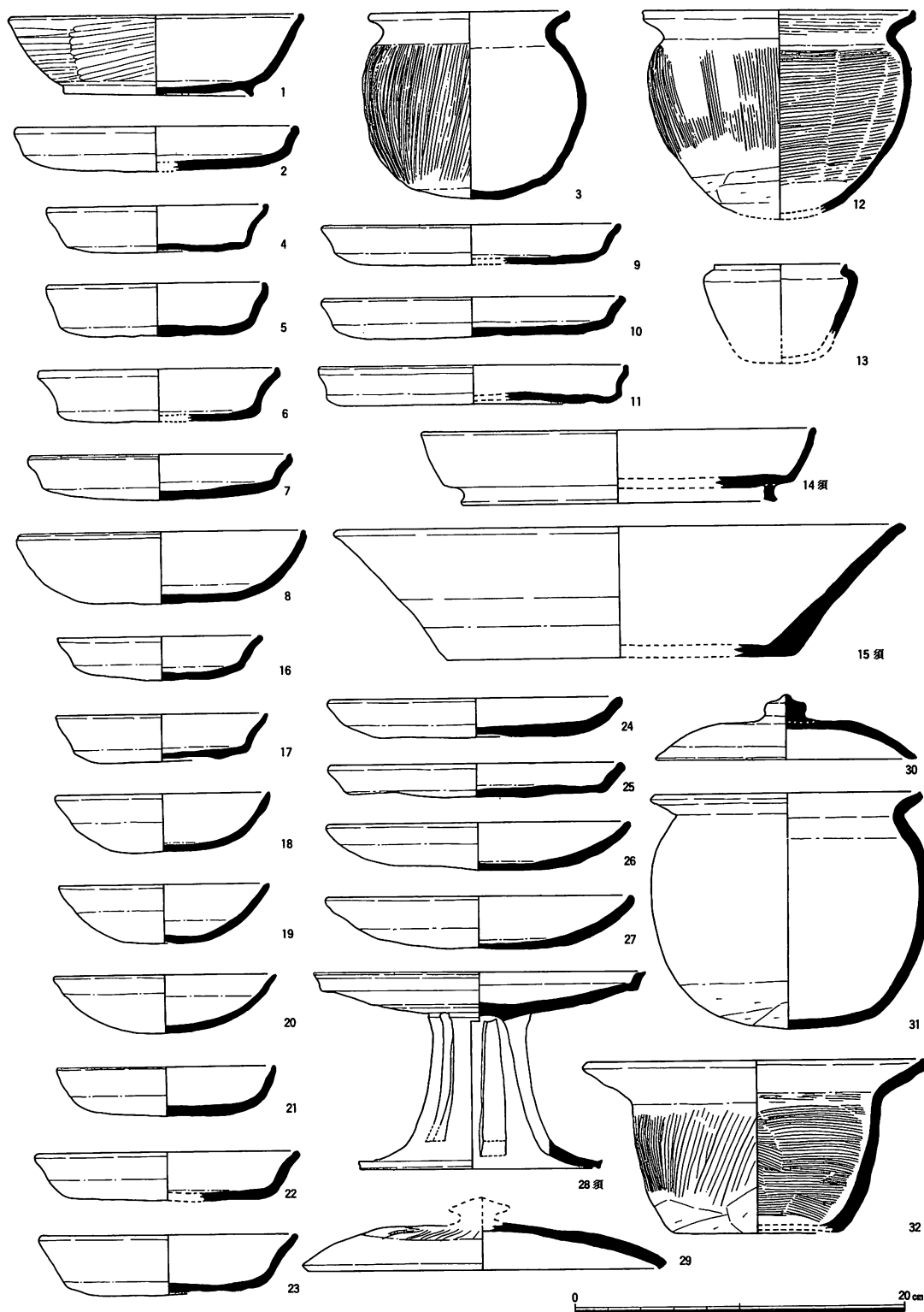
第18図 第92次調査 出土遺物実測図 SD2400 : 1 ~ 3、SK6510 : 4 ~ 15 SK6524 : 16 ~ 32 ( 1 : 4 )
