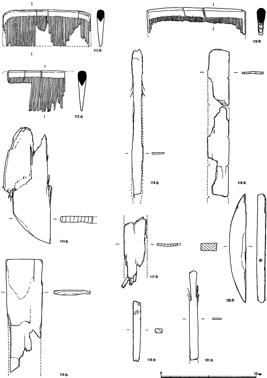
第 8 図 第90次調査 出土遺物実測図 SE6410 : 111~121 ( 1 : 2 )
