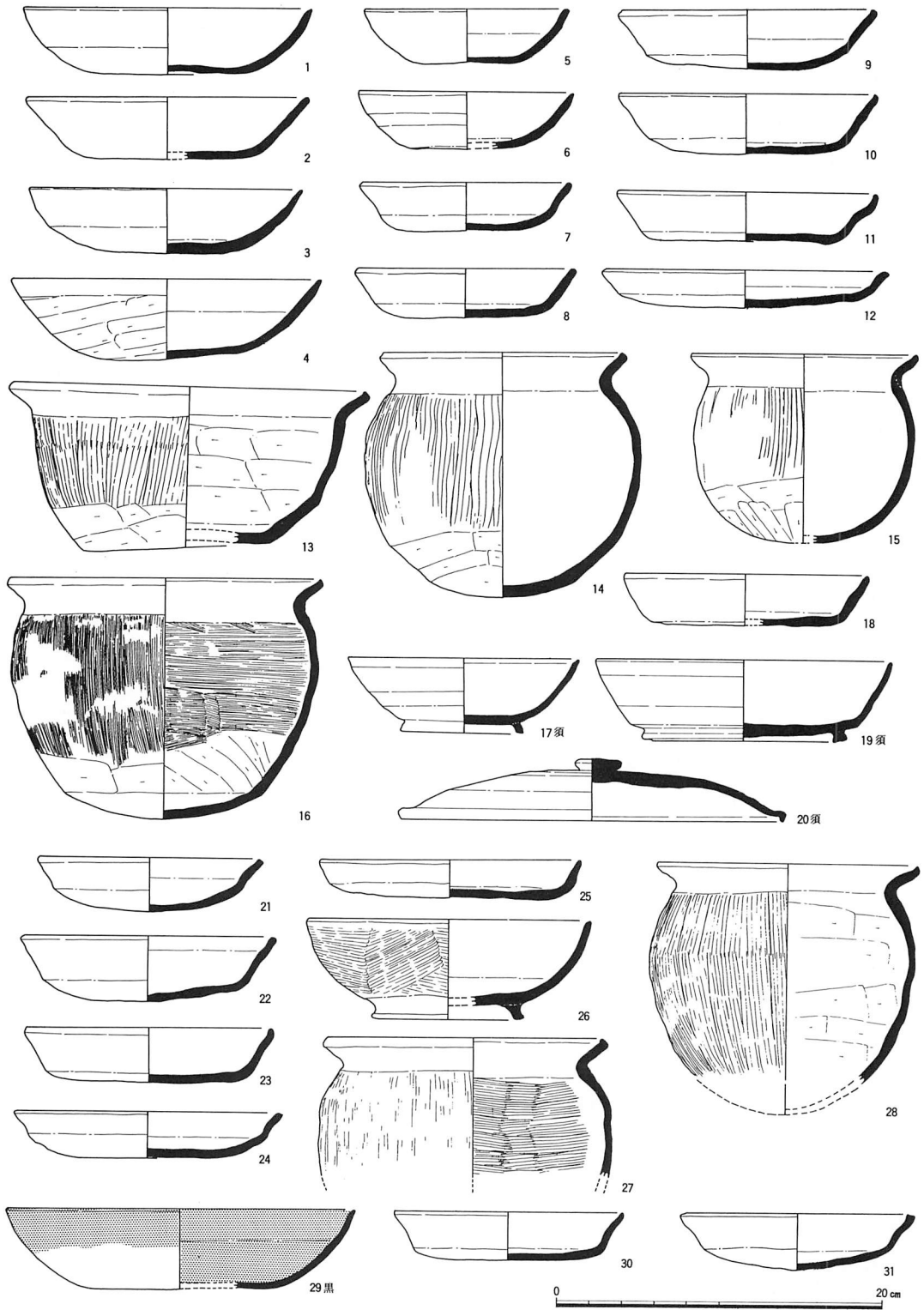
第23図 第93次調査 出土遺物実測図 SK6549 : 1~20、SK6552 : 21~28、SK6551 : 29~31 (1 : 4)
