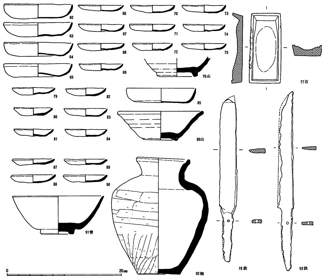
第25図 第93次調査 出土遺物実測図 S X 6533 : 62~78、S X 6534 : 79~86、S X 6537 : 87~93 (1 : 4)
