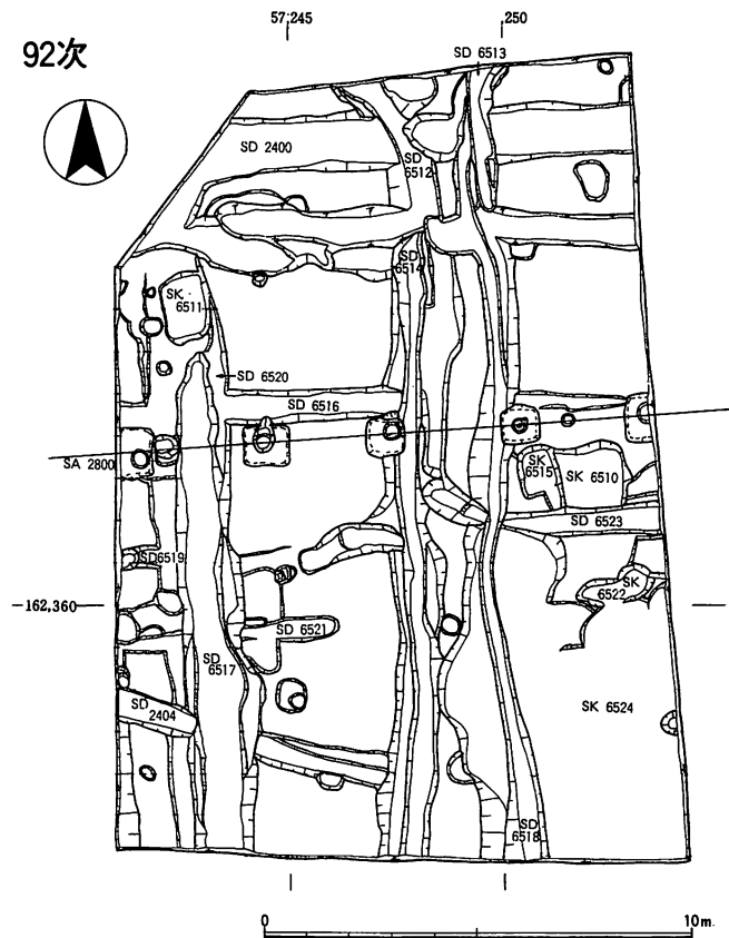
第16図 第92次調査 遺構実測図(1:200)
