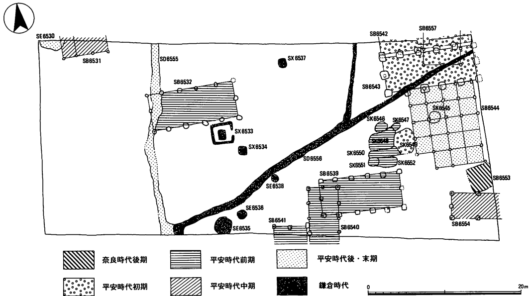
第21図 第93次調査 時期別遺構配置図 (1 : 500)
