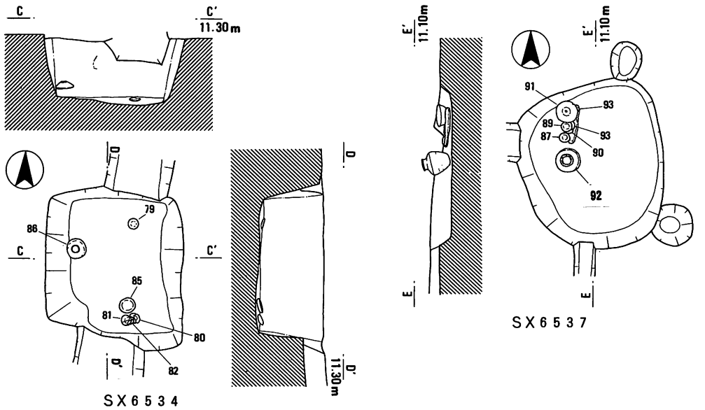
第22図 第93次調査 中世墓実測図 (1:40)
