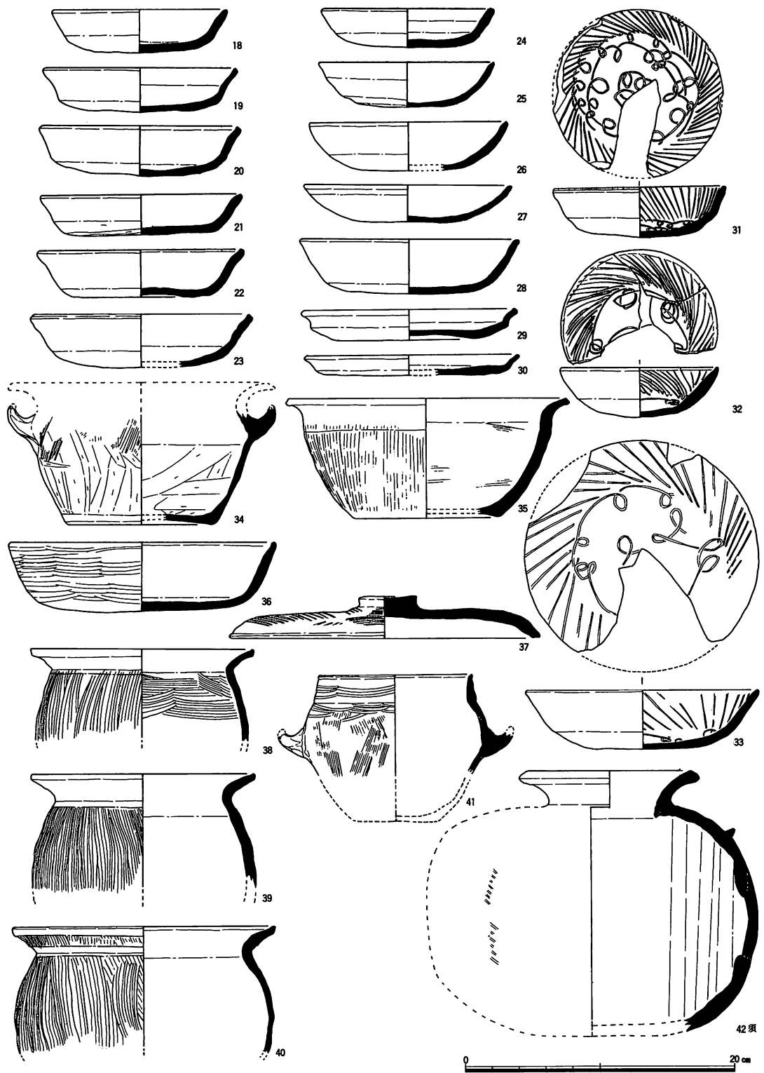
第4図 第90次調査 出土遺物実測図 SK6424:18~35、SK6425:36~42 (1:4)
