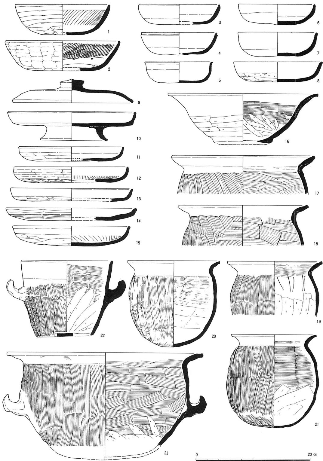
第14図 第91次調査 出土遺物実測図 SE6480：1～23（1：4）
