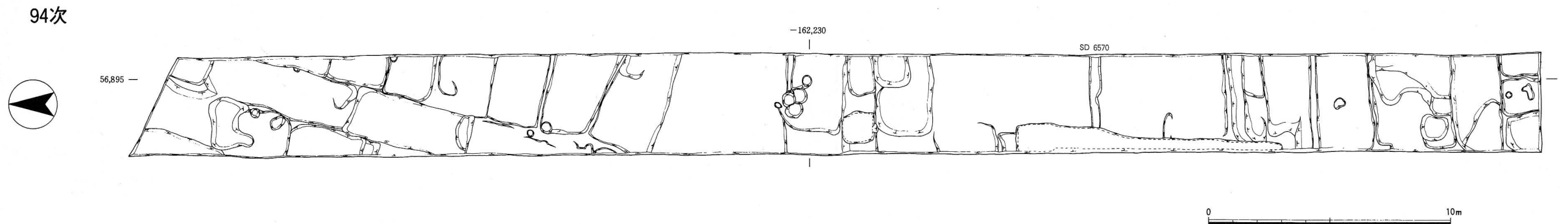
第27図 第94次調査 遺構実測図(1:200)
