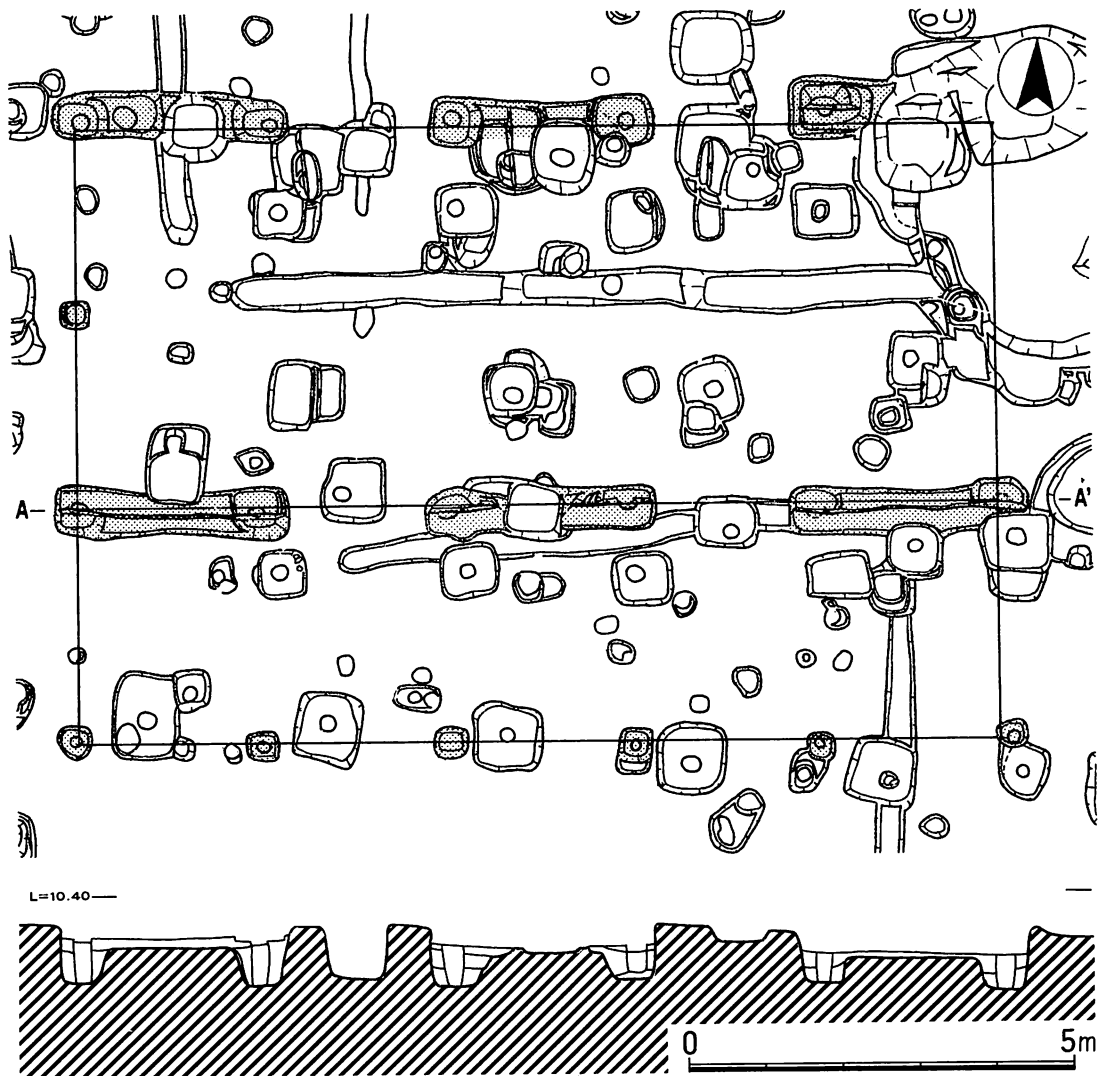
第6図 掘立柱建物S B 5800遺構平面図 (1:100)
