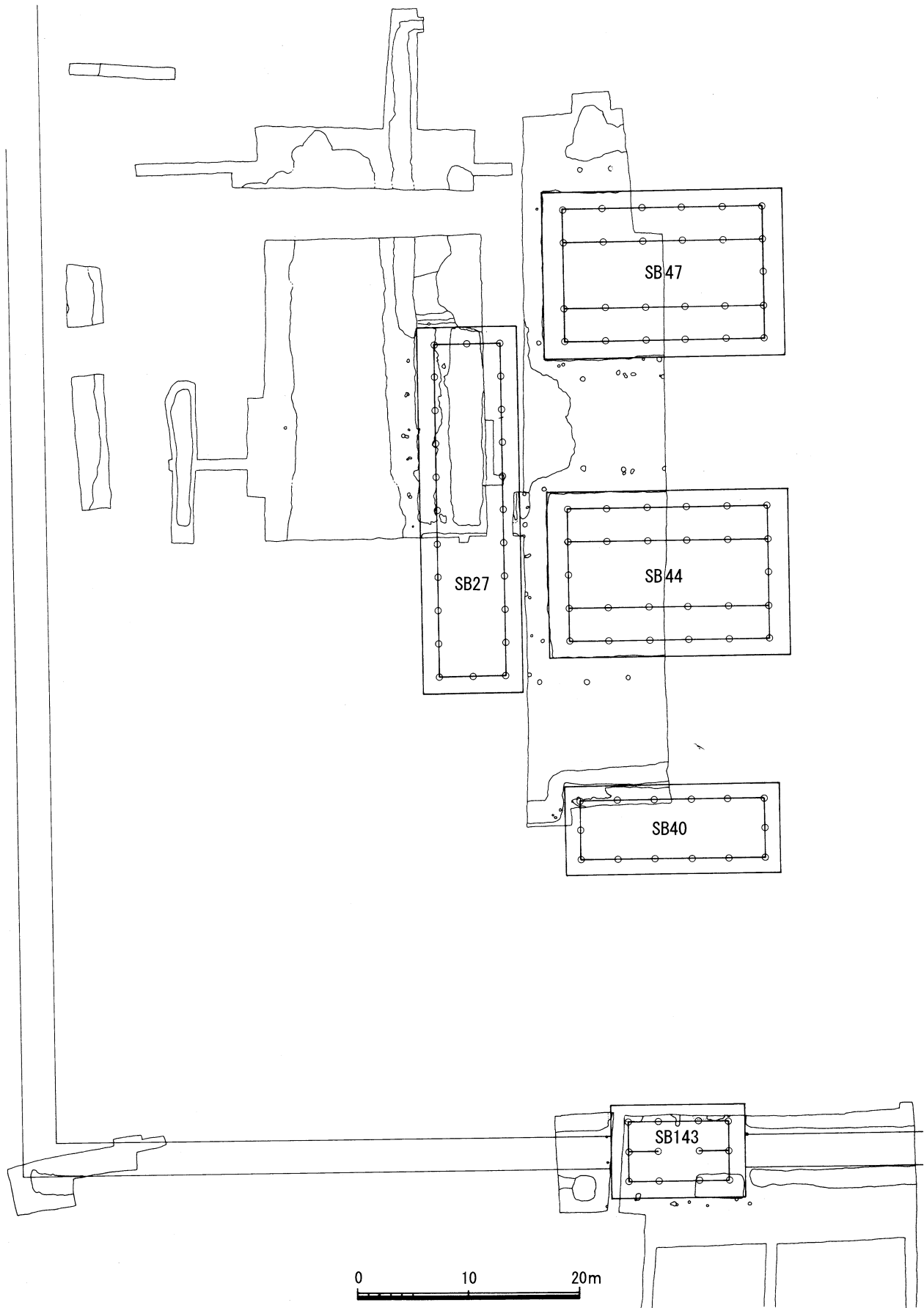
Fig. 1 長塚地区建物配置図案(1:500)
