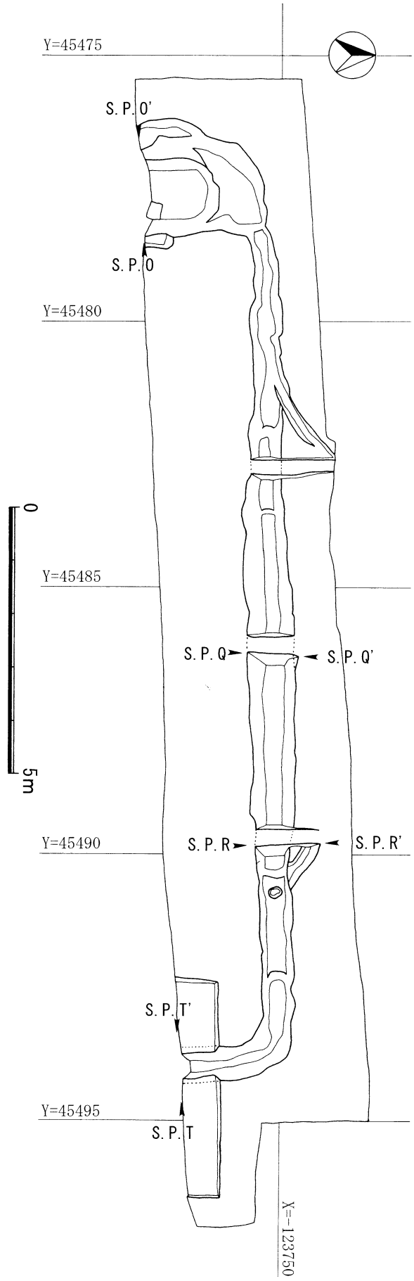
6AEB-A区平面図(1:100) 東溝, 西溝, 北溝断面図(1:50)
