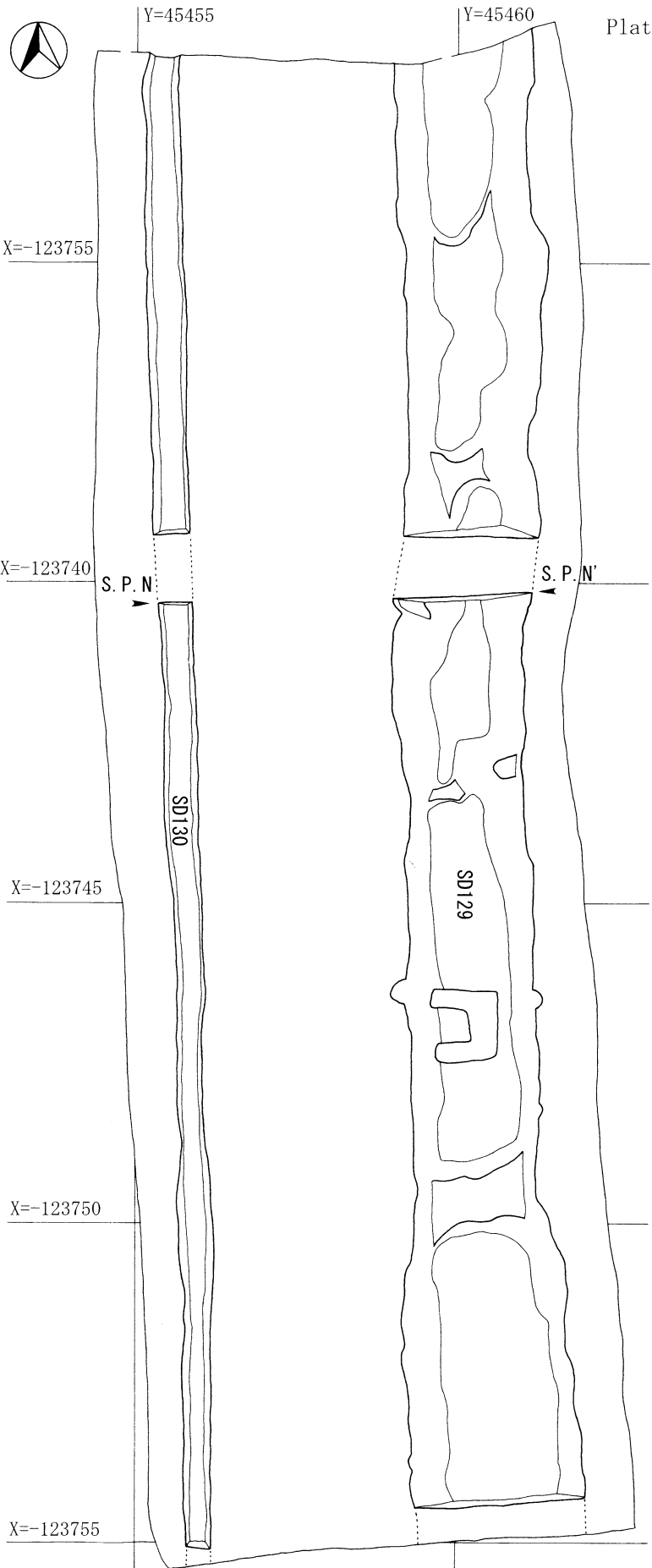
6AEB-B区平面図(1:100) 溝SD129-SD130断面図(1:50)
