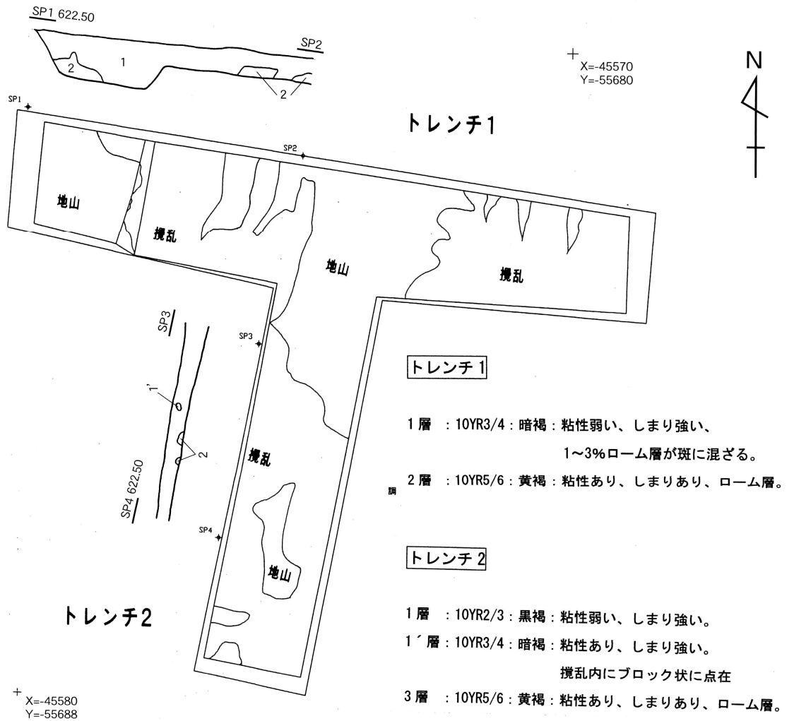
図8 増野新切Ⅱ遺跡調査図及び土層断面図(1:80)
