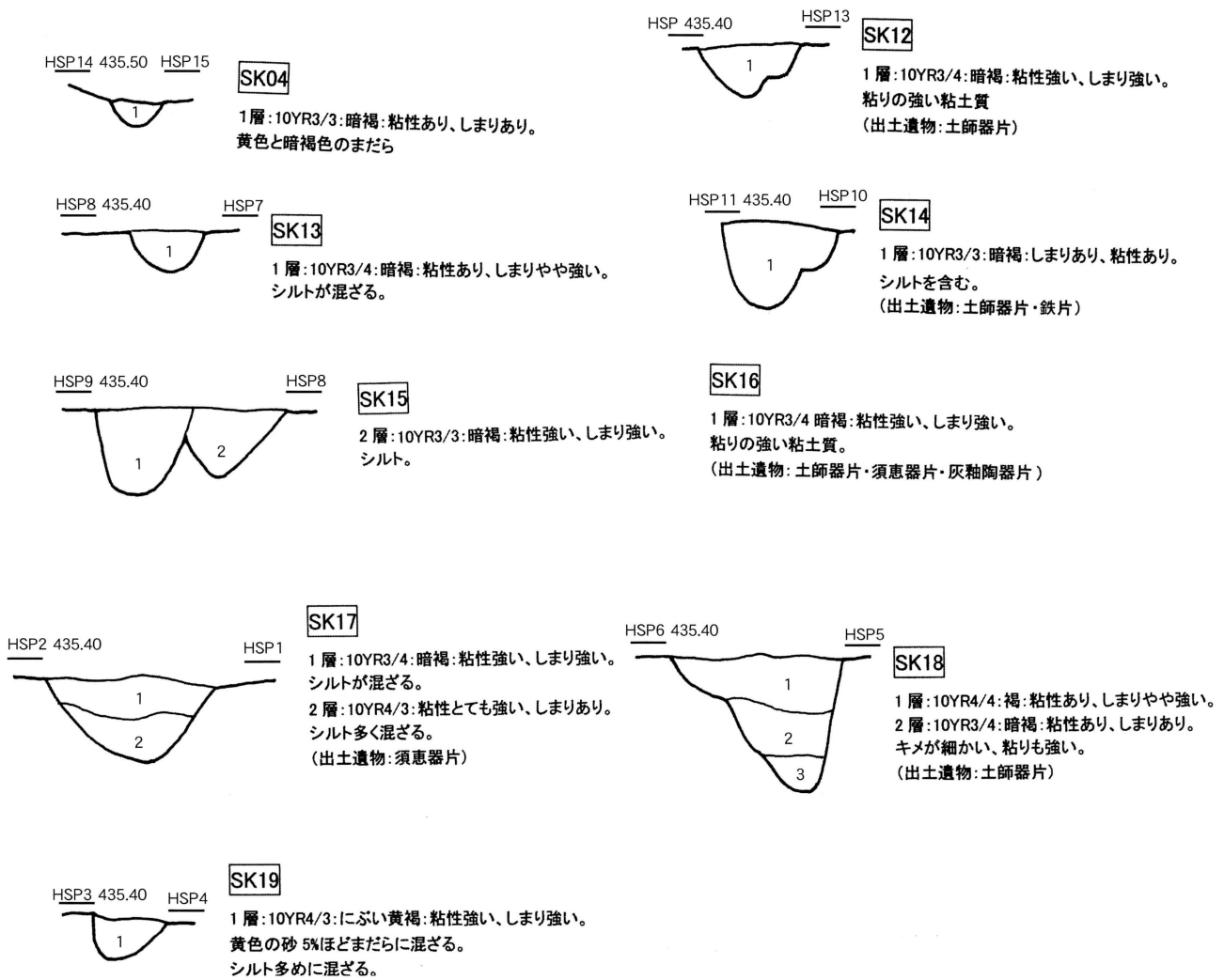
図34 堂垣外遺跡土坑半裁図(1:20)
