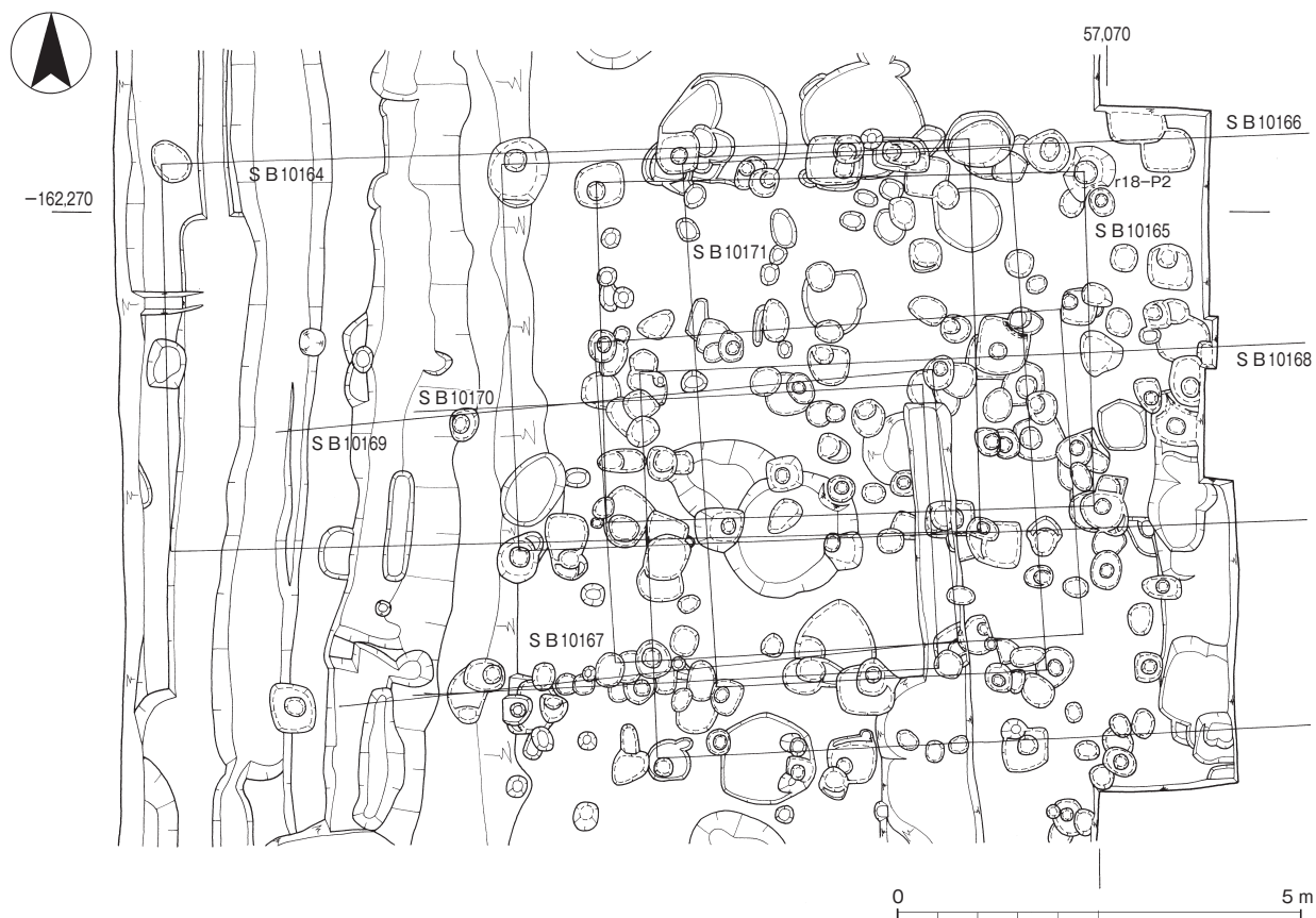
第Ⅱ-5図 第167次調査 SB10164～10171平面図(1:100)
