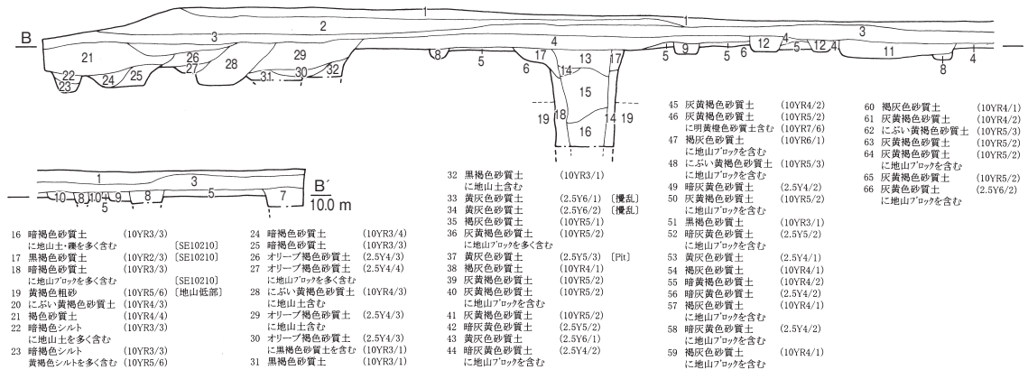
第Ⅱ-4図 第167次調査 土層断面図 (1:100)
