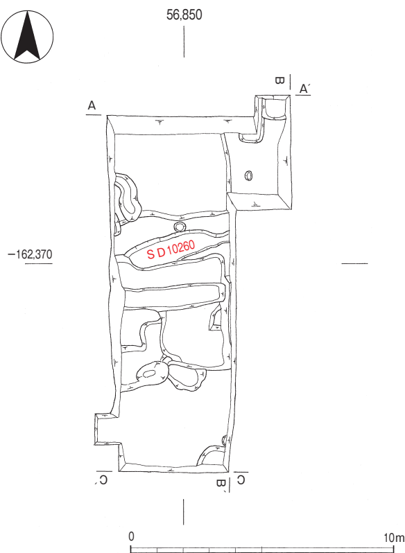
第IV-2図 第169次調査 遺構平面図 (1 : 200)
