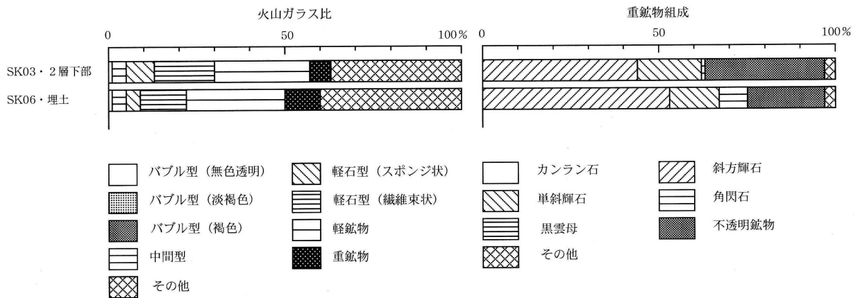
図1 テフラ組成ダイアグラム
