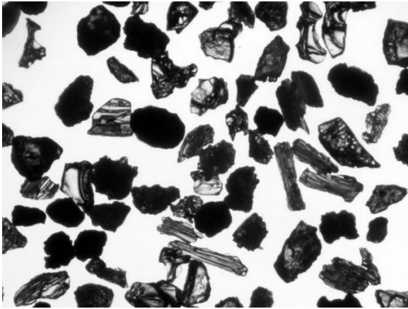
写真1 SK03・2層下部テフラ分析試料の顕微鏡写真(透過光)
