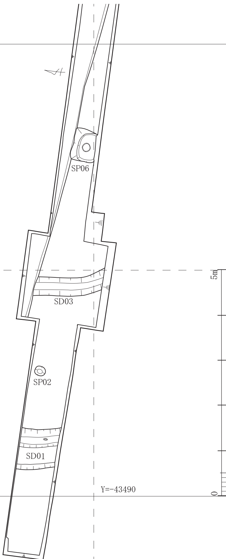
第10图 8区・9区遺構平面図 (S=1/50)
