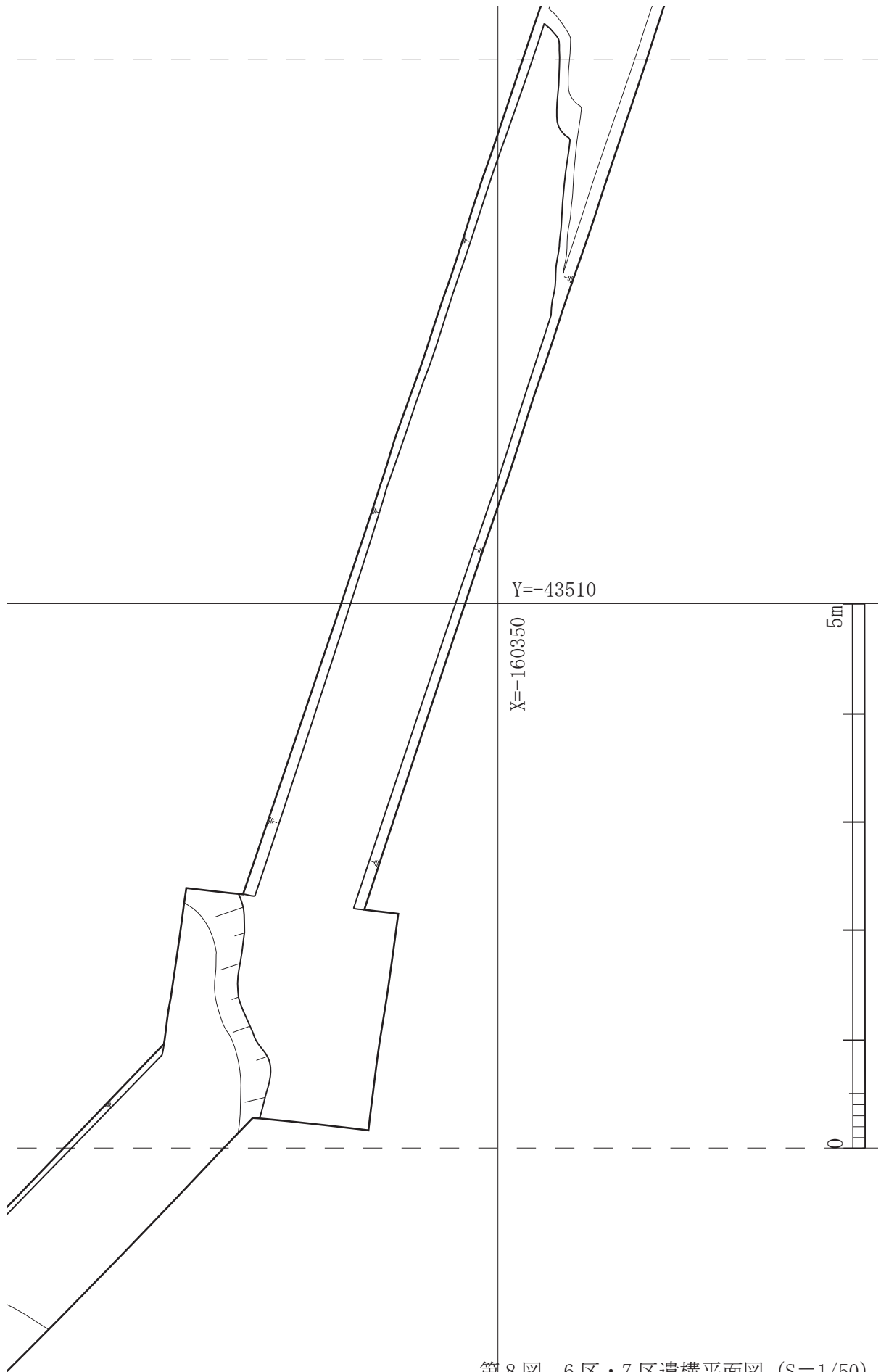
第8图 6区・7区遺構平面図 (S=1/50)
