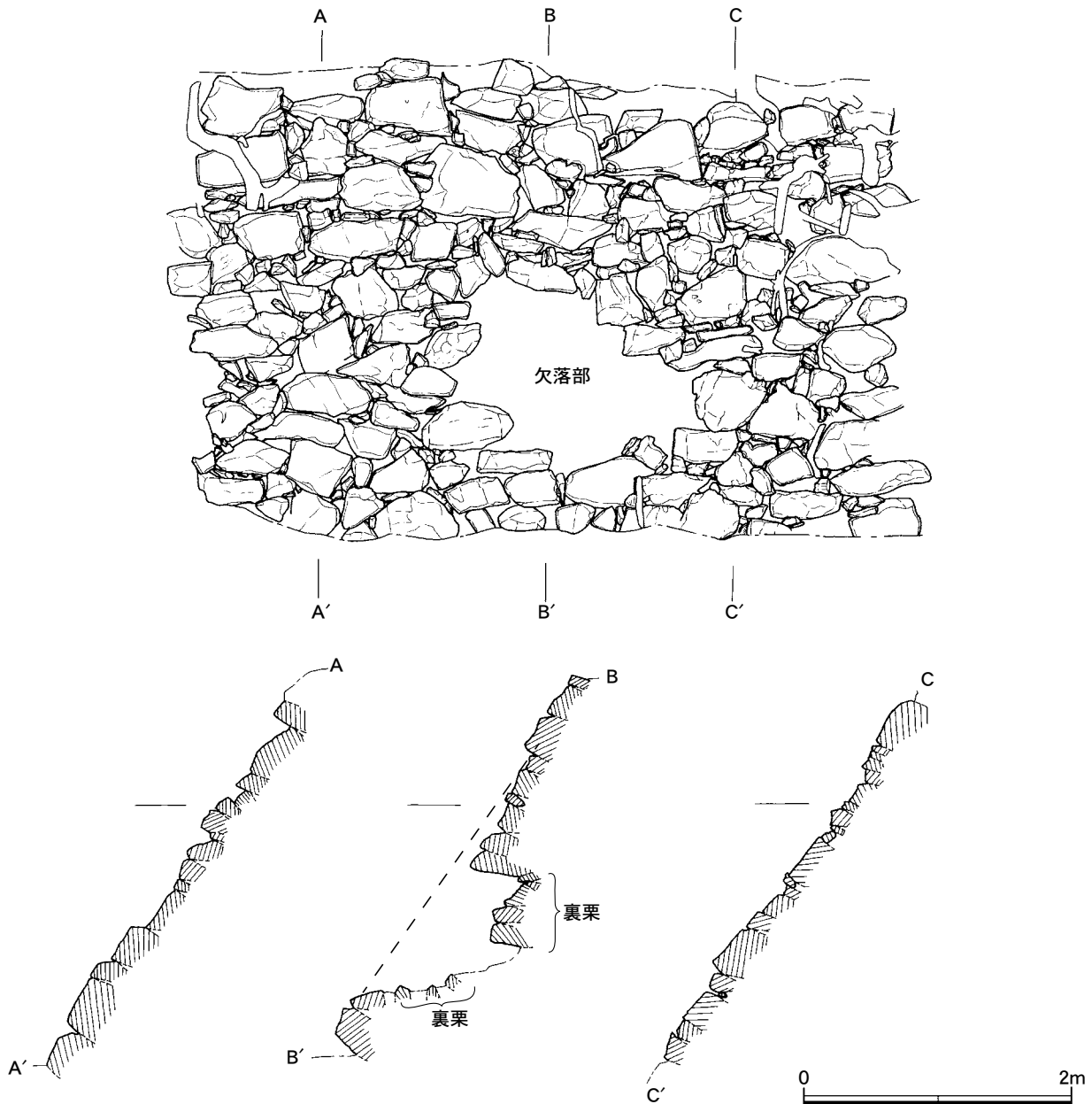
第7図 9面築石欠落部1 (S=1/50)
