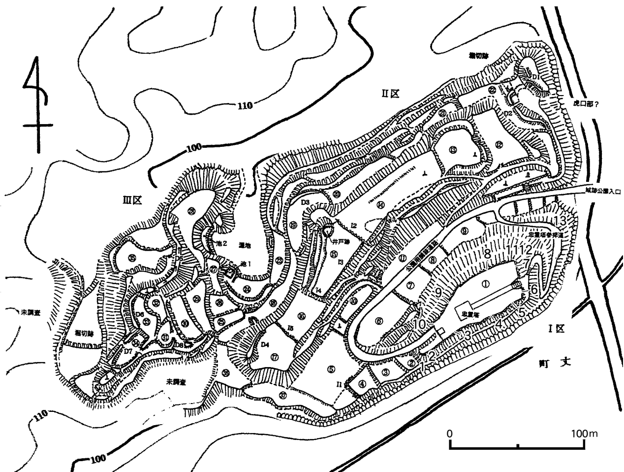
第6図 平田城跡縄張り図 (S=1/2,700)
