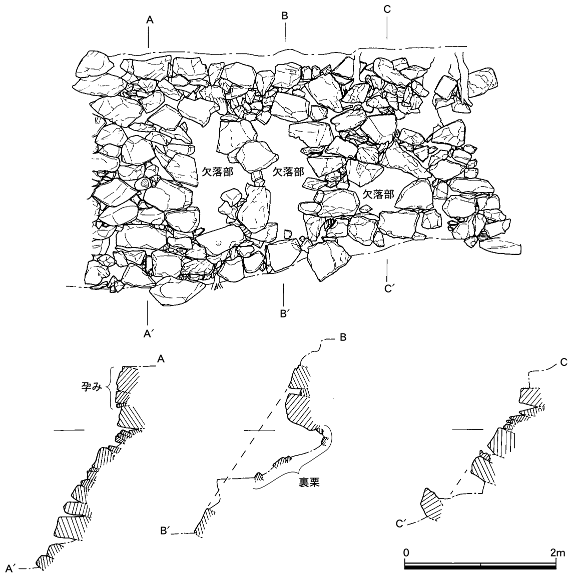
第8図 9面築石欠落部2 (S=1/50)
